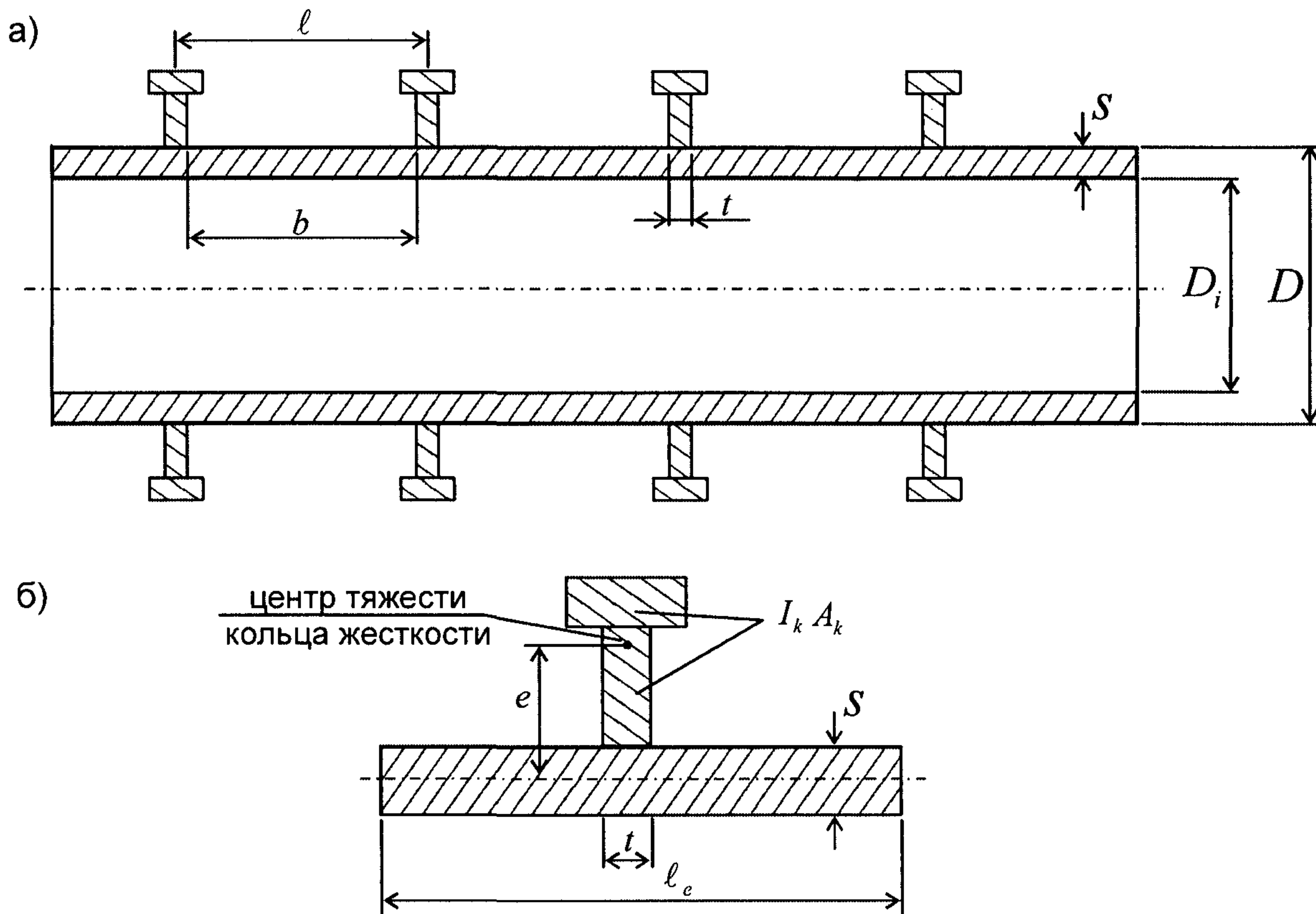
Рис. 5.3. Труба, подкрепленная кольцами жесткости
