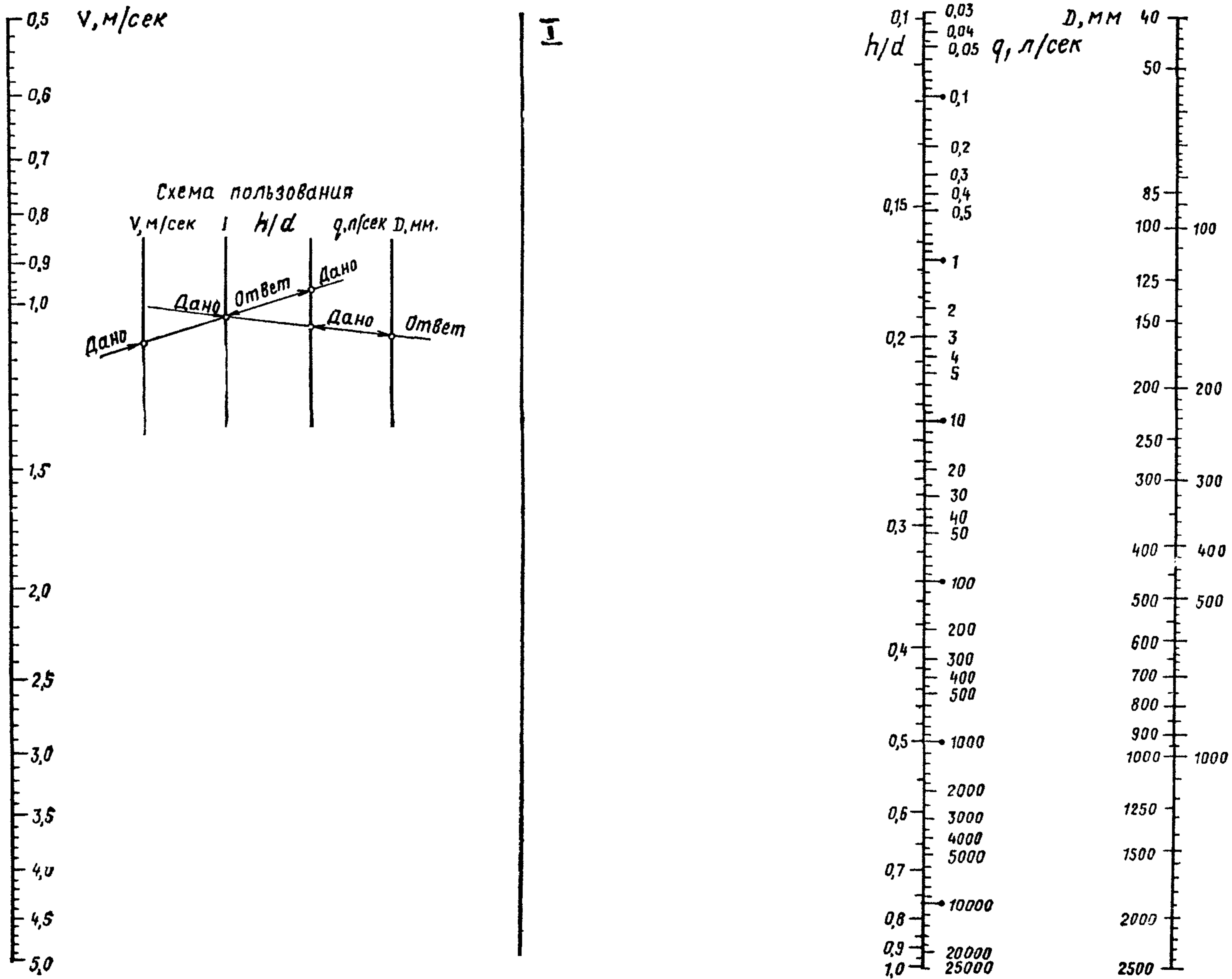
Рис. 2. Номограмма для определения диаметров канализационных трубопроводов
