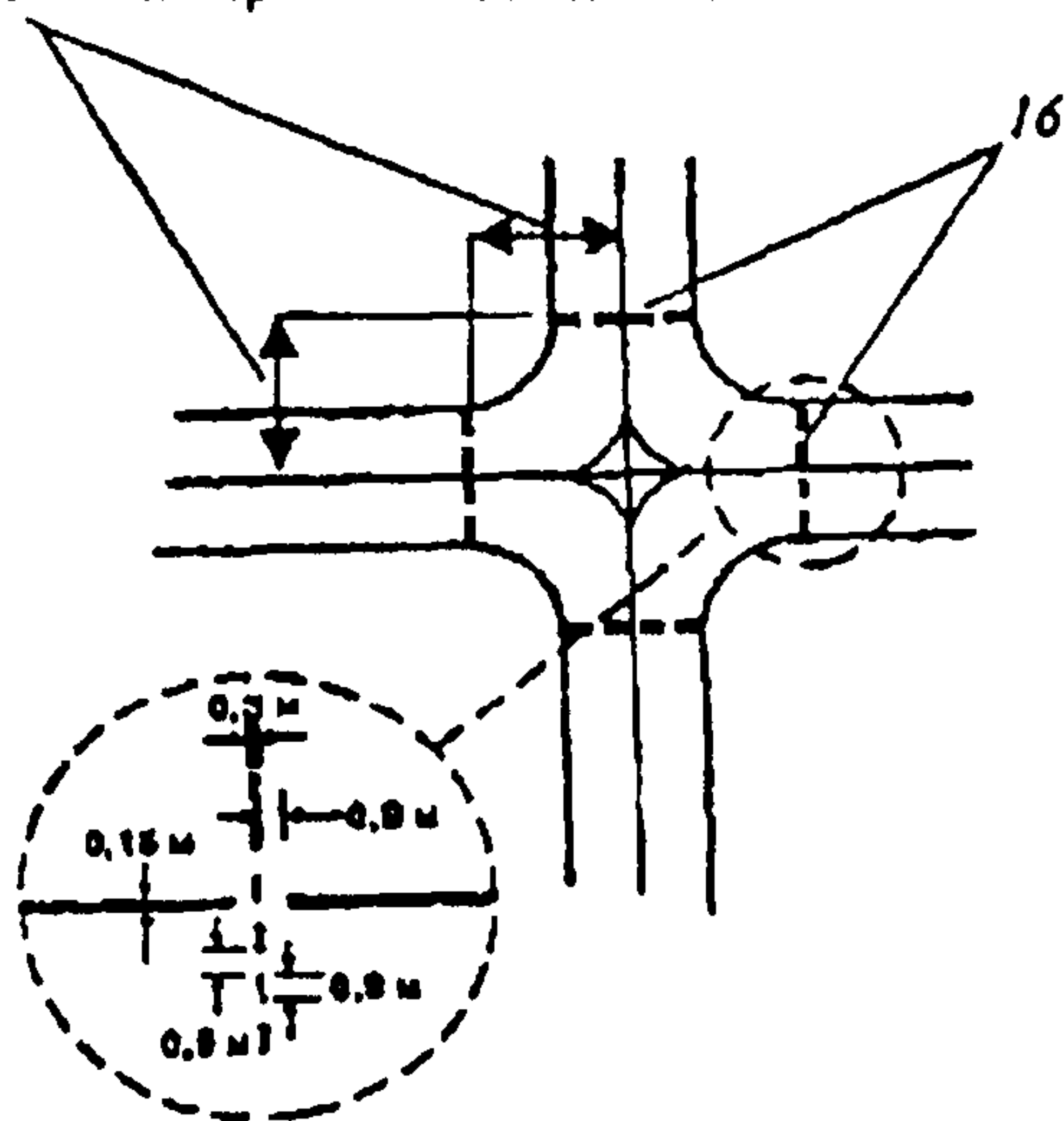
Рис. 4.6. Схема маркировки аэродрома:
