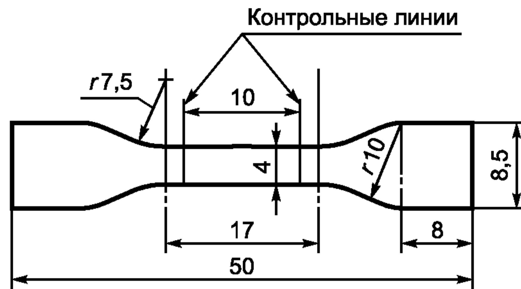
Рисунок 2 — Образец в виде двусторонней лопатки уменьшенного размера
