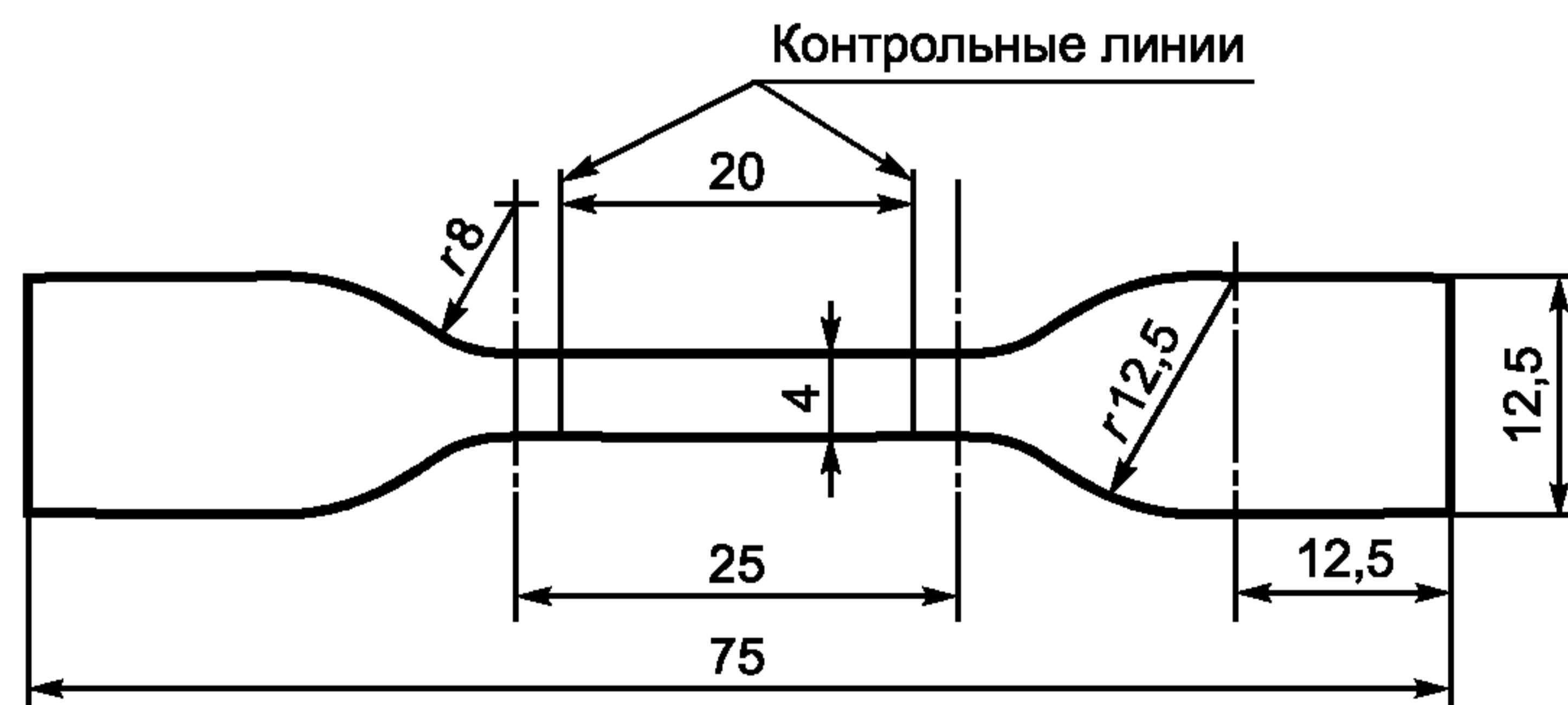
Рисунок 1 — Образец в виде двусторонней лопатки
