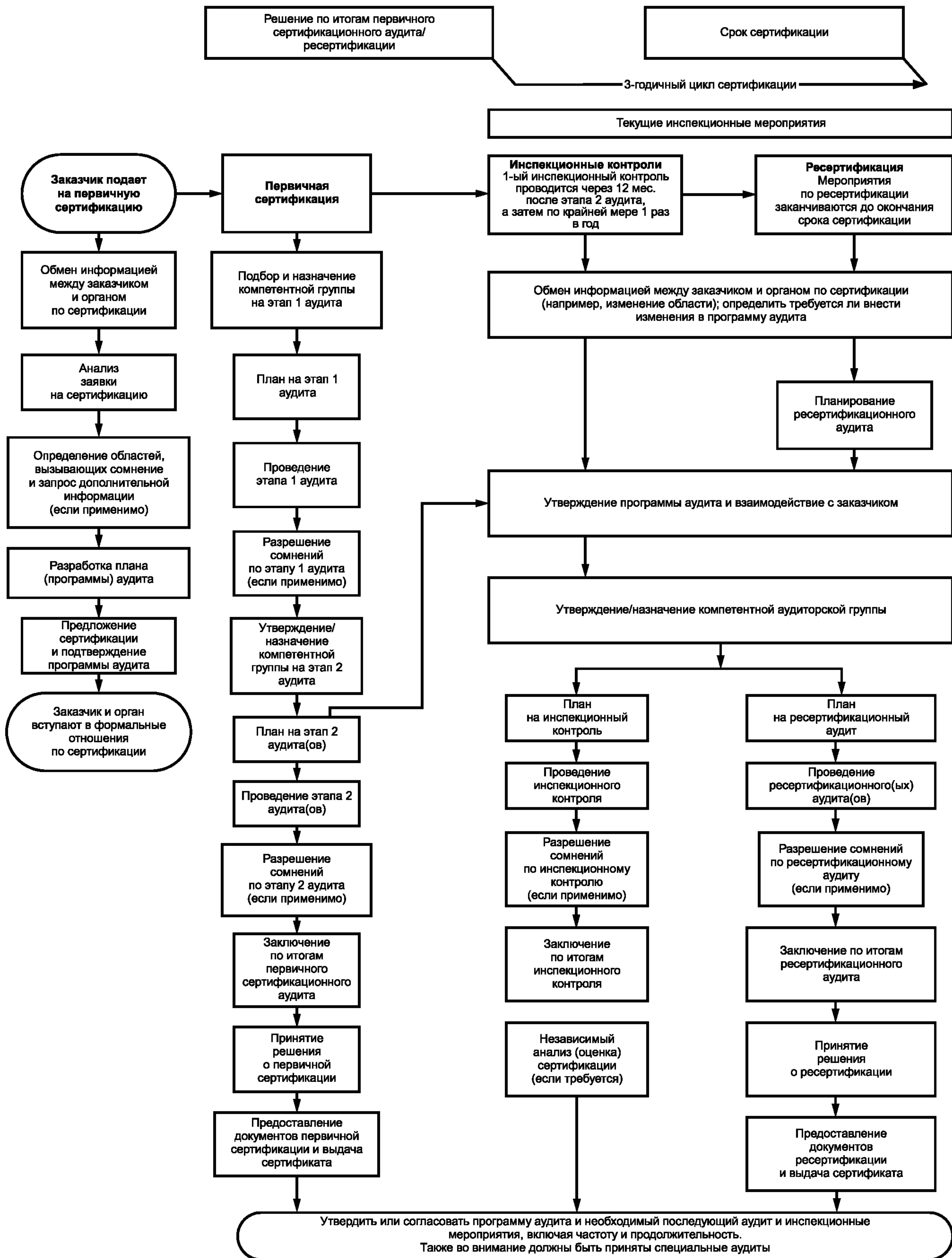
Рисунок Е.1 — Типичная блок-схема процесса аудита третьей стороной и сертификации
