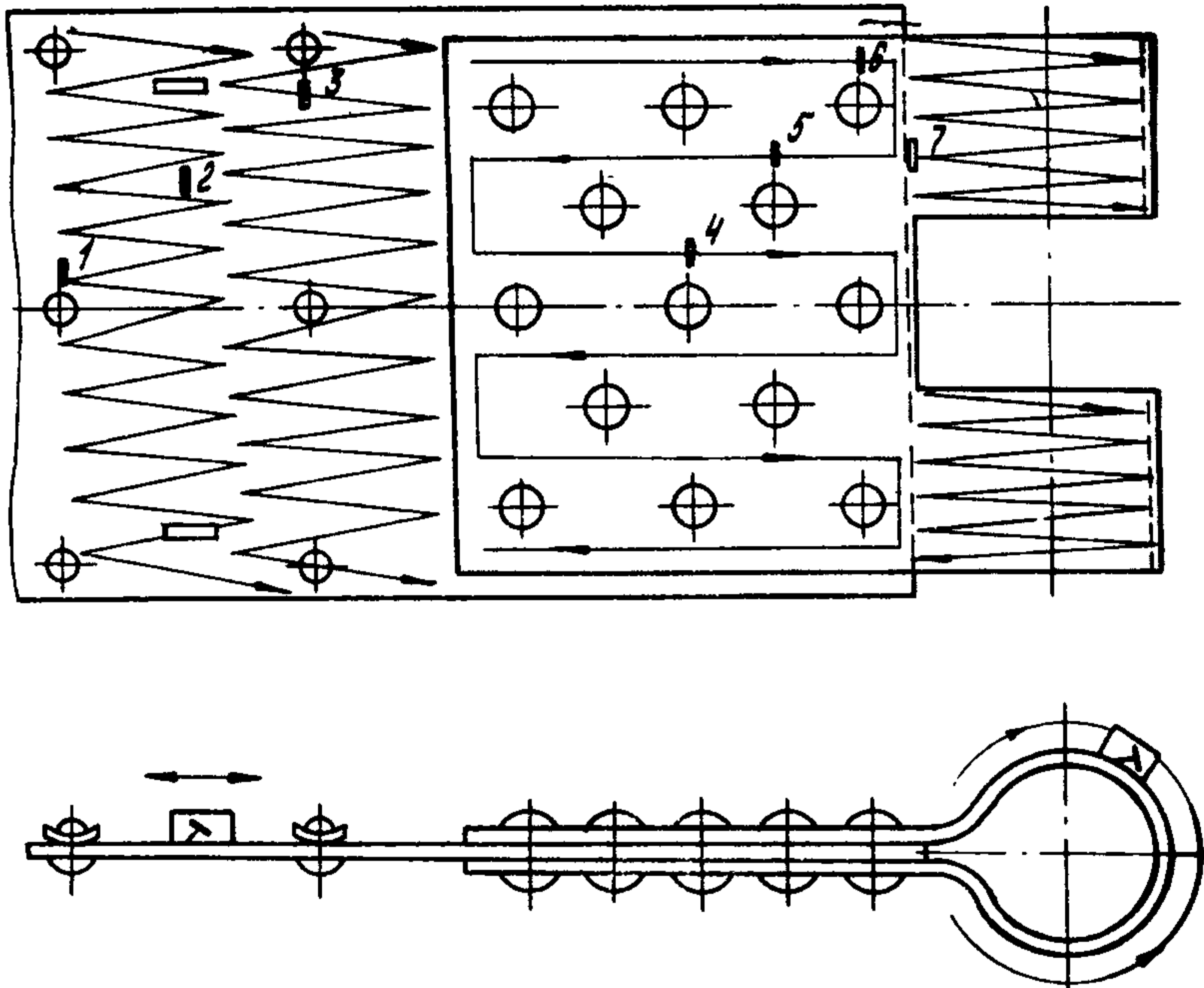
Рис. 2. Схема перемещения ультразвуковой искательной головки: 1-7 - искусственные дефекты
