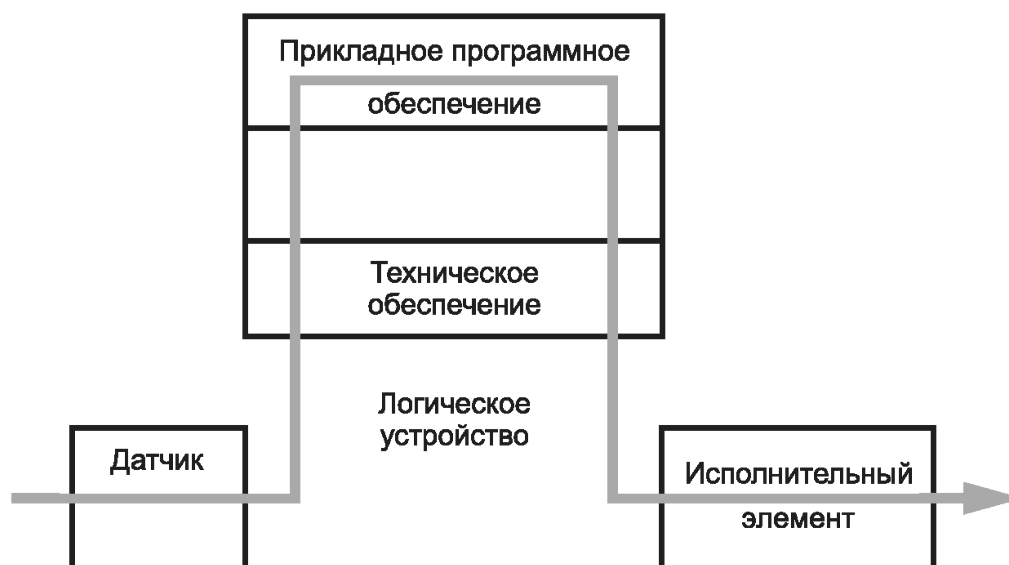
Рисунок С.1 — Логическое решающее устройство
