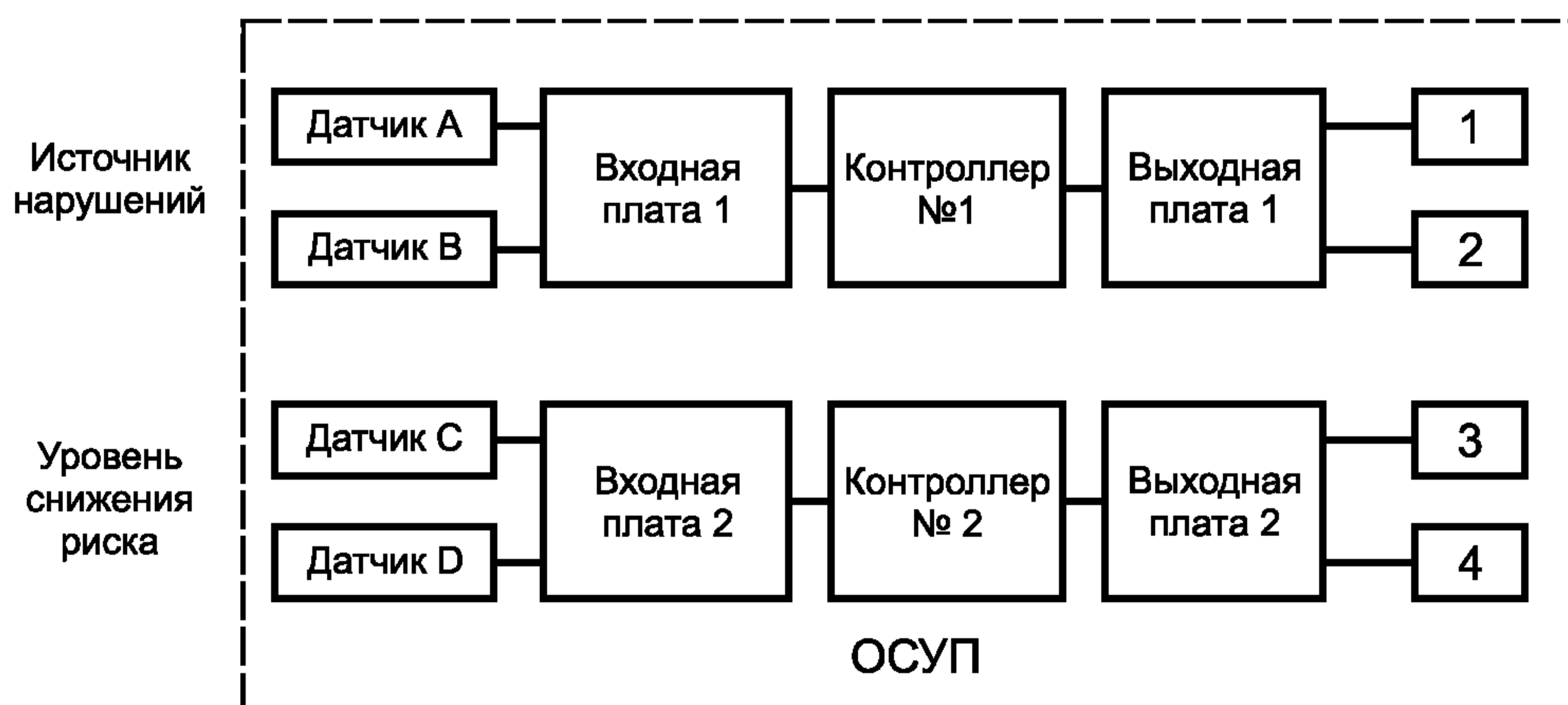
Рисунок 2 — Функция ОСУП и независимость источника нарушений
