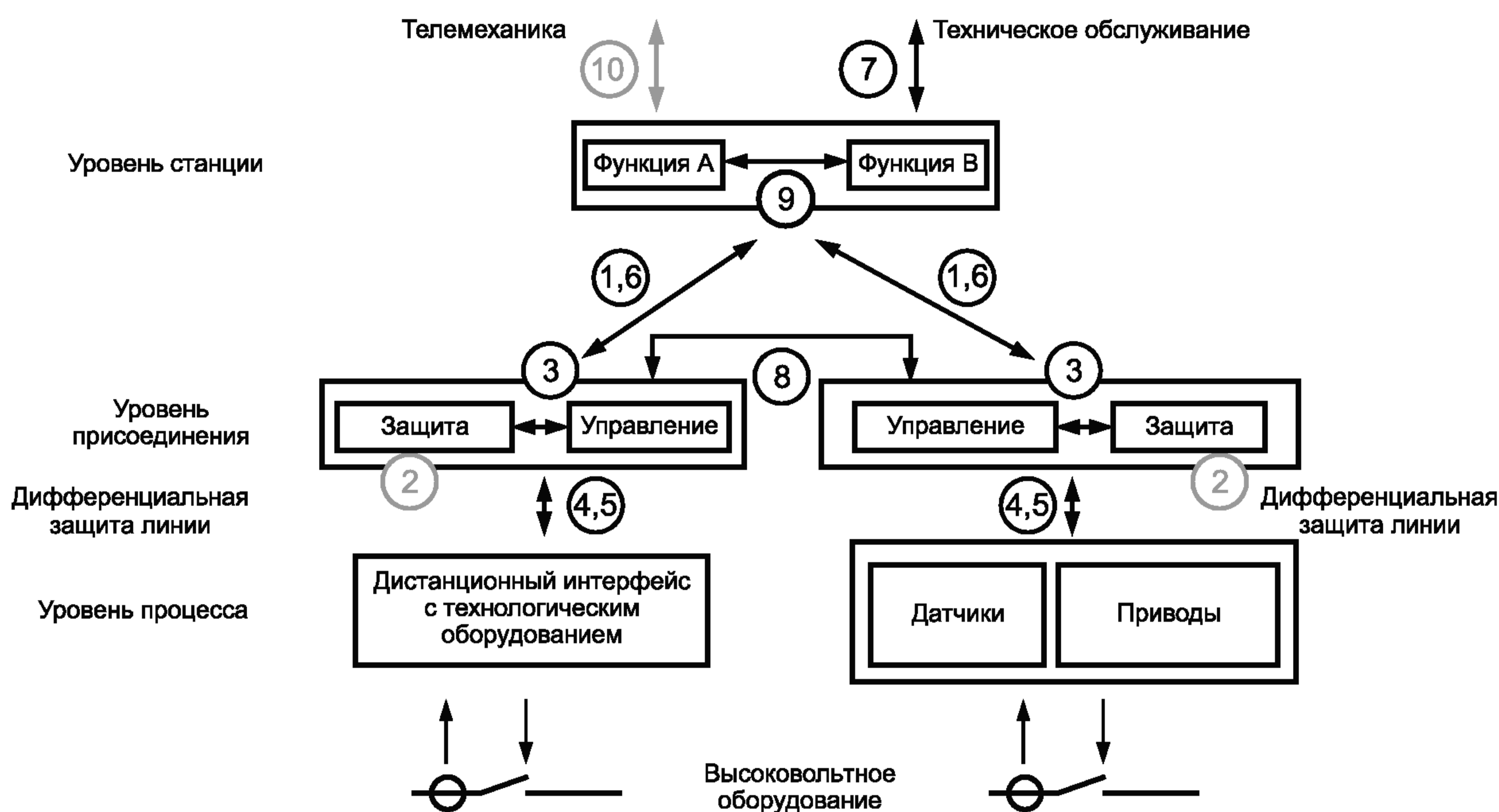
Рисунок ДА.1 — Модель интерфейсов системы автоматизации подстанции
