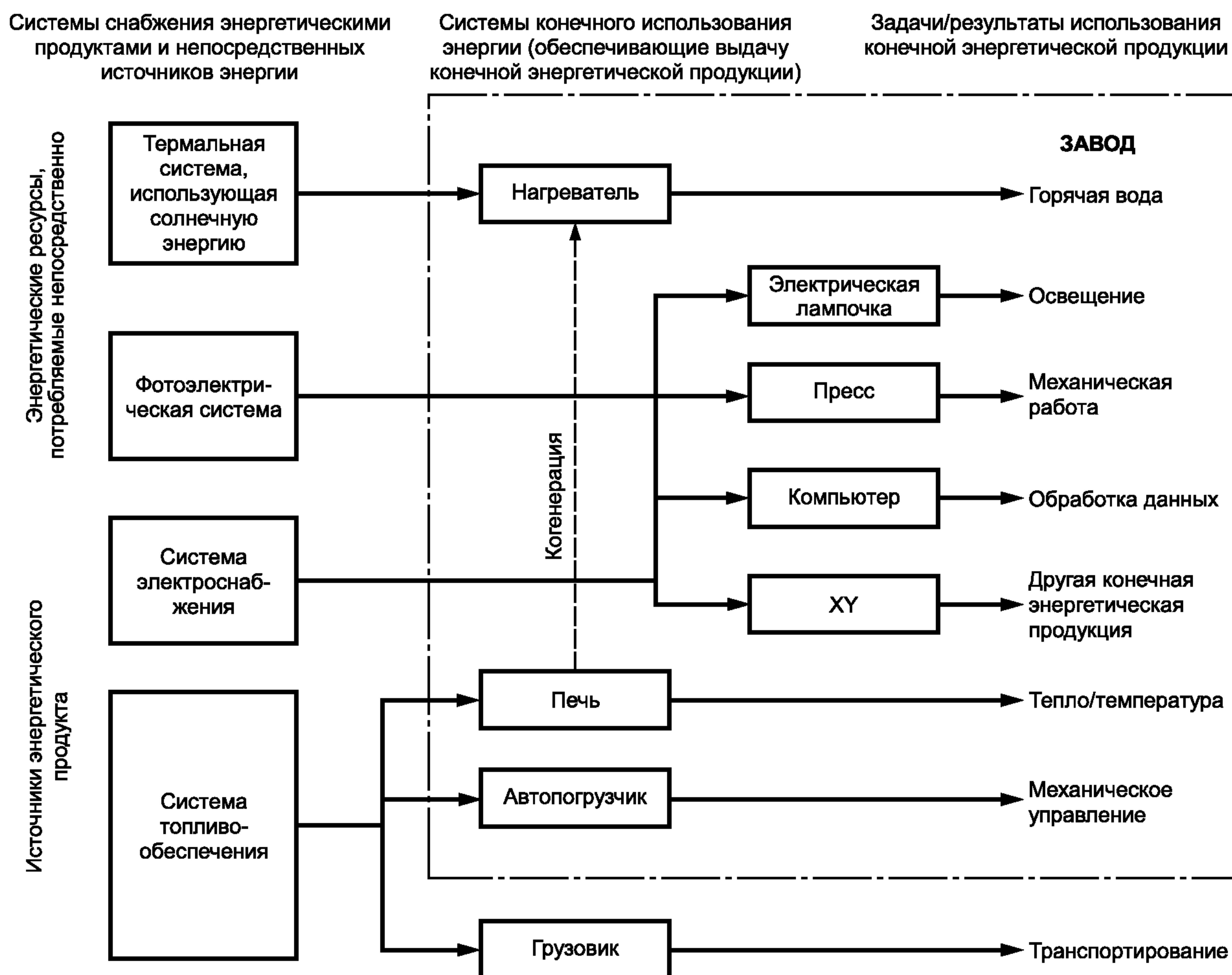
Рисунок 2 — Примеры возможной комбинации энергосистемы на предприятии
