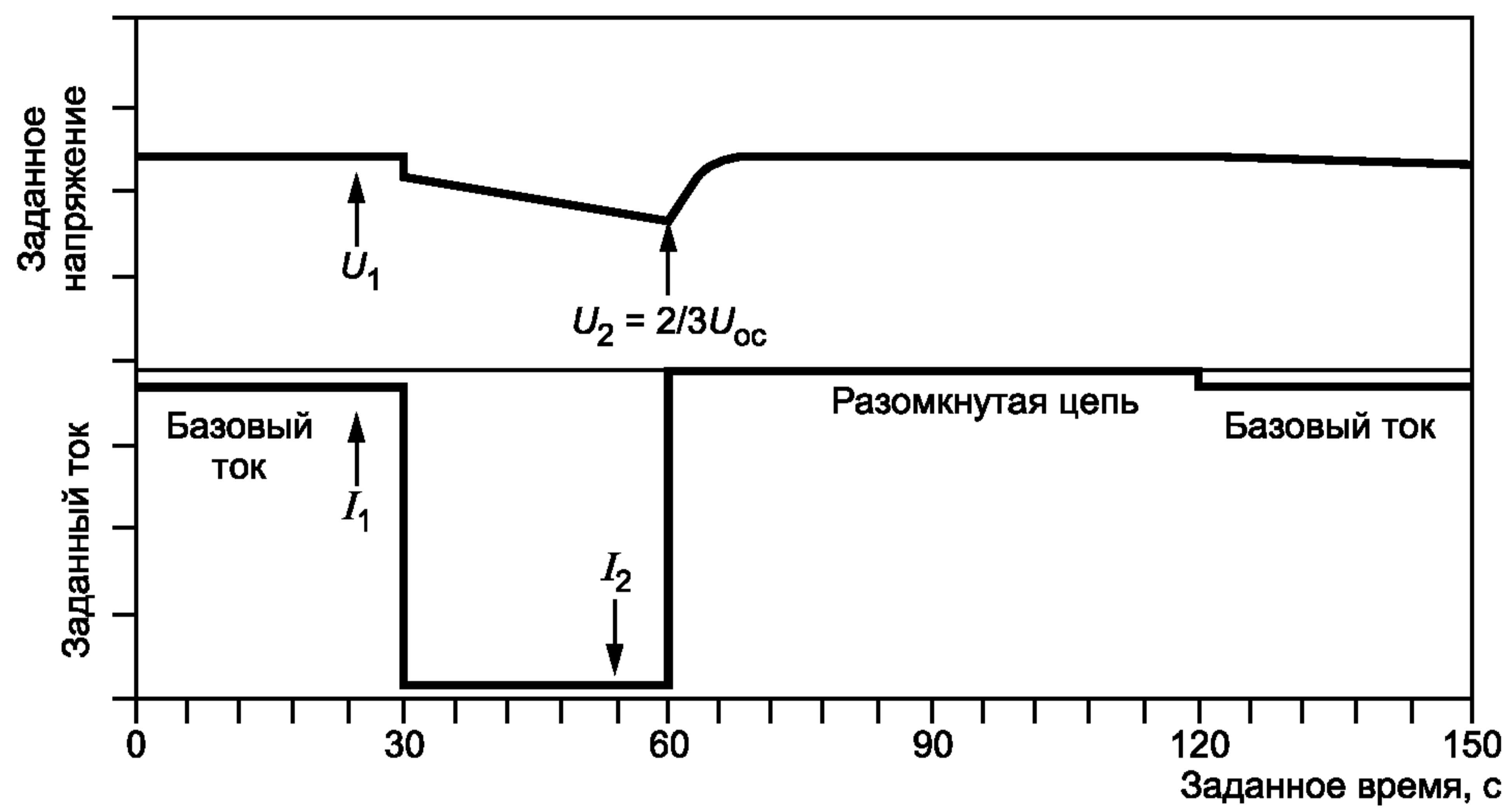
Рисунок 1 — Профиль испытания на пиковую мощность
