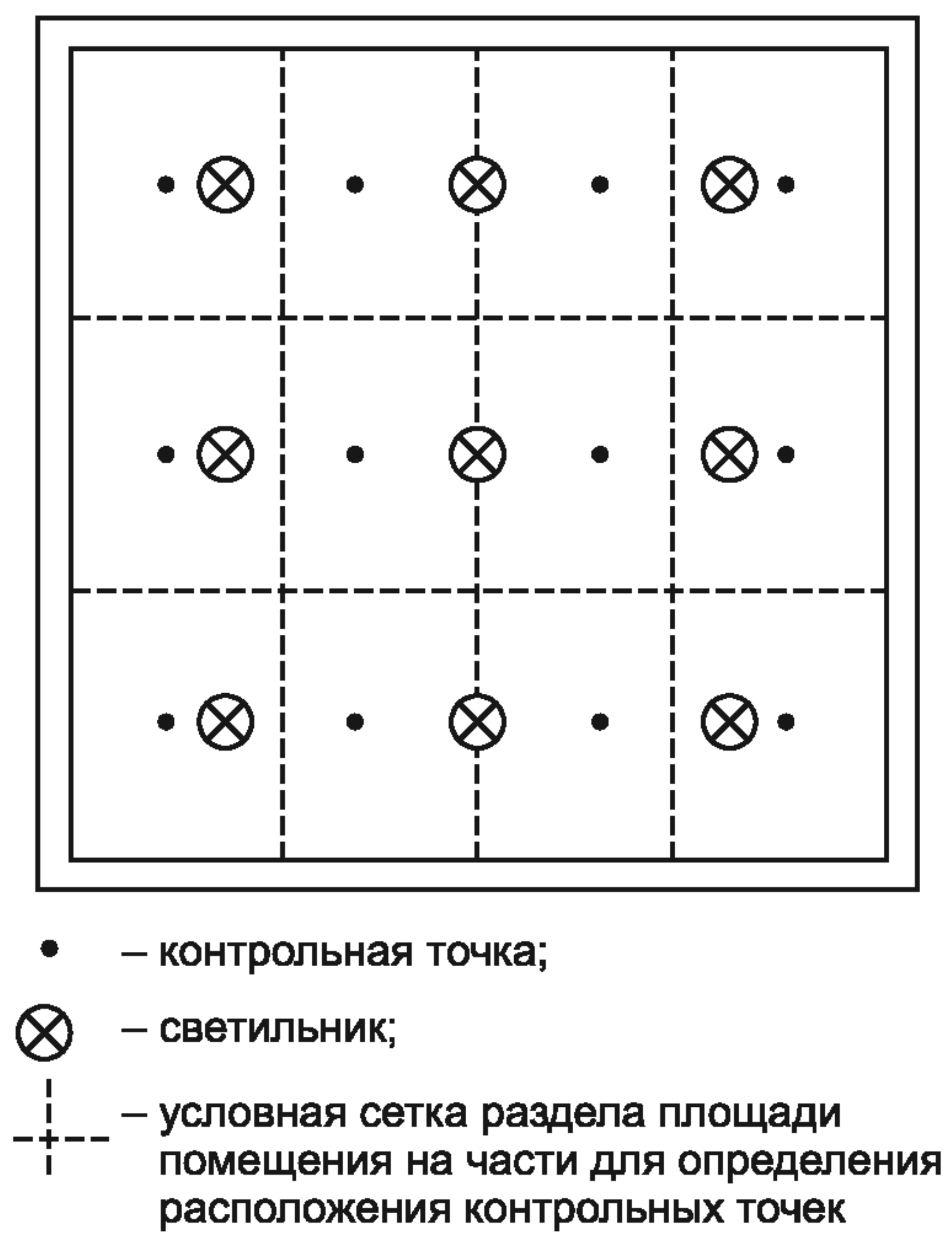
Рисунок В.1 — Расположение контрольных точек при измерении коэффициента пульсации освещенности в помещении
