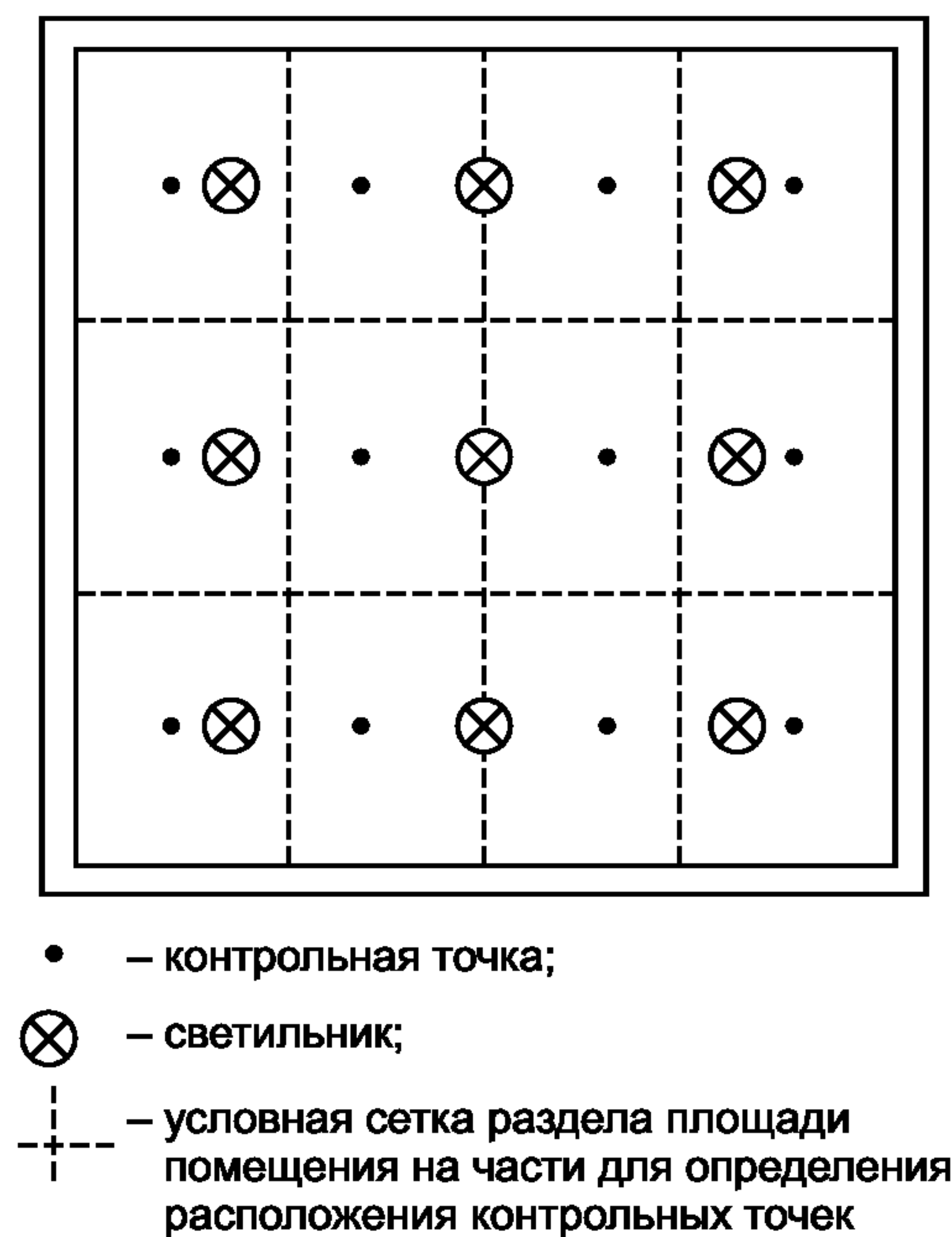
Рисунок А.3 — Расположение контрольных точек при измерении средней освещенности в помещении
