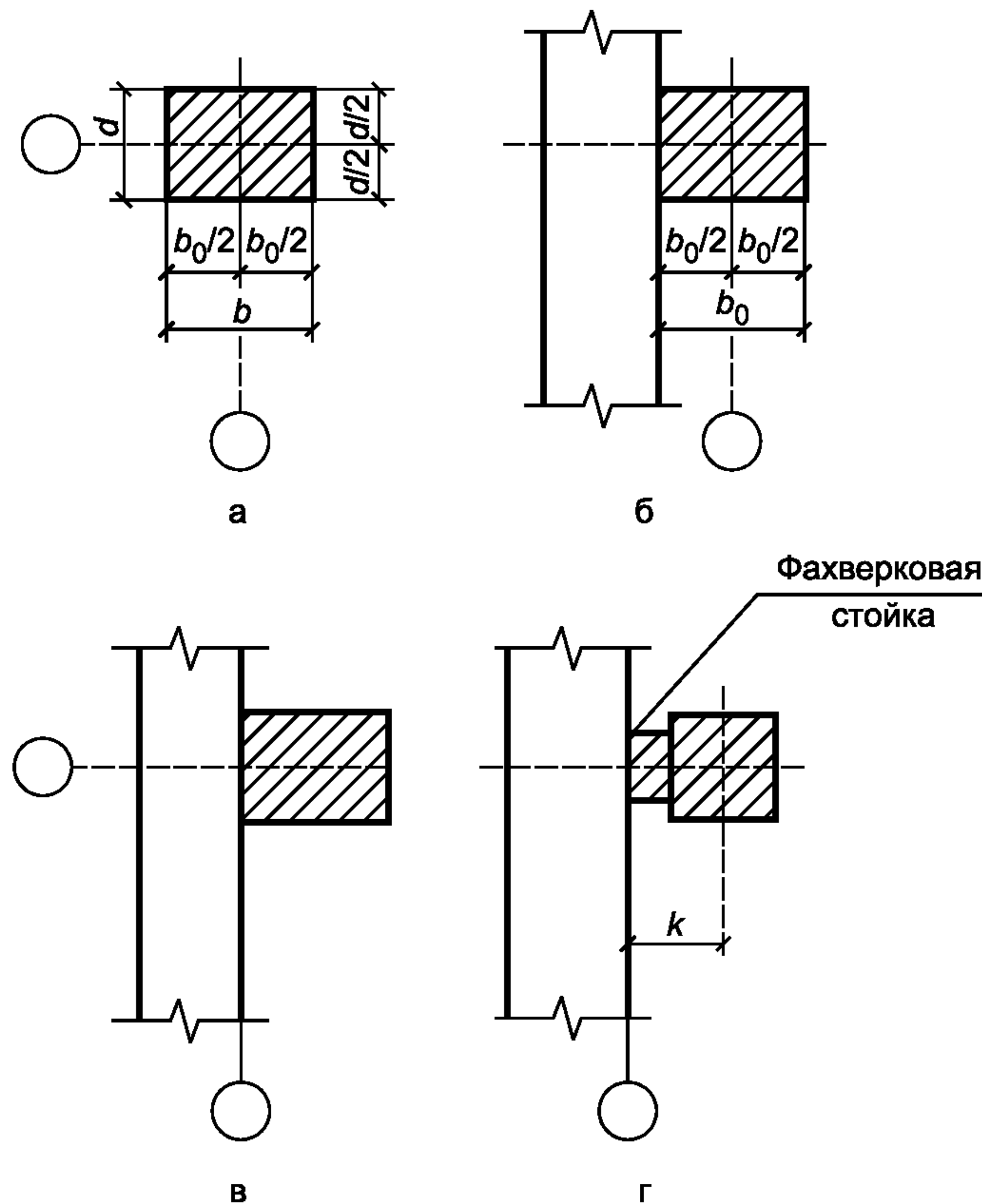
Рисунок 11 — Привязка колонн каркасных зданий к координационным осям
