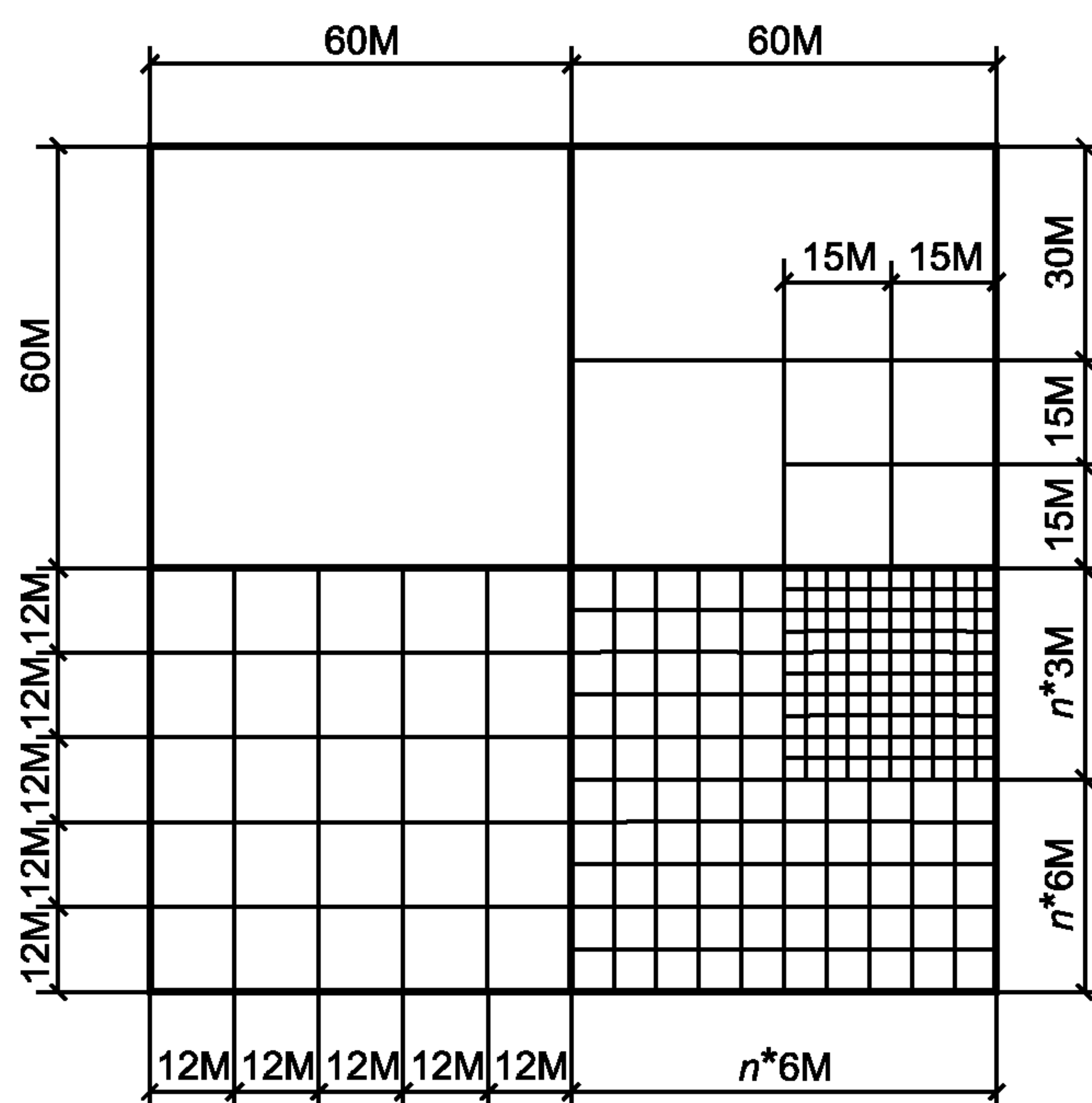
Рисунок 2 — Многомодульные сетки
