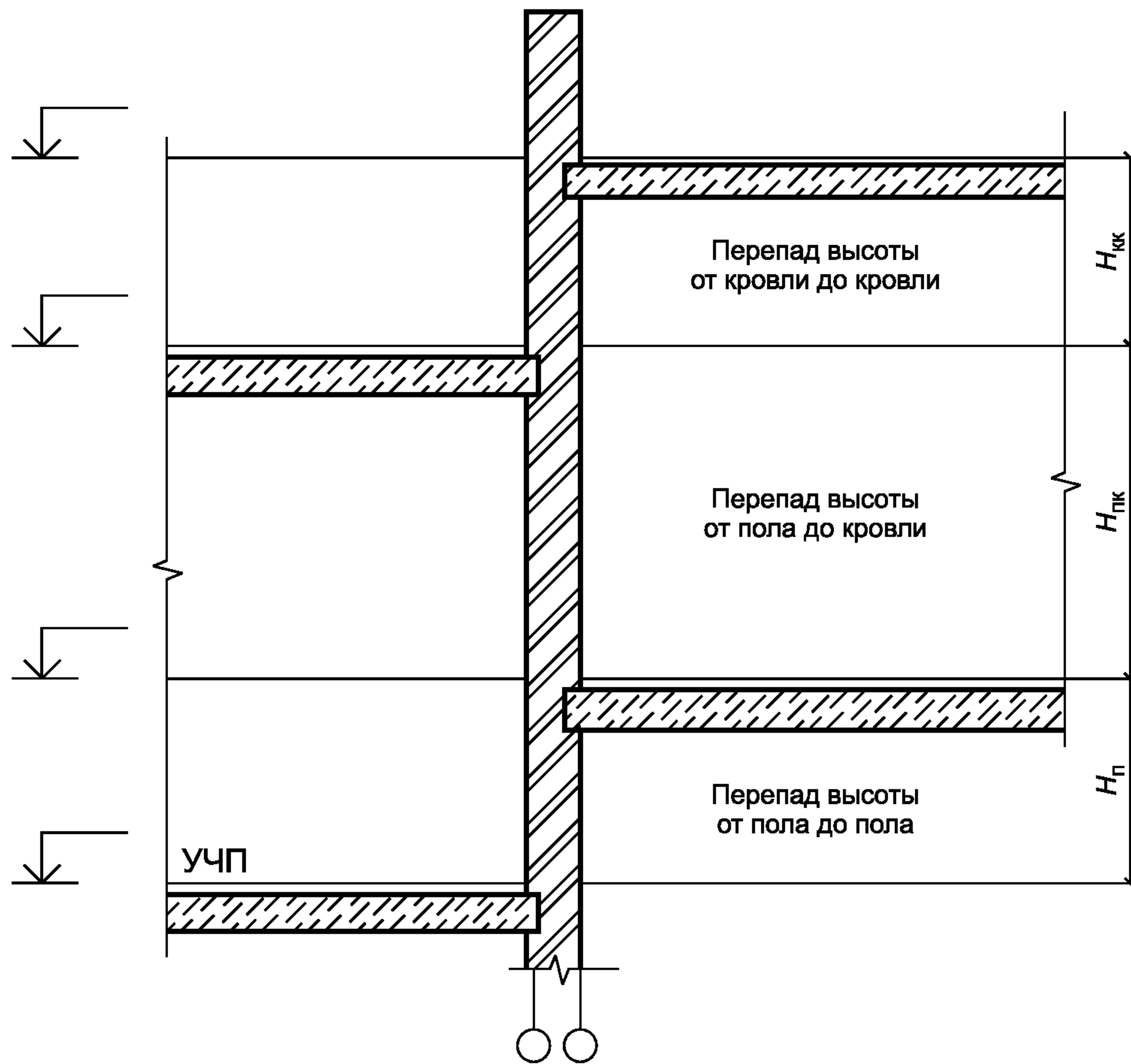
Рисунок 8 — Изменение уровня этажей или кровли (перепад высоты)
