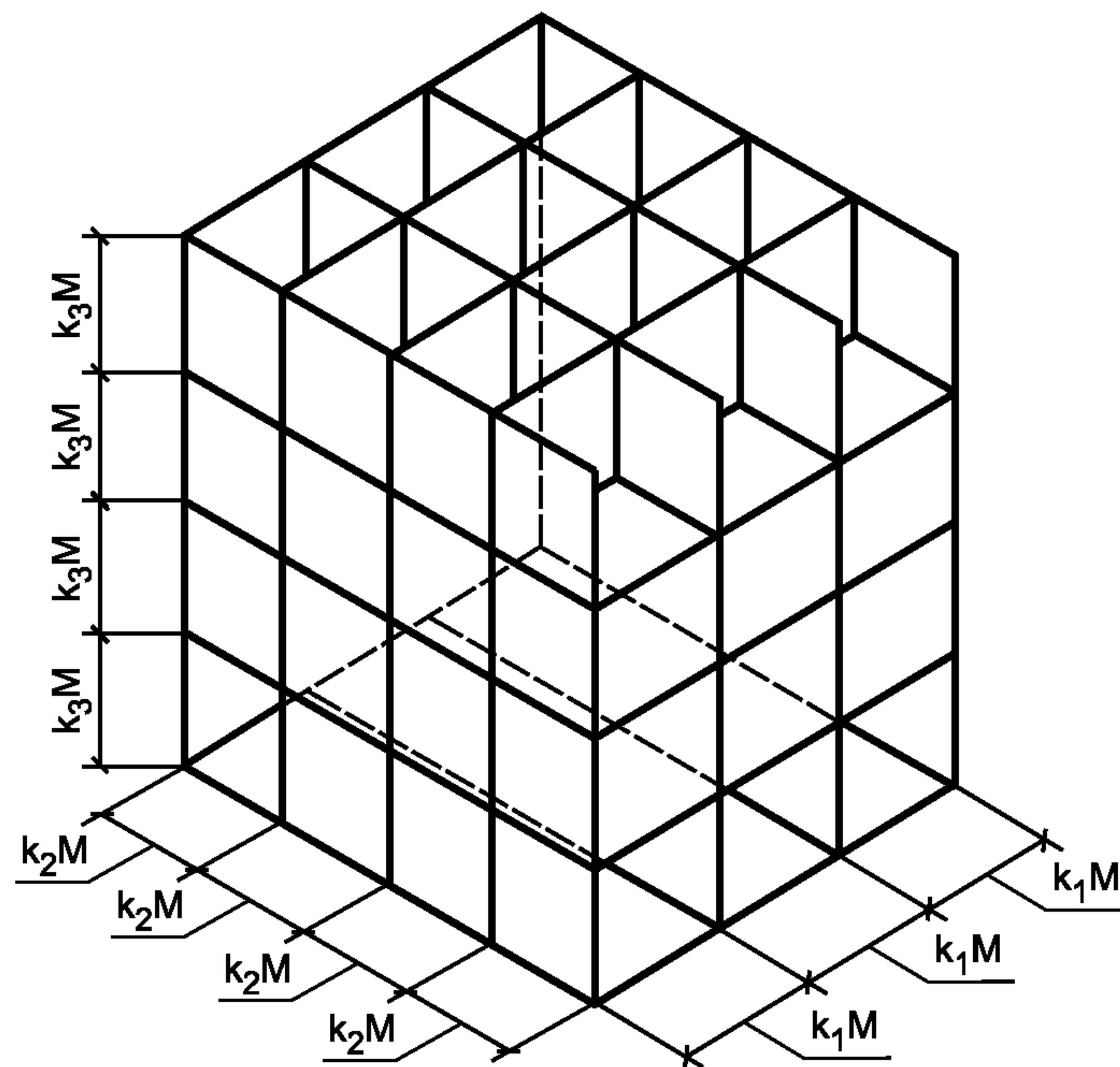
Рисунок 1 — Прямоугольная модульная координационная система
