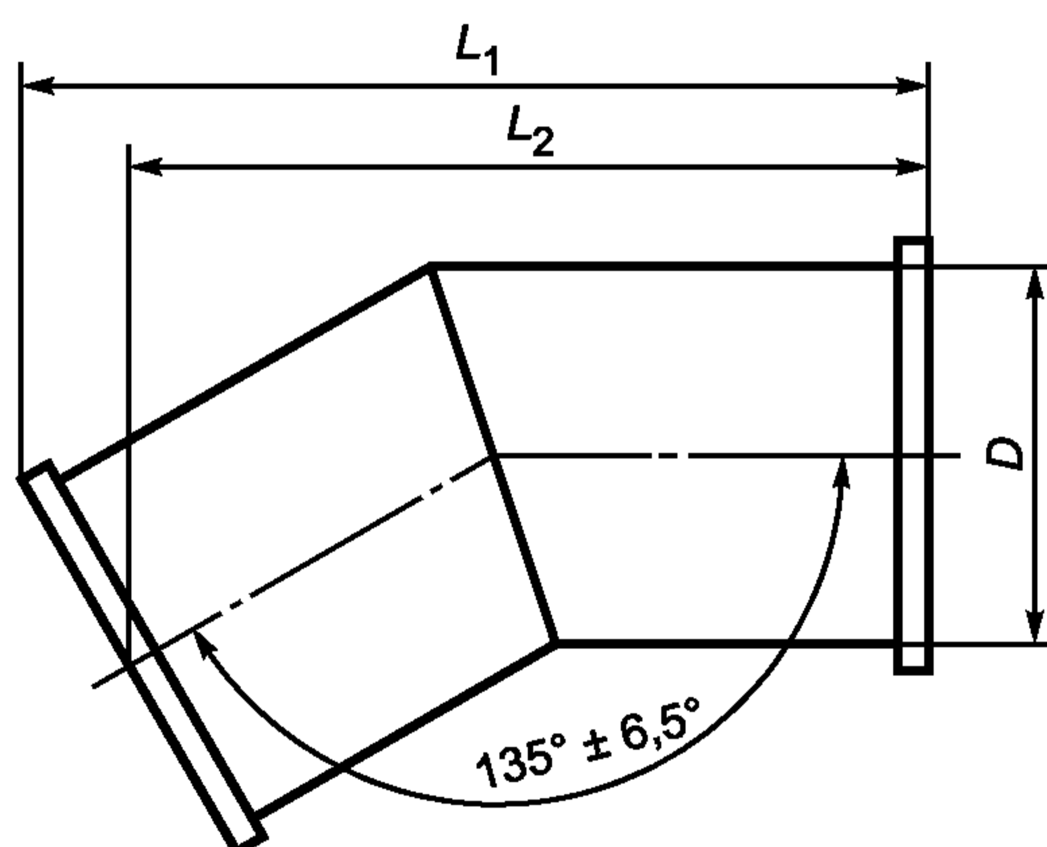
Рисунок А.4 — Размеры колена 135°
