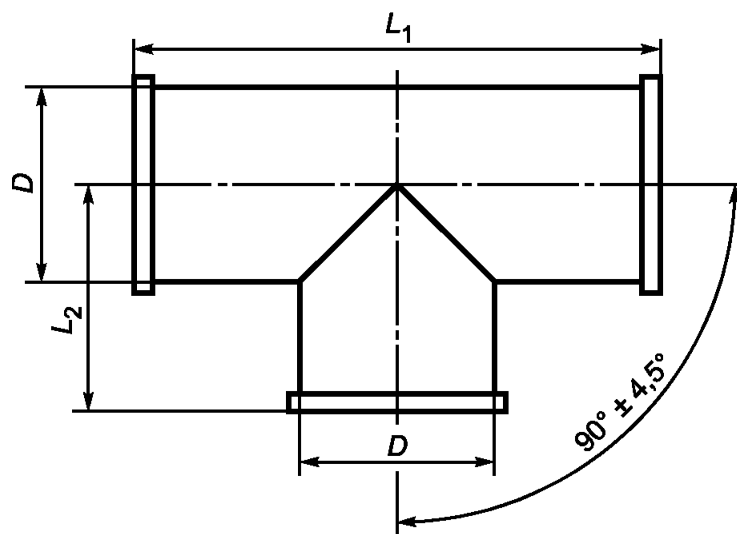
Рисунок А.6 — Тройник 90°
