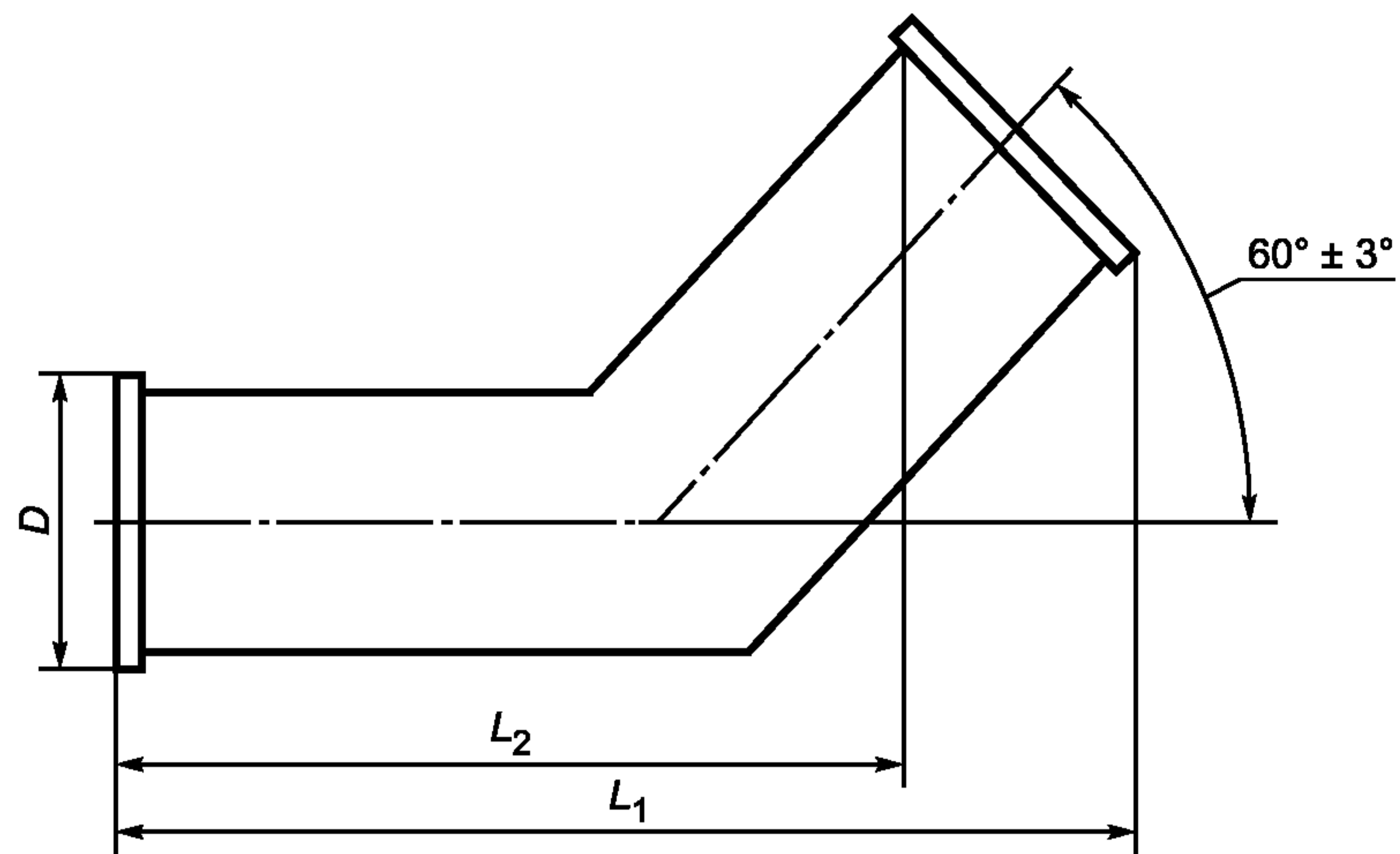
Рисунок А.5 — Колено 60°
