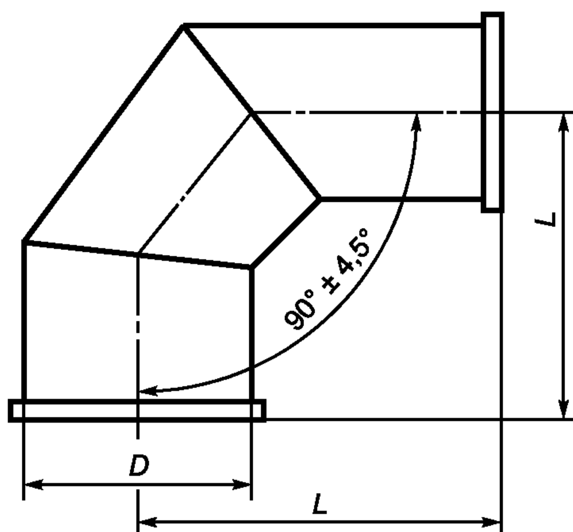
Рисунок А.3 — Размеры колена 90°
