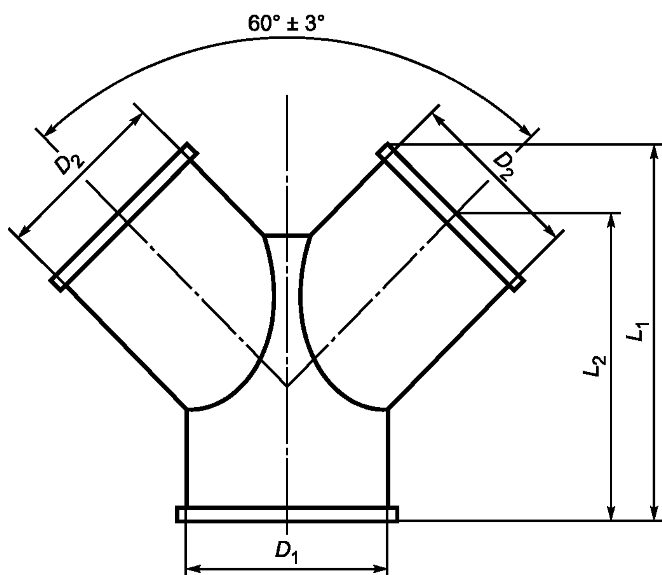
Рисунок А.8 — Тройник вилкообразный
