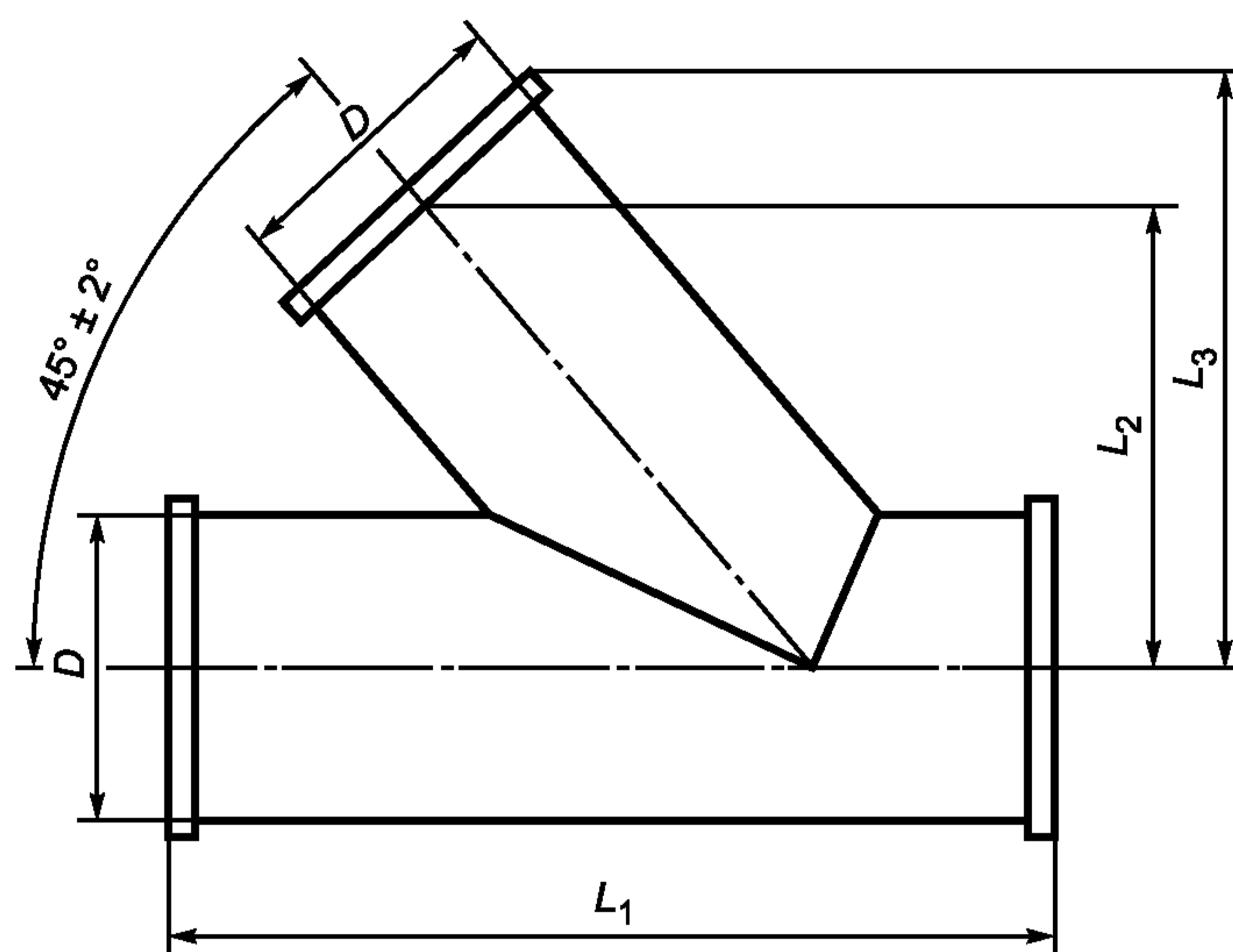
Рисунок А.7 — Тройник 45°
