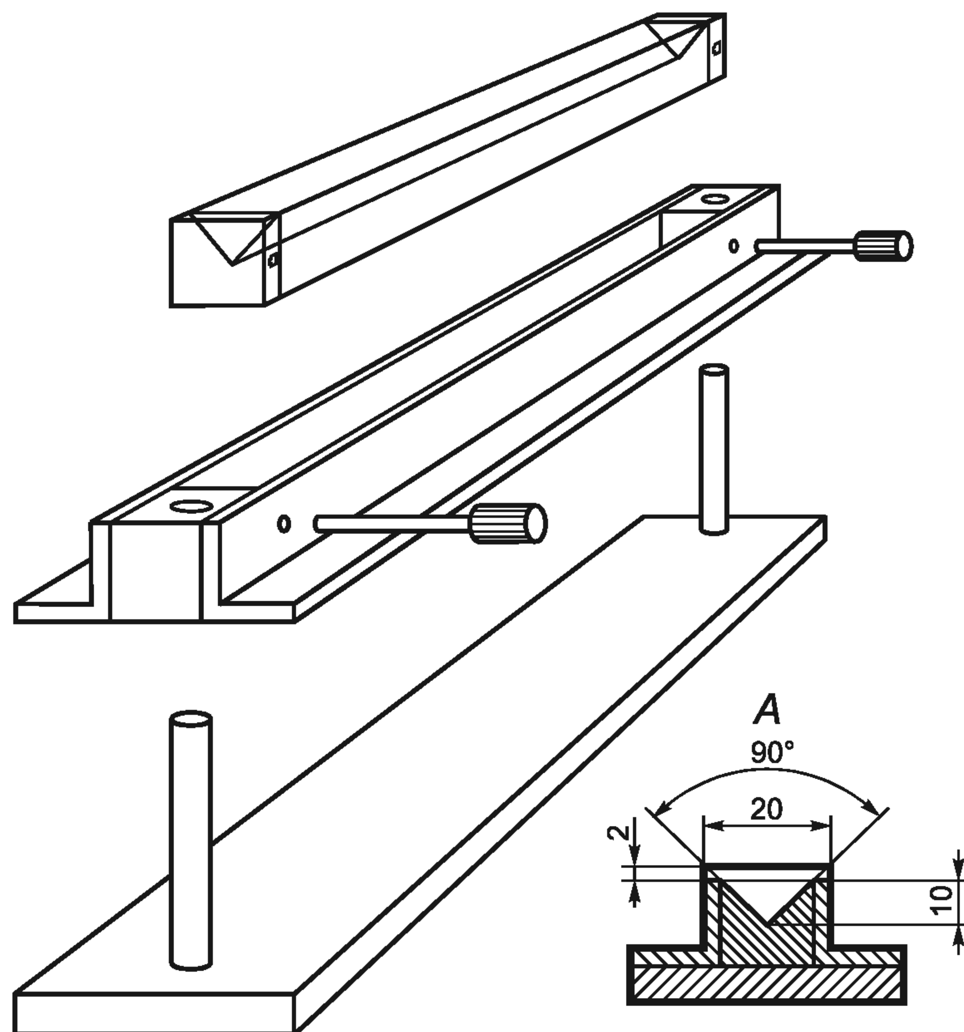
A — поперечное сечение лотка длиной 250 мм
