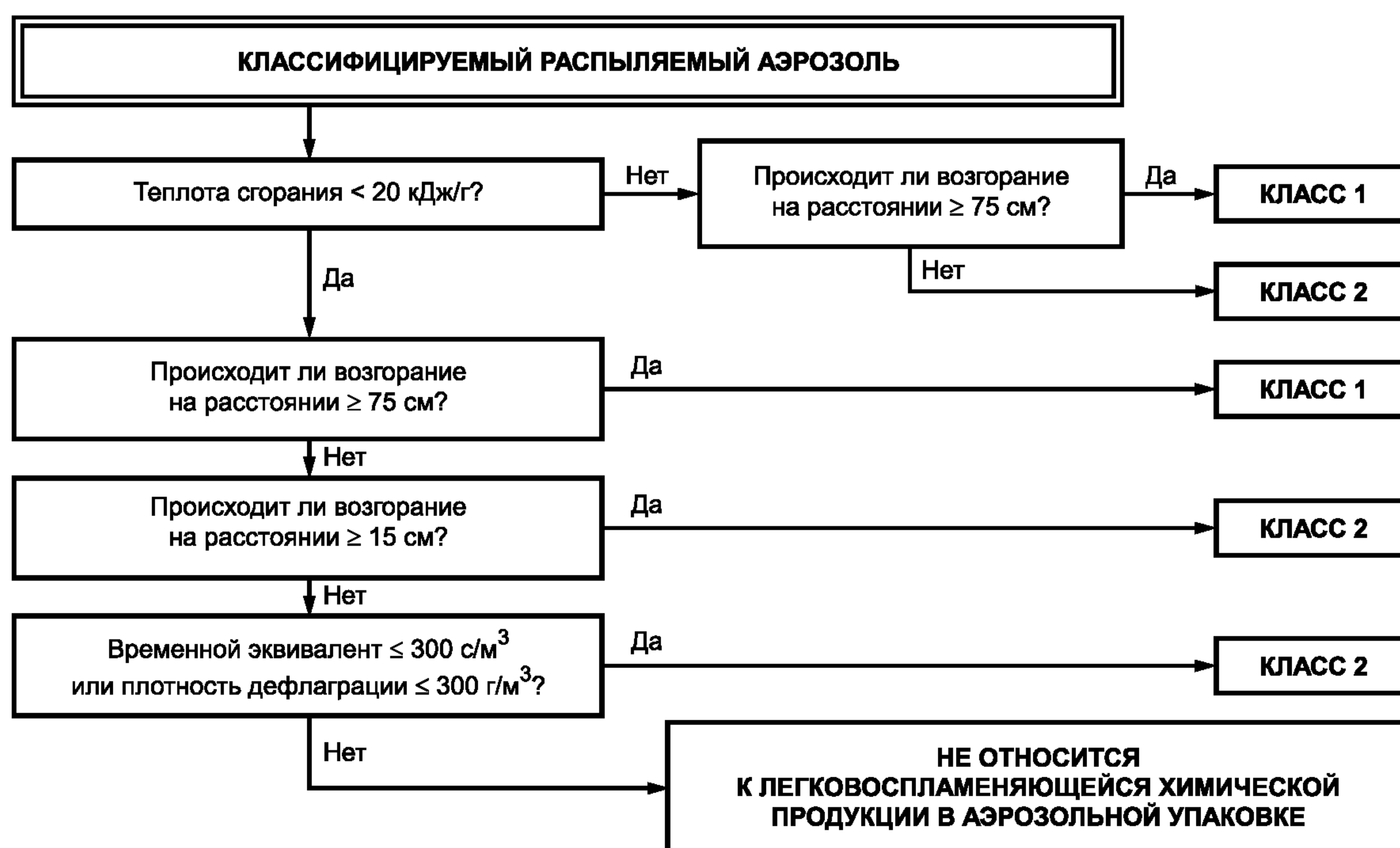
Рисунок 2 — Процедура классификации химической продукции, являющейся распыляемым аэрозолем
