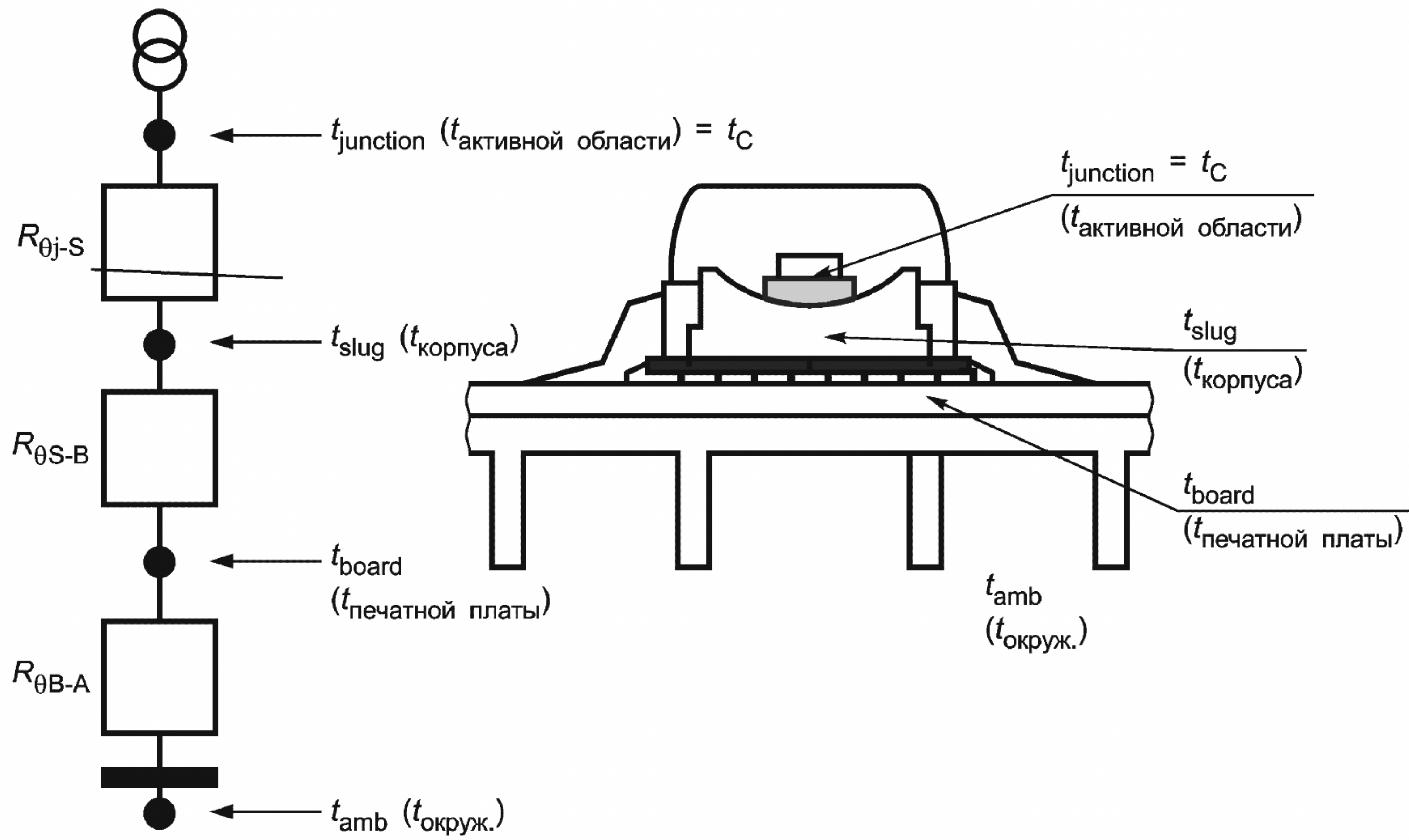
Рисунок 1 — Схематическая цепочка тепловых сопротивлений
