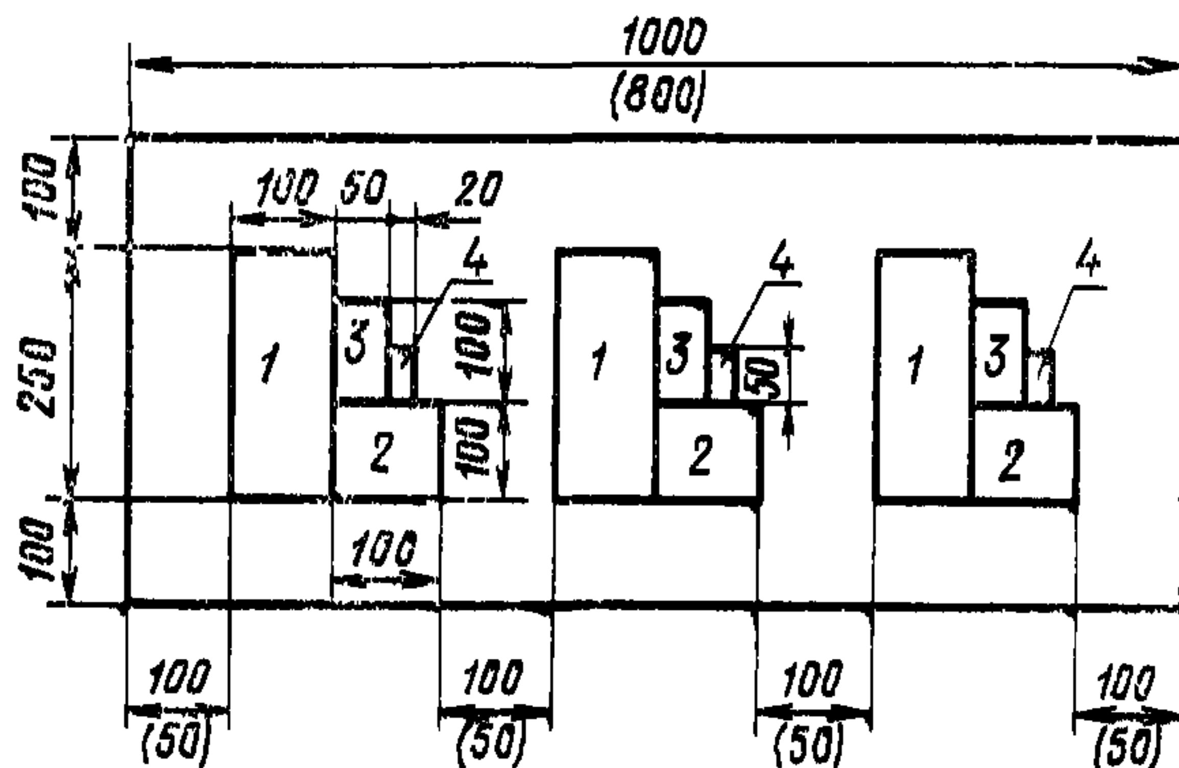
1 — полоски изола, из которых вырезают образцы для определения предела прочности при разрыве, относительного и остаточного удлинения; 2 — образцы для определения водопоглощения; 3 — образцы для определения температуроустойчивости; 4 — образцы для определения гибкости.
