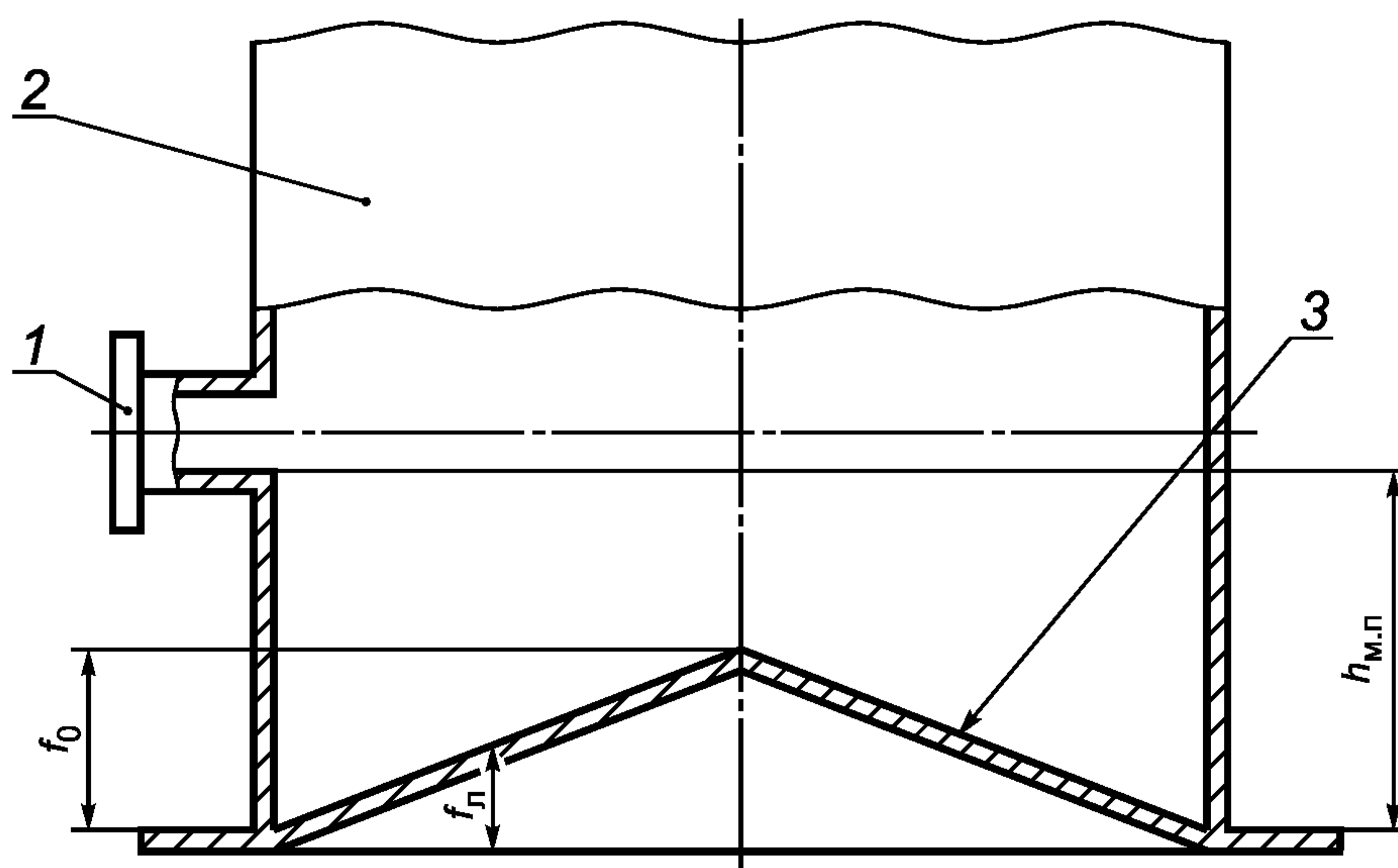
1 — приемо-раздаточный патрубок; 2 — стенка резервуара; 3 — неровности дна; f_0 — высота неровностей дна; f_{л} — высота точки касания дна грузом рулетки; h_{м.п} — высота «мертвой» полости
