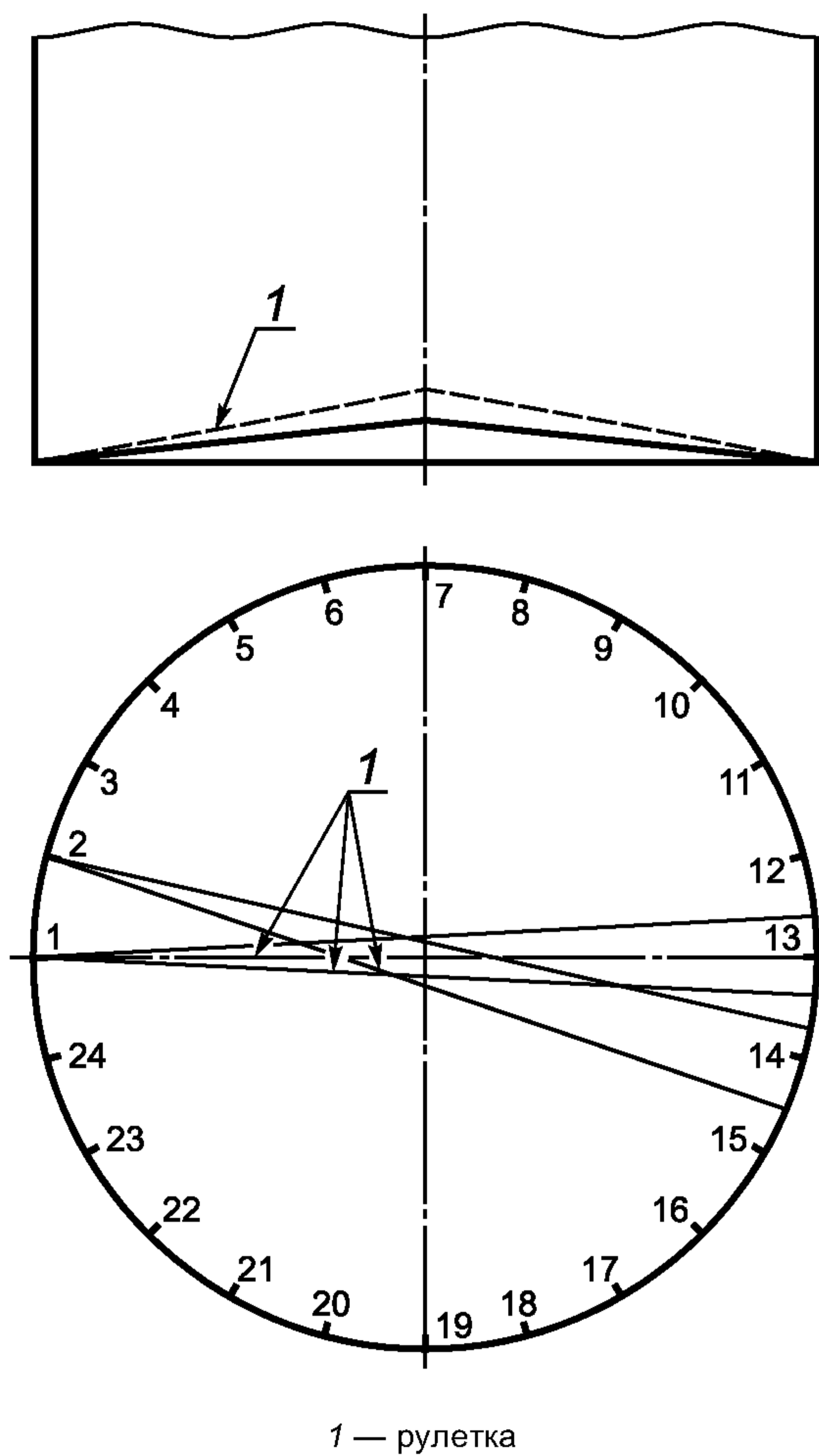
Рисунок Б.1 — Схема определения центра резервуара
