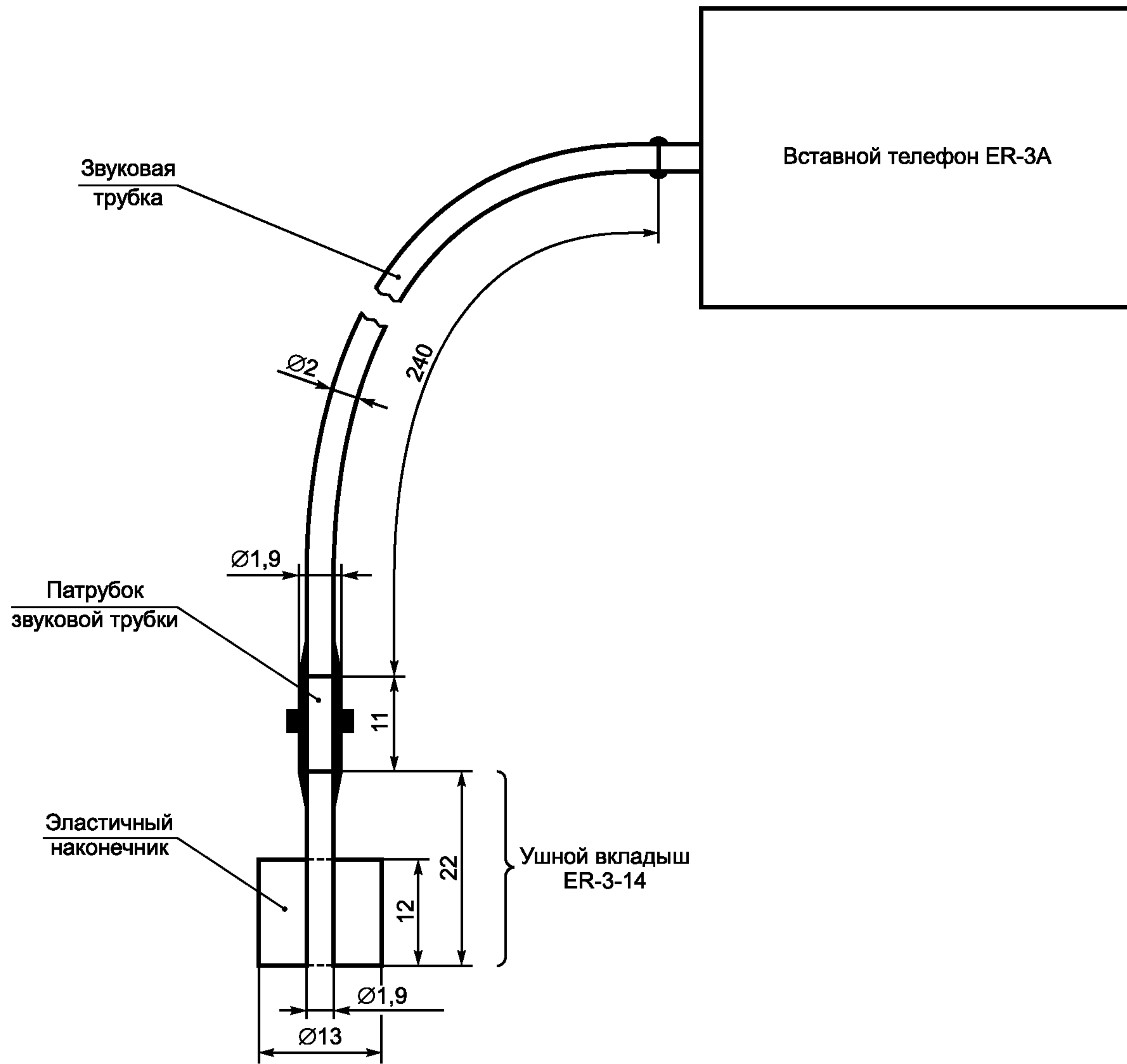
Рисунок 1 — Вставной телефон ER-3A и ушной вкладыш ER-3-14
