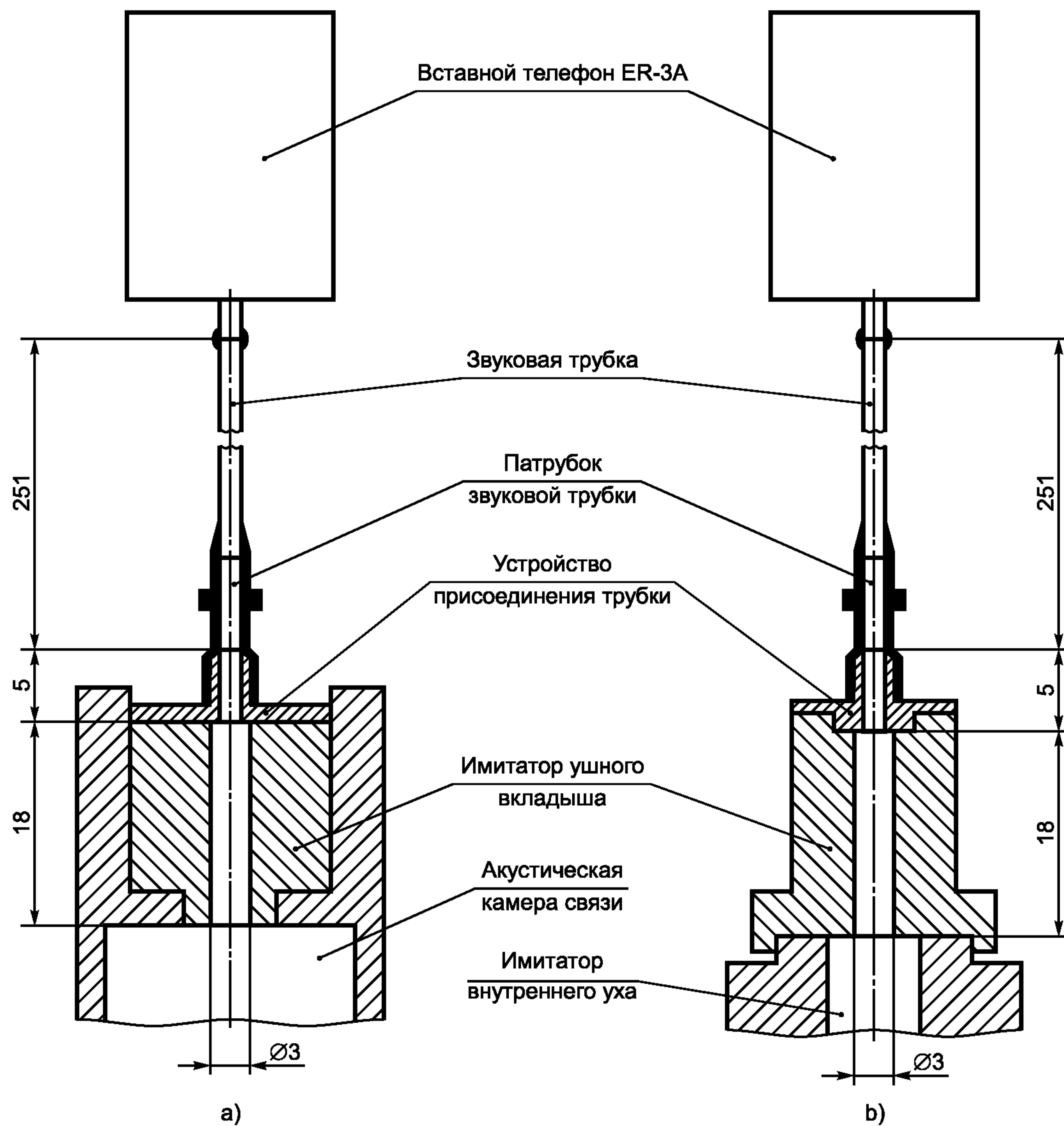
а) к акустической камере связи; б) к имитатору внутреннего уха
