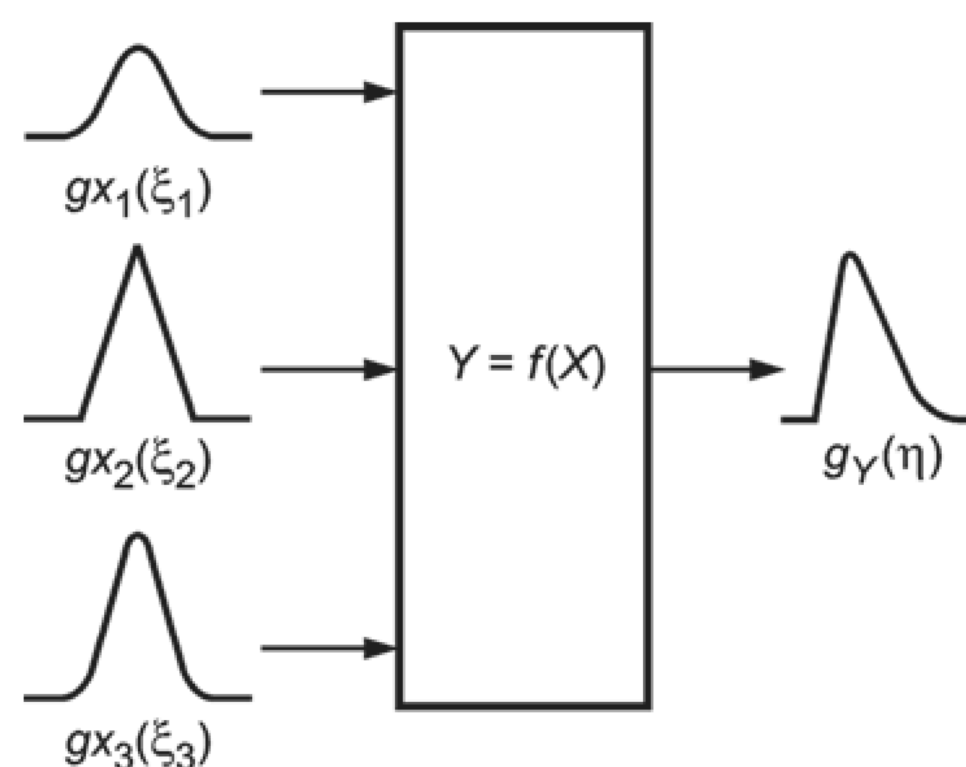
Рисунок 2 — Трансформирование распределений трех ( N = 3 ) независимых входных величин
