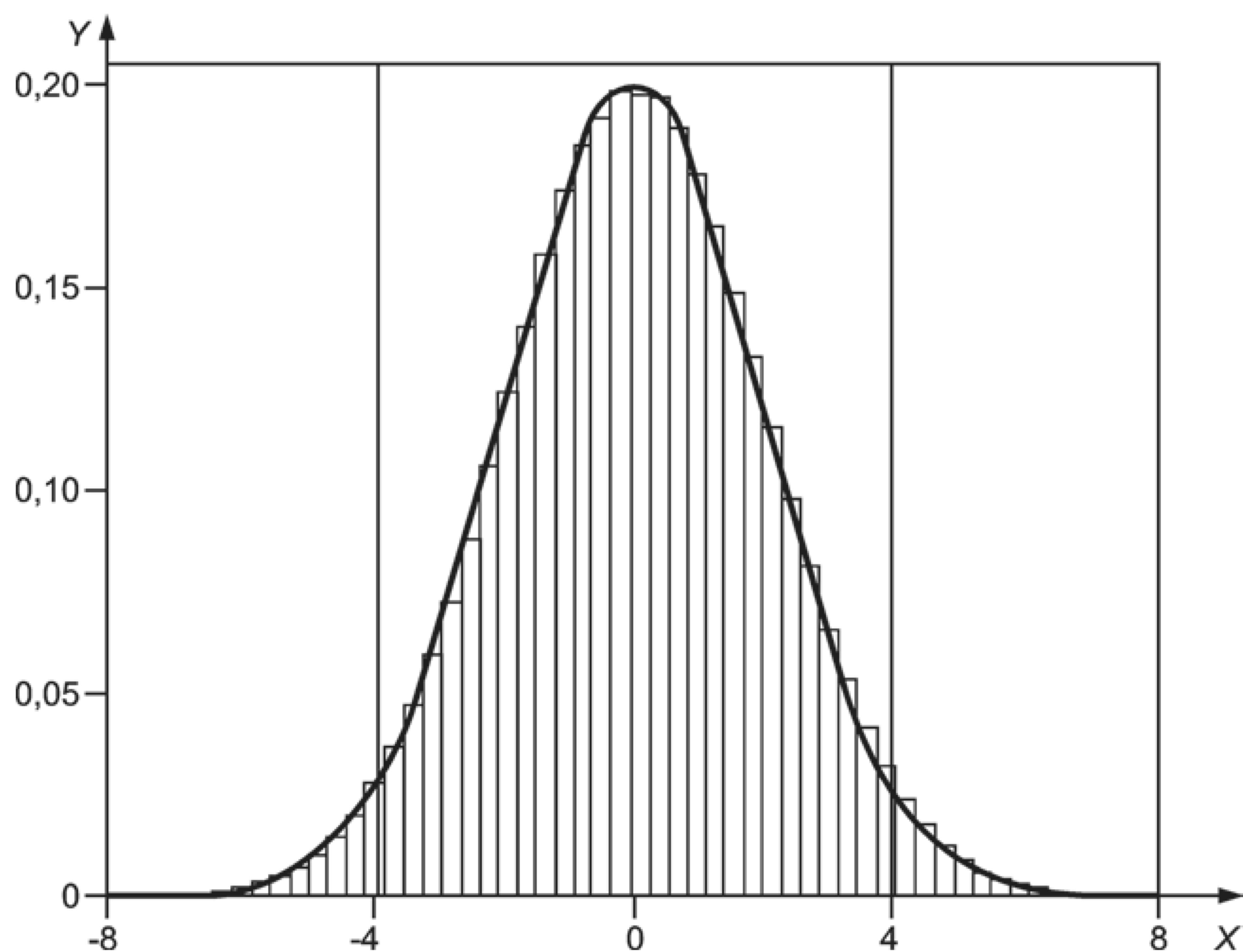
X — величина (безразмерная); Y — плотность распределения вероятностей
