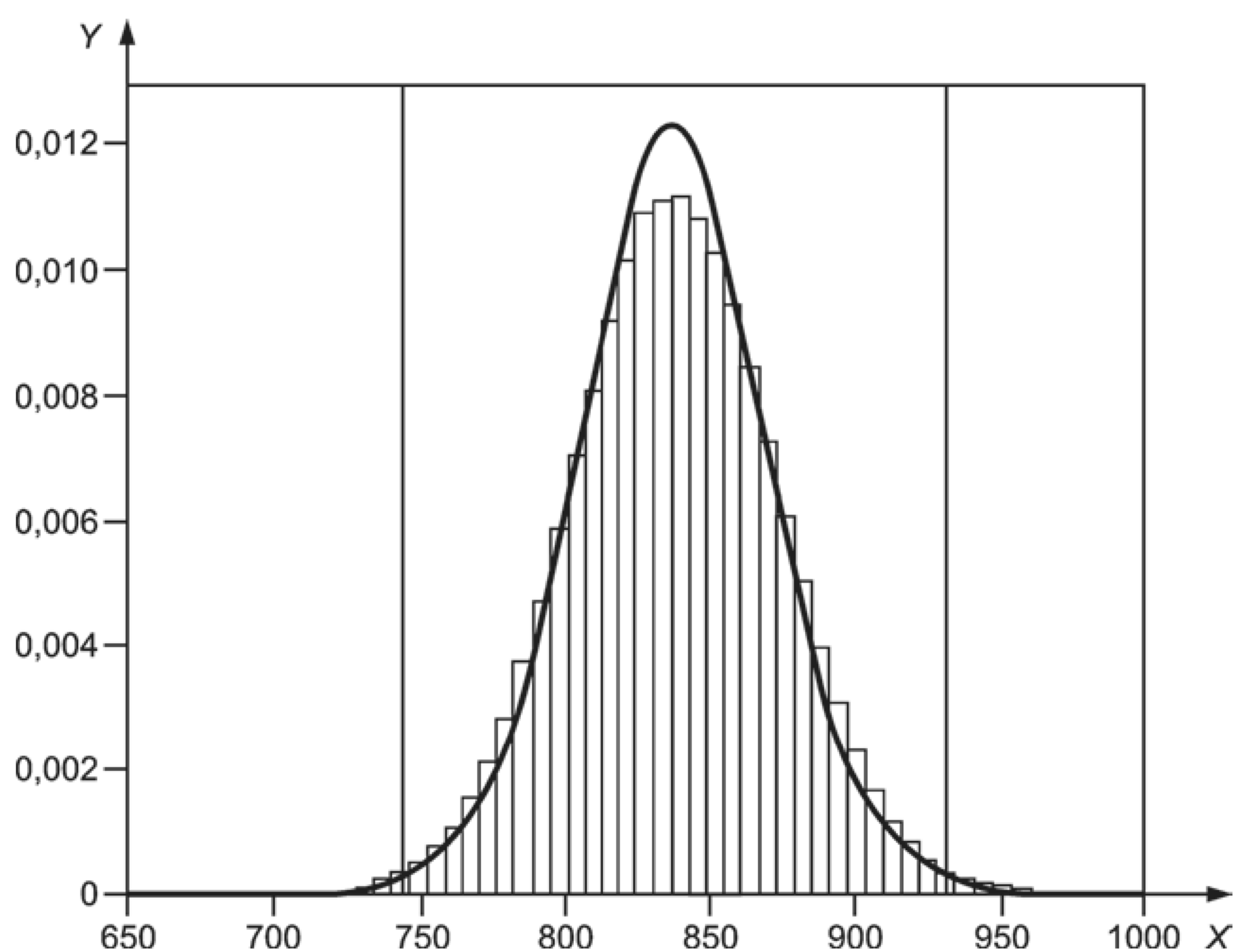
X — отклонение длины калибруемой концевой меры длины от номинала, нм; Y — плотность распределения вероятностей, нм -1
