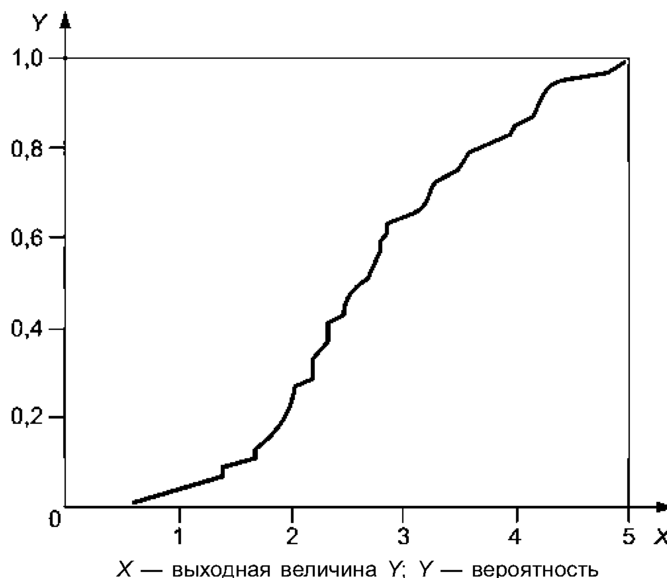
Рисунок D.1 — Аппроксимация \tilde{G}_Y(\eta) функции распределения G_Y(\eta)
