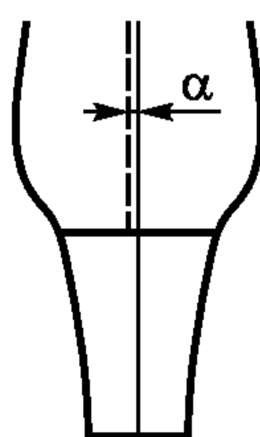
Рисунок 9 — Измерение перекоса каблука
