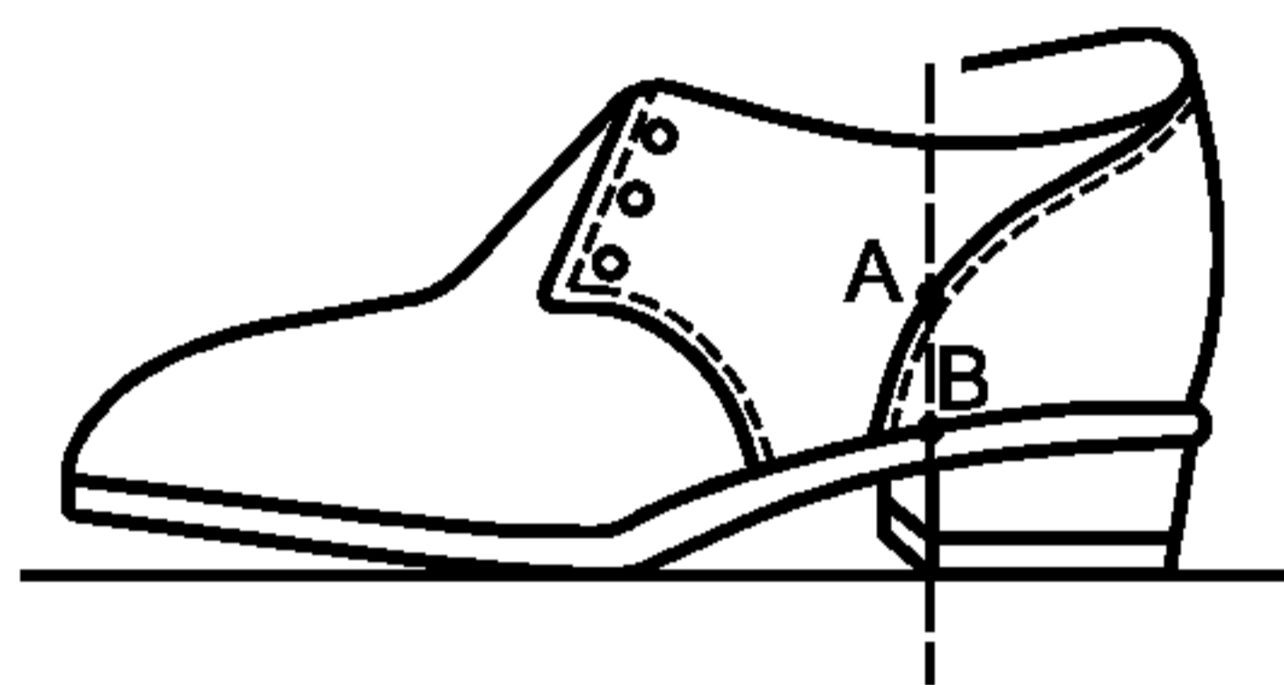
Рисунок 8 — Измерение перекоса накладных задников (задников)
