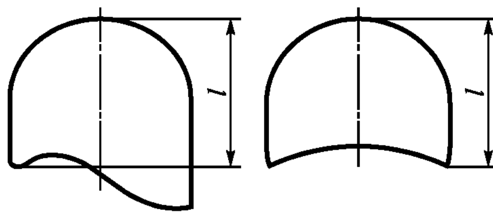
Рисунок 4 — Измерение длины каблука и набойки
