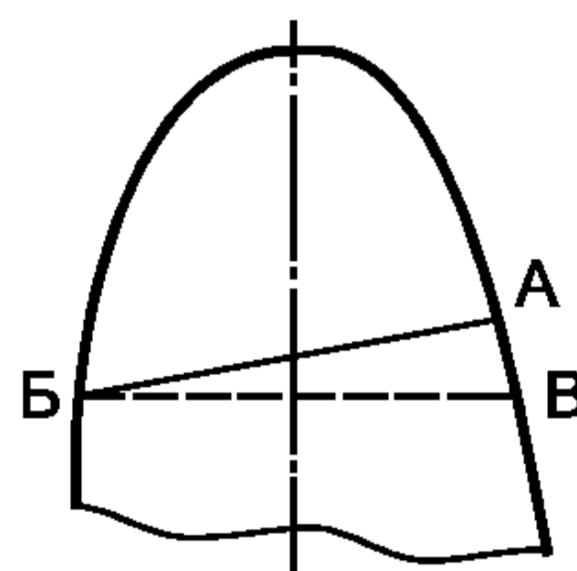
Рисунок 5 — Измерение перекоса носка
