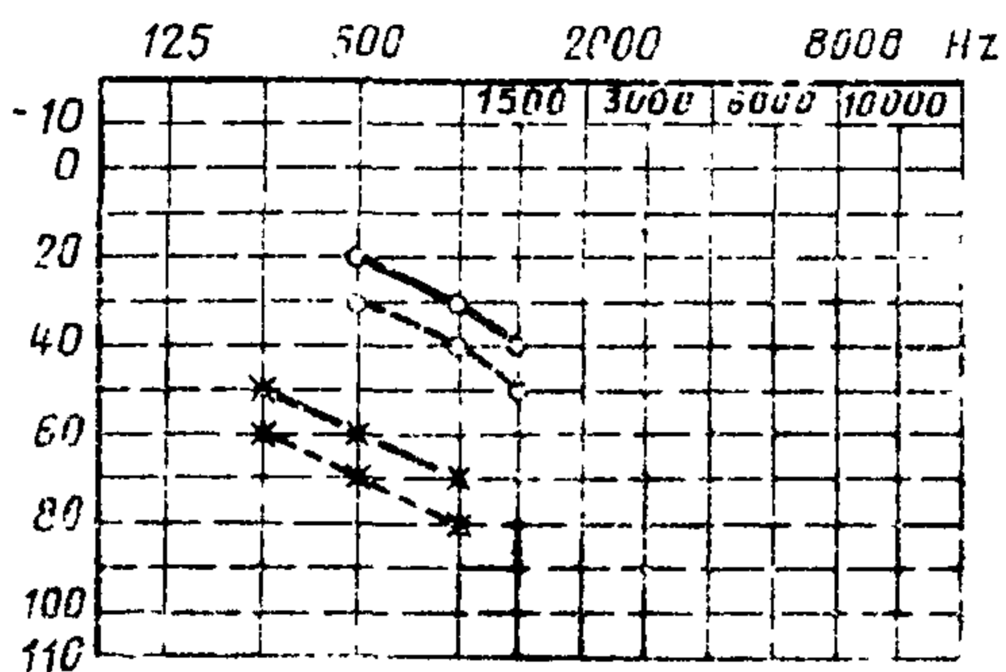
Аудиограмма
