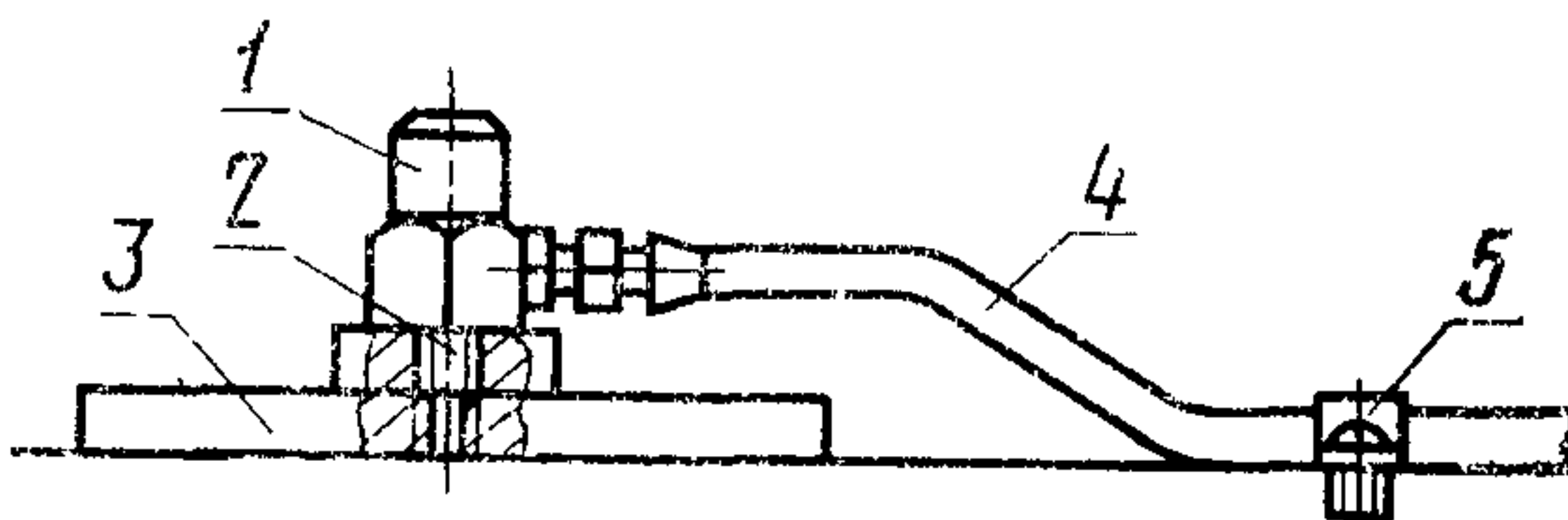
1—вибропреобразователь; 2—шпилька; 3—диск; 4—кабель. 5—скоба
