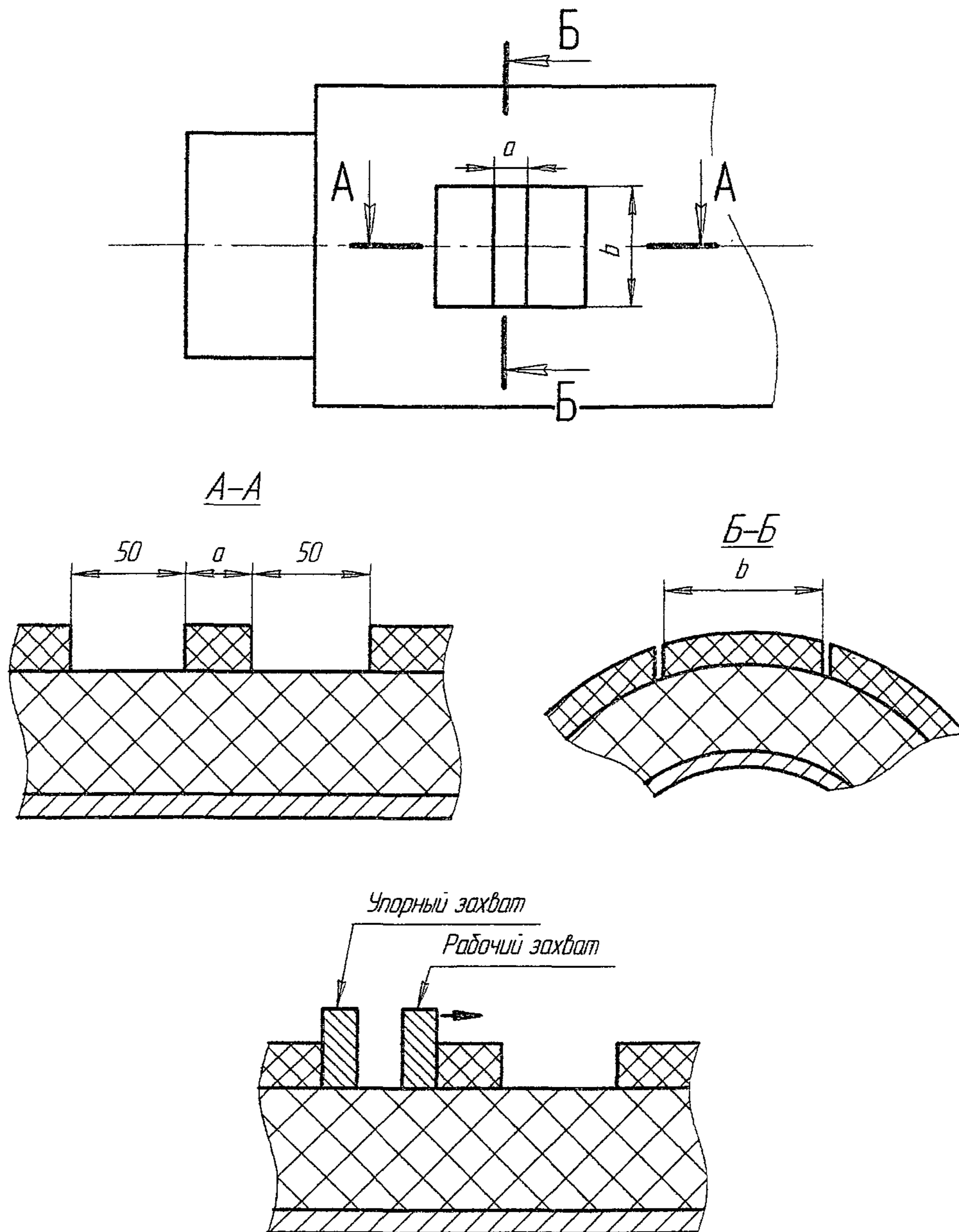
Рисунок В1 – Образцы для испытаний
