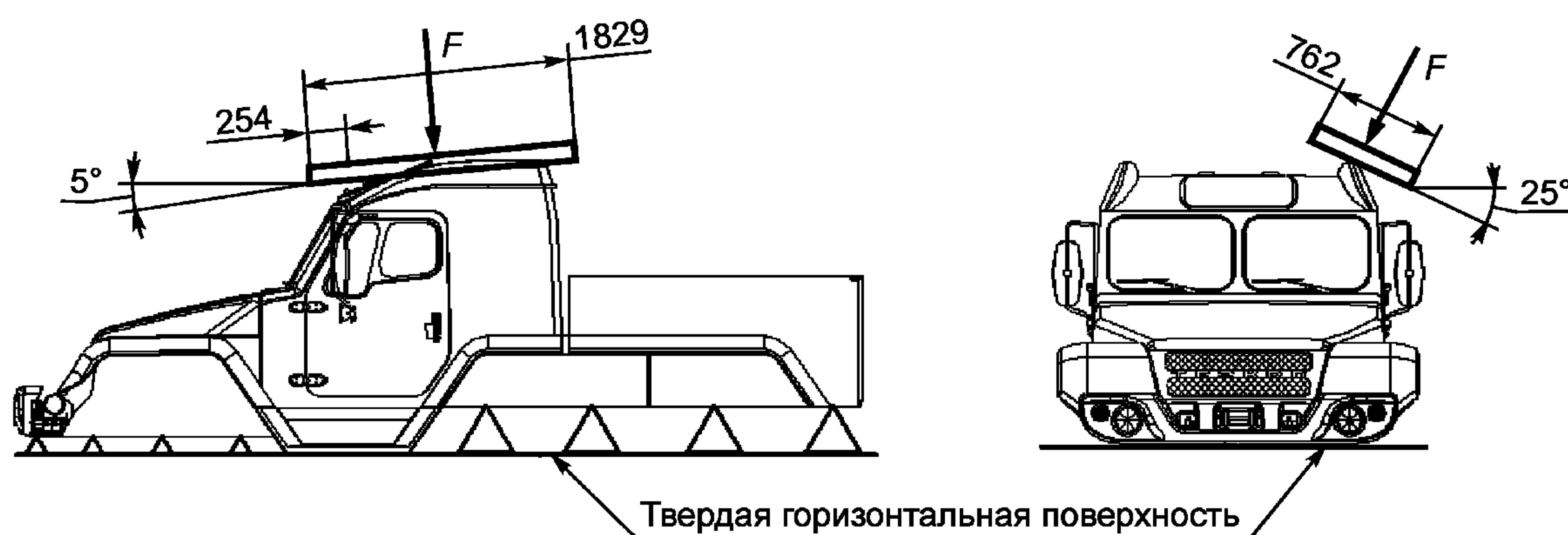
Рисунок 1 — Схема испытания защитных свойств кузова/кабины
