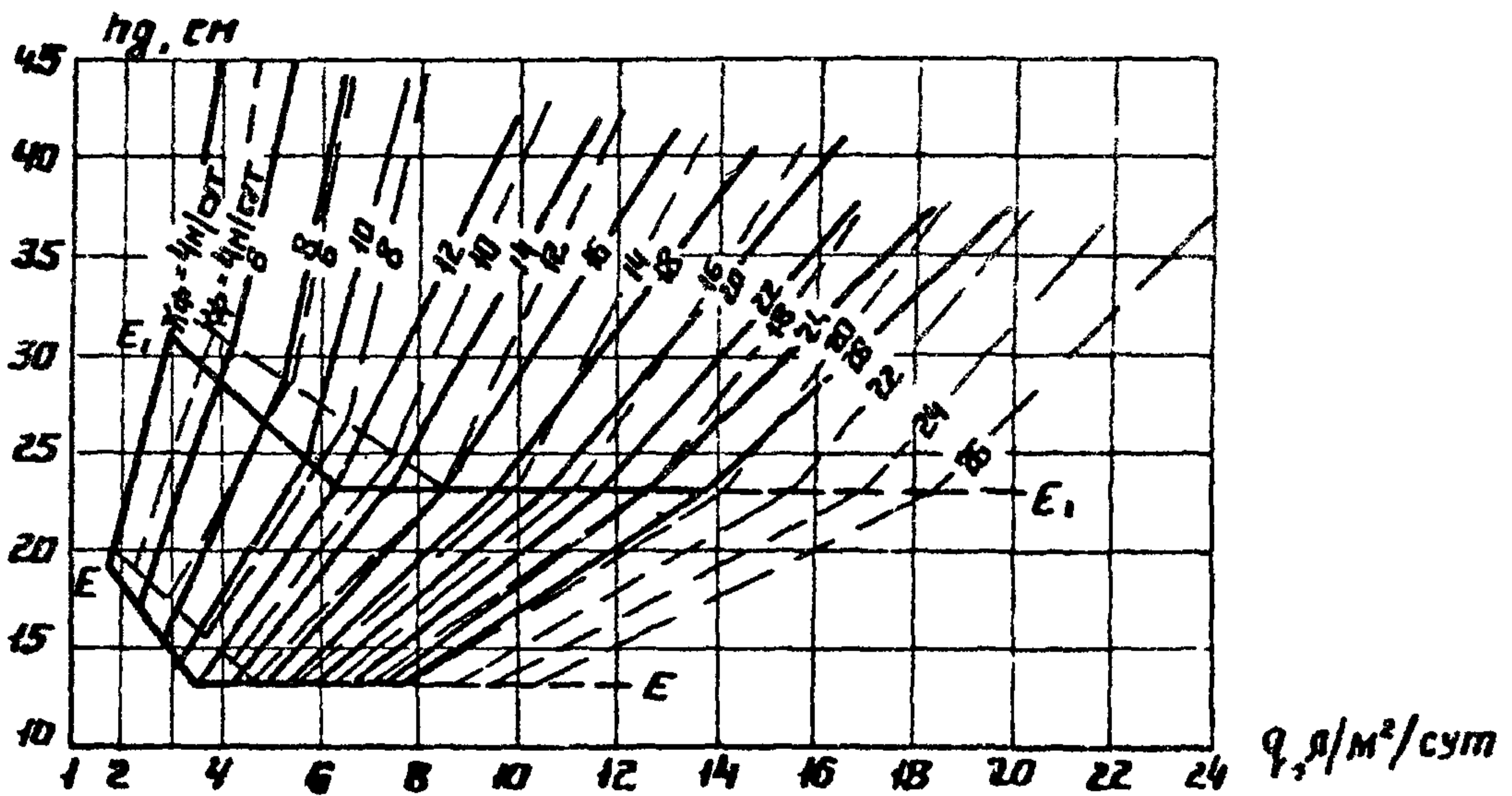
Рис. 14 График для определения толщины дренажного слоя при поперечном профиле дорожной одежды с индексом \Gamma и пути фильтрации 4 м Обозначения те же, что и на рис. 7
