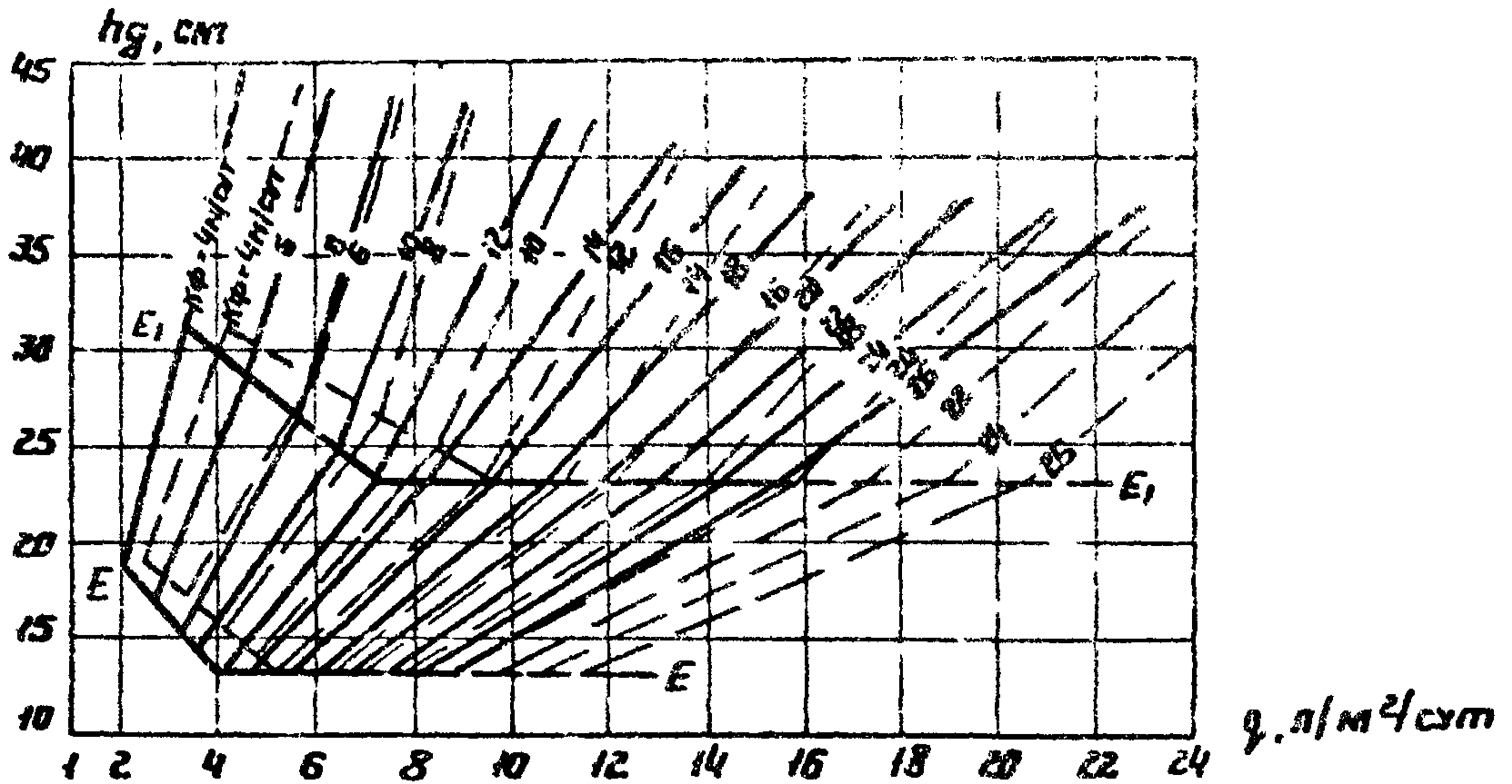
Рис. 13 График для определения толщины дренажного слоя при поперечном профиле дорожной одежды с индексом \Gamma и пути фильтрации 10 м Обозначения те же, что и на рис. 7
