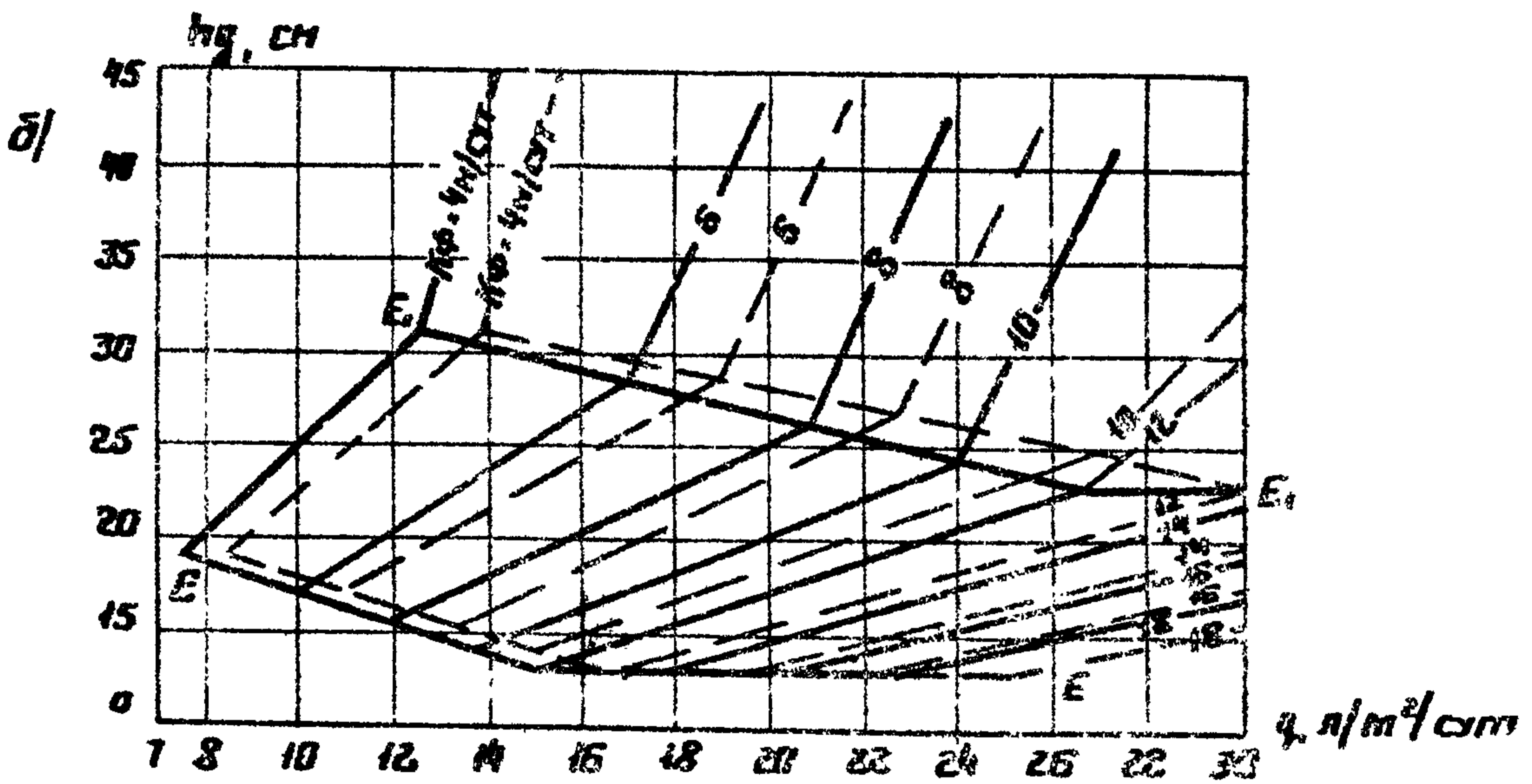
Рис. 18 График для определения толщины дренирующего слоя при поперечном профиле дренажной овражной с индексом Д и пути фильтрации 7 м а - глубина ровика 25 см; б - глубина ровика - 45 см Обозначение те же, что и на рис. 7
