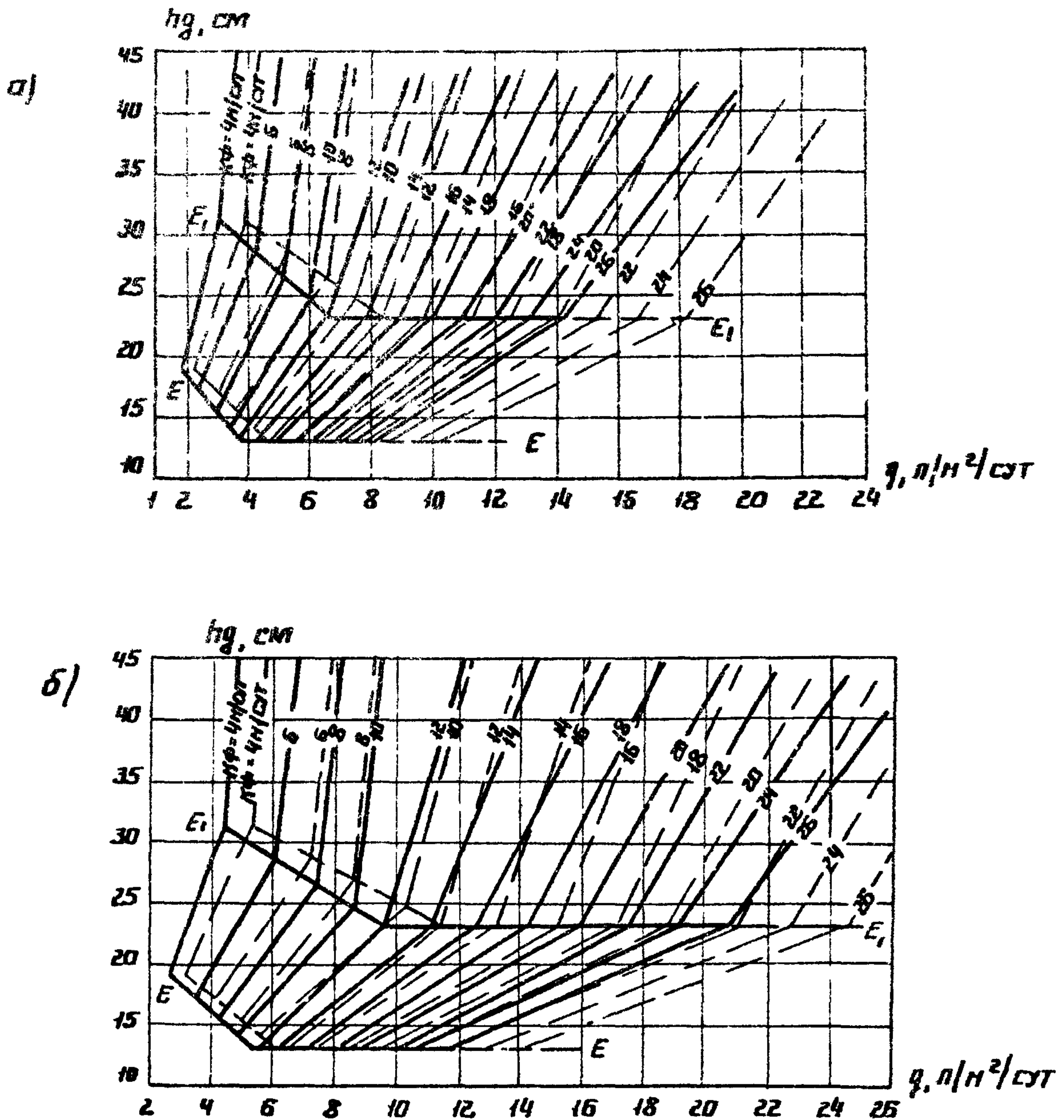
Рис 24 График для определения толщины дренажного слоя при поперечном профиле дорожной одежды с индексом Д и пути фильтрации 13 м а - глубина ровика 25 см; б - глубина ровика - 45 см. Обозначения те же, что и на рис. 7
