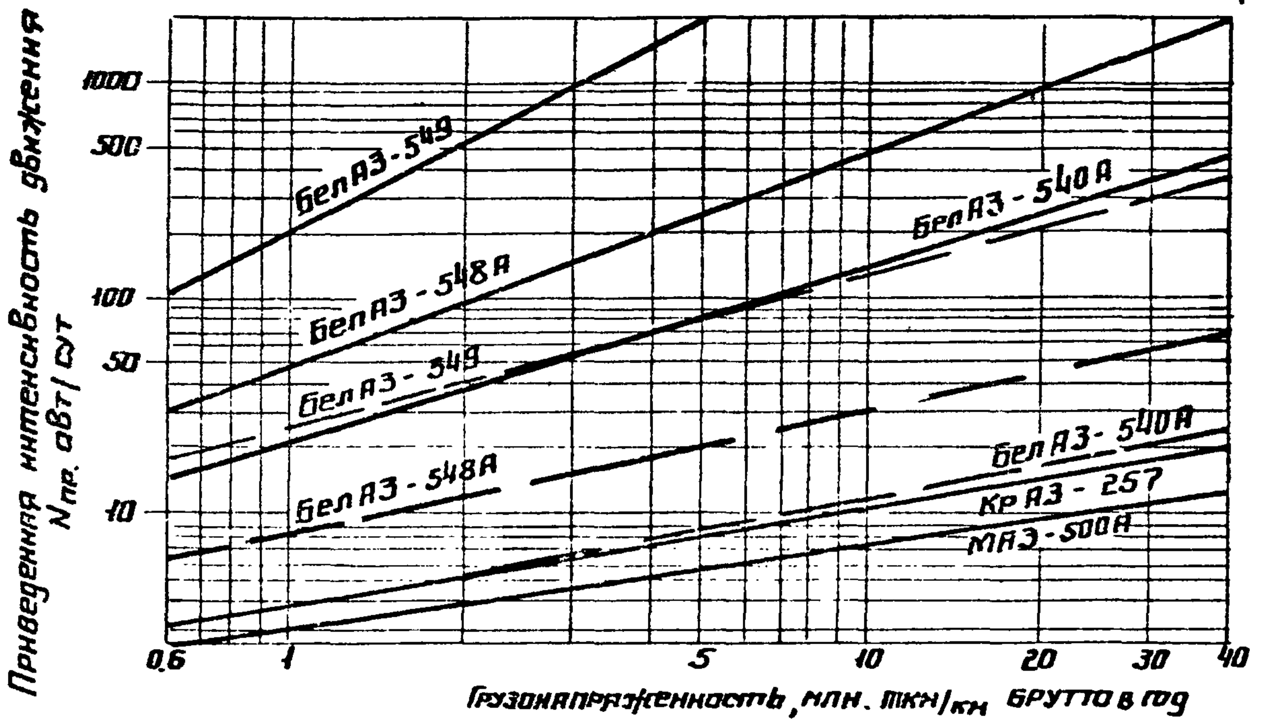
Рис 30 Номограмма для определения приведенной интенсивности движения к расчетному автомобилю БелАЗ-548. Обозначения те же, что и на Рис. 28
