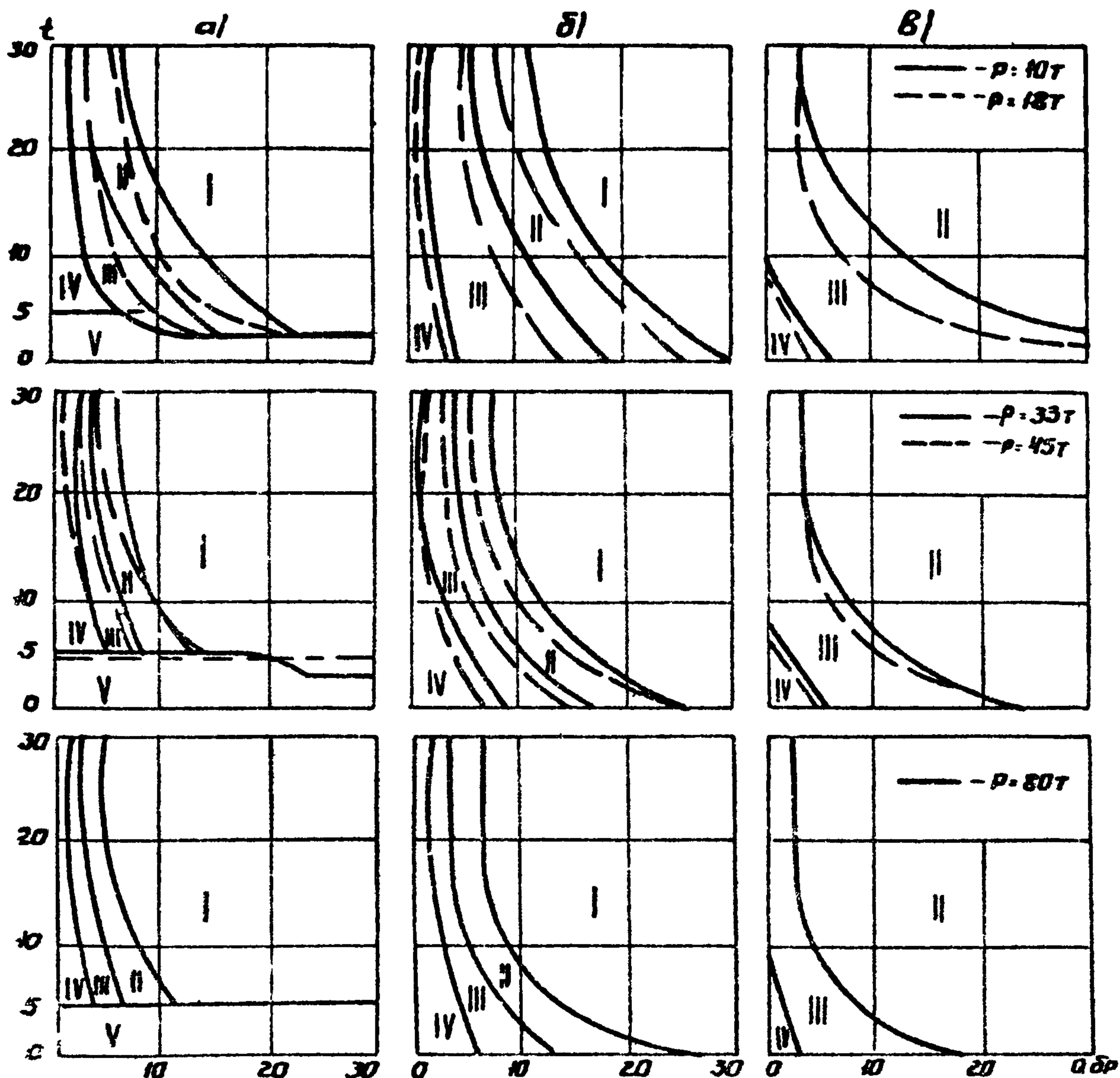
Рис. 1 Области экономически обоснованного применения различных типов покрытий
