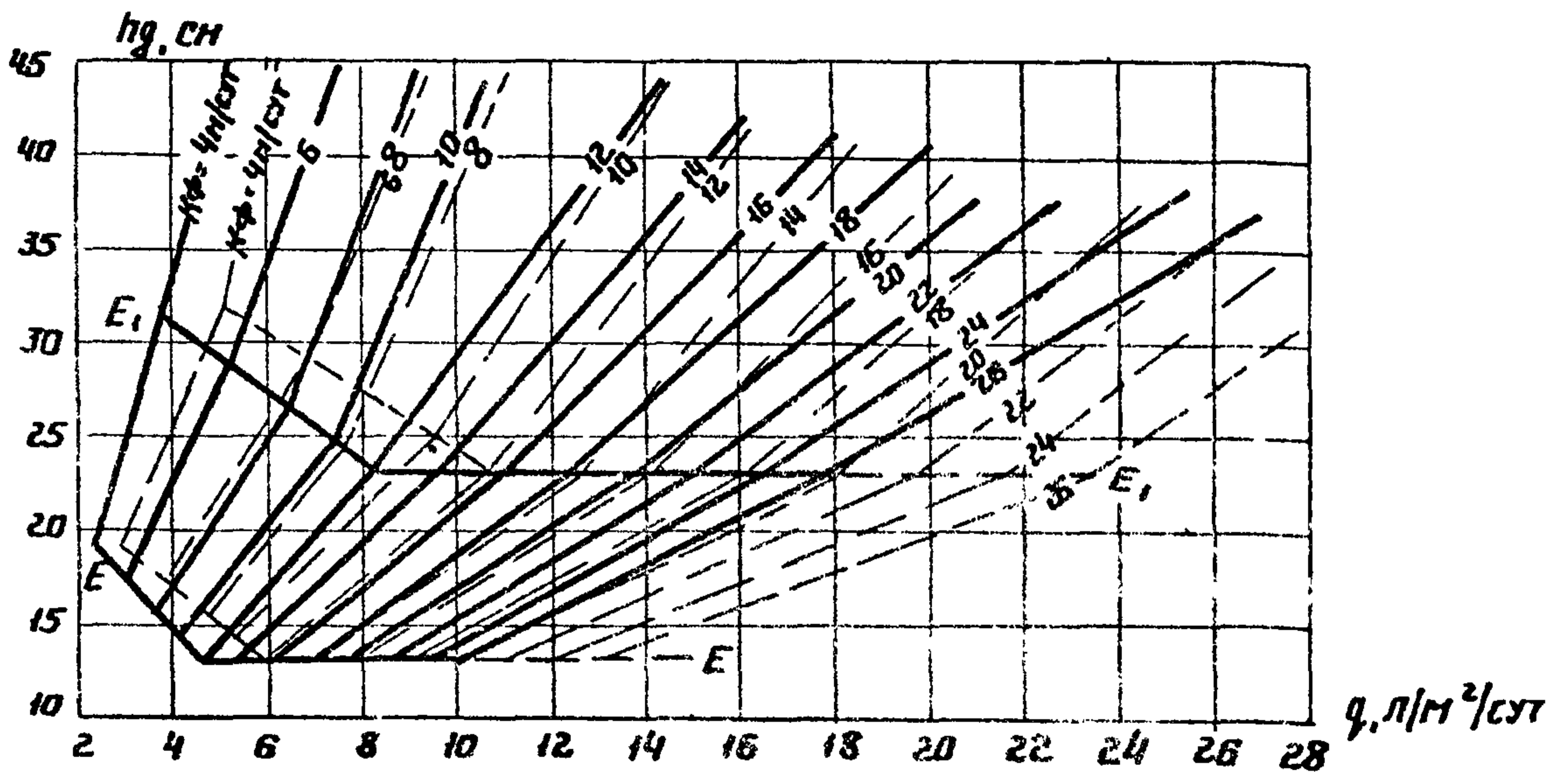
Рис. 12 График для определения толщины дренажного слоя при поперечном профиле дорожной одежды с индексом В и Г и пути фильтрации 9 м. Обозначения те же, что и на рис. 7
