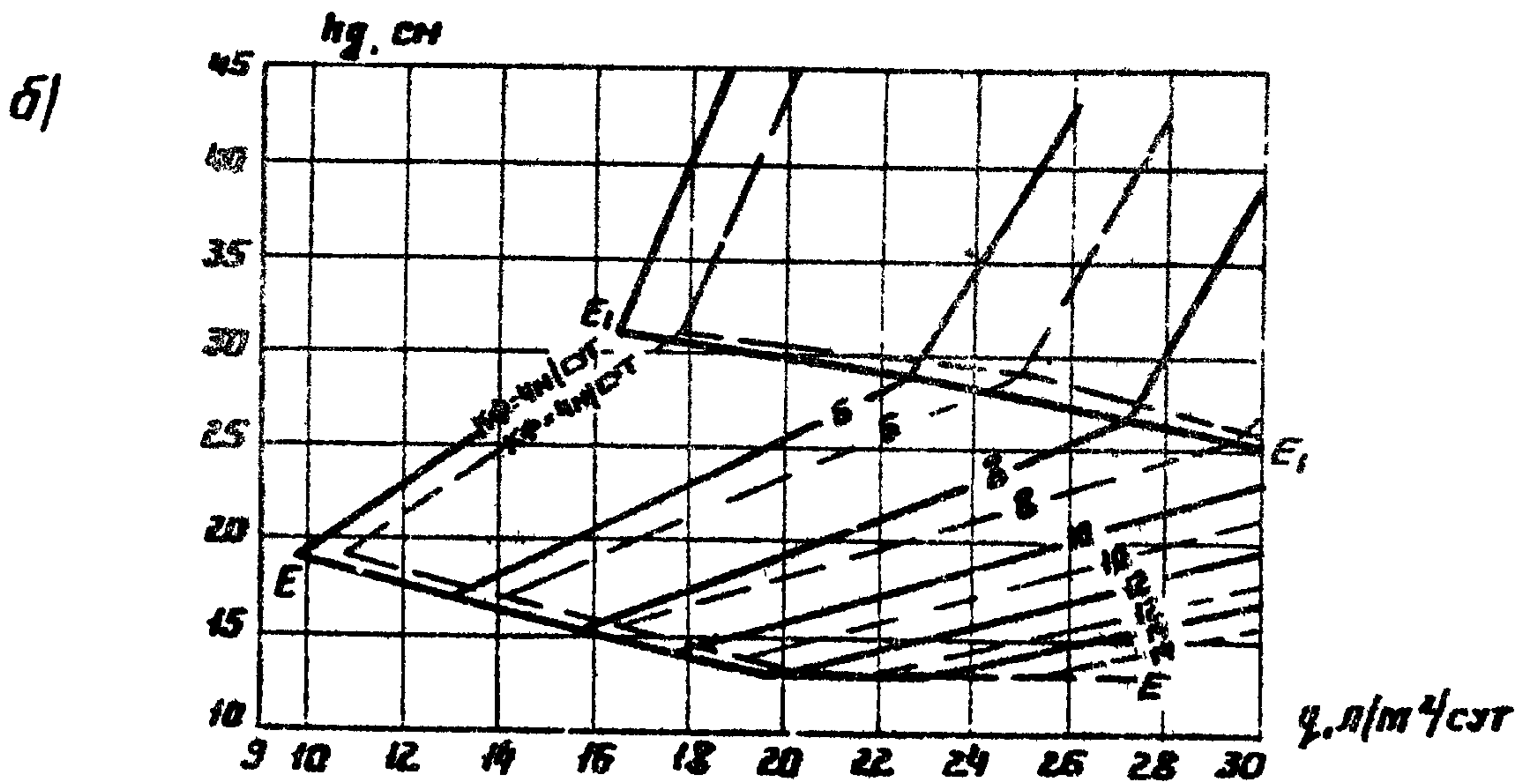
Рис. 17 ГРАФИКИ для определения толщины дренажного слоя при поперечном профиле дорожной одежды с индексом D и пути фильтрации B и а) толщина равна 25 см; б) толщина равна 45 см. Обозначения те же, что и на рис. 7
