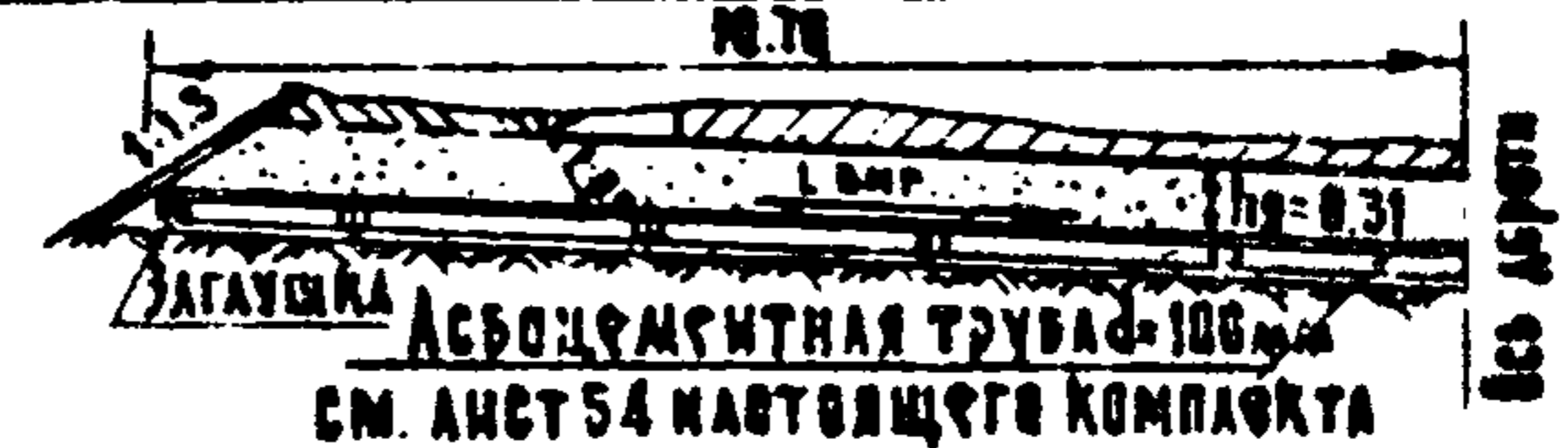
ПОПЕРЕЧНАЯ ПРОРЕЗЬ НА ВЫРАЖЕ ПРИ ПРОДАЛЬНОМ УКЛОНЕ ВЫШЕ 40%
