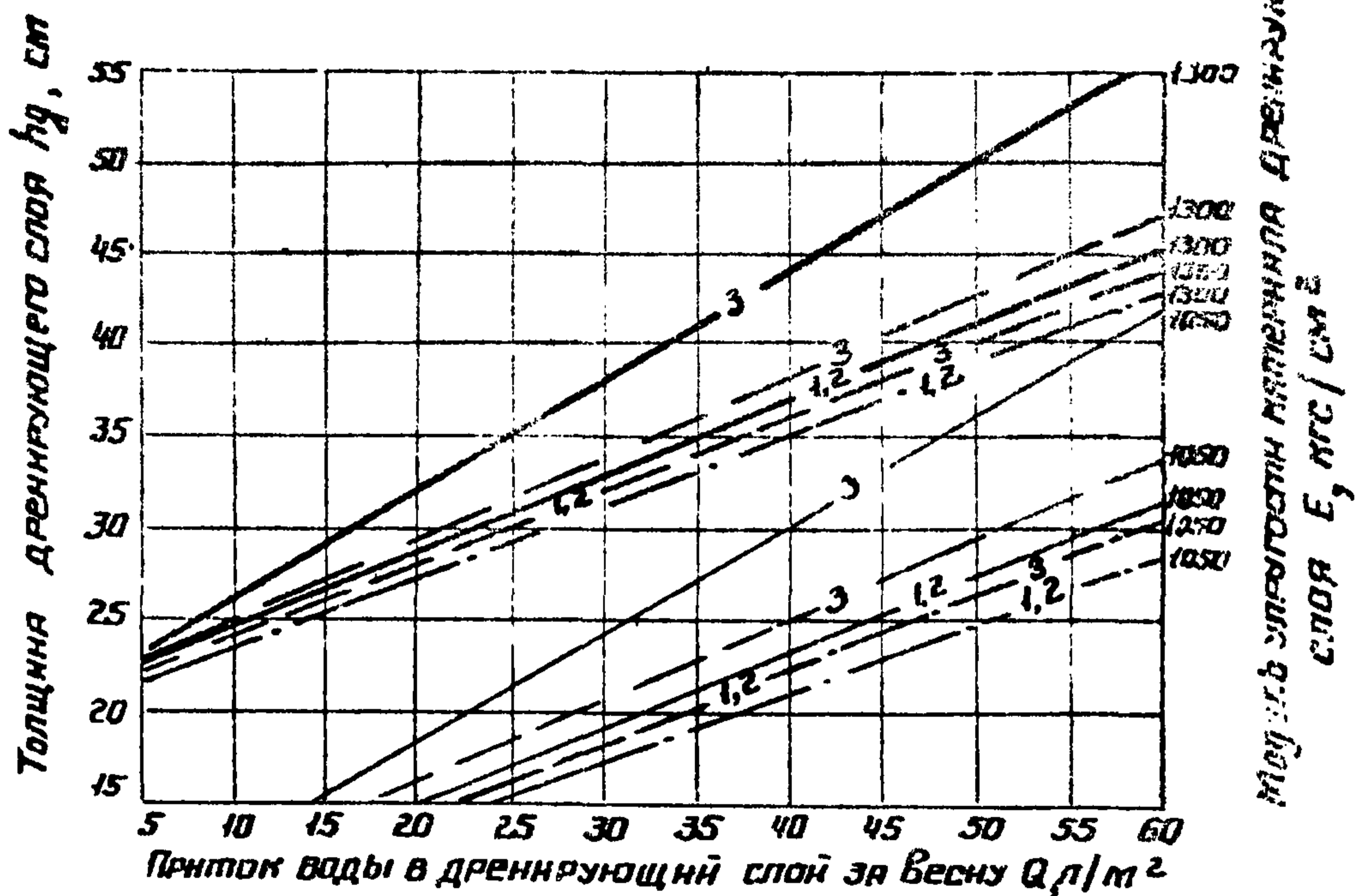
Рис. 4 График для определения толщины дренажного слоя основания h_d из песка средней крупности при поперечном профиле проезжей части с индексом Б
