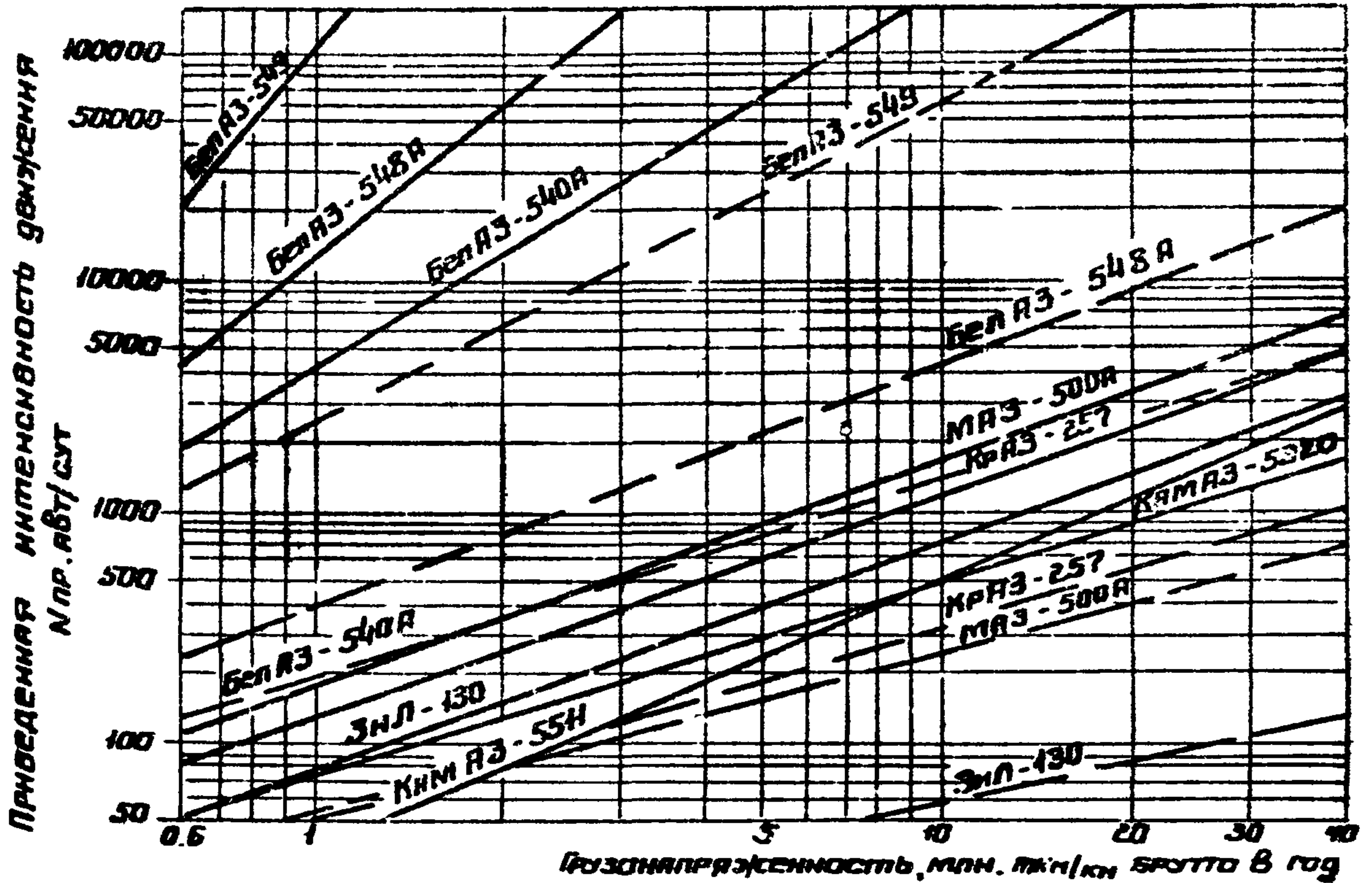
Рис. 28 Номограмма для определения приведенной интенсивности движения к расчетному автомобилю группы А
