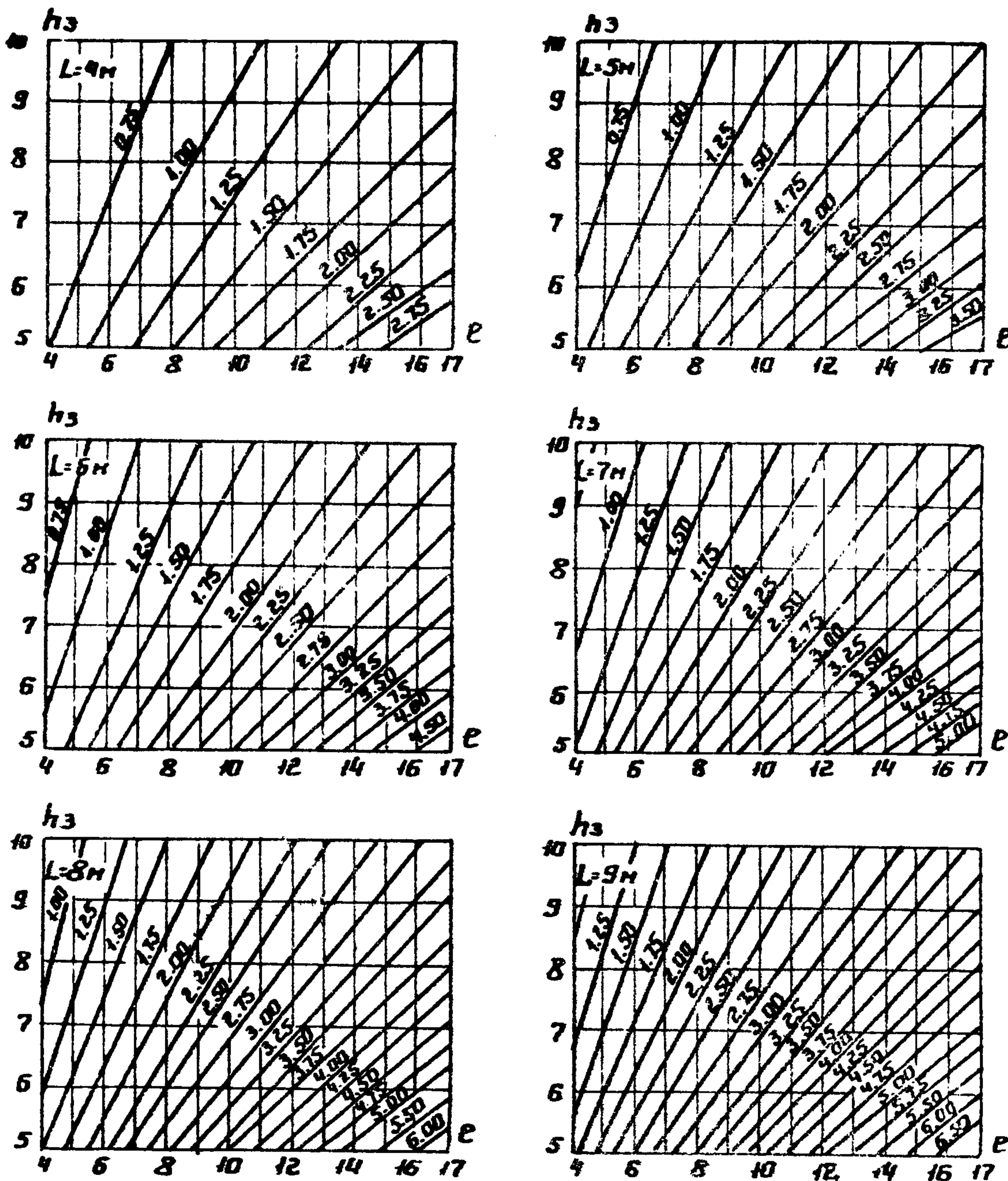
Рис. 27 Графики для определения расстояния между трубчатыми воронками (поперечный профиль дорожной одежды с индексом 8)
