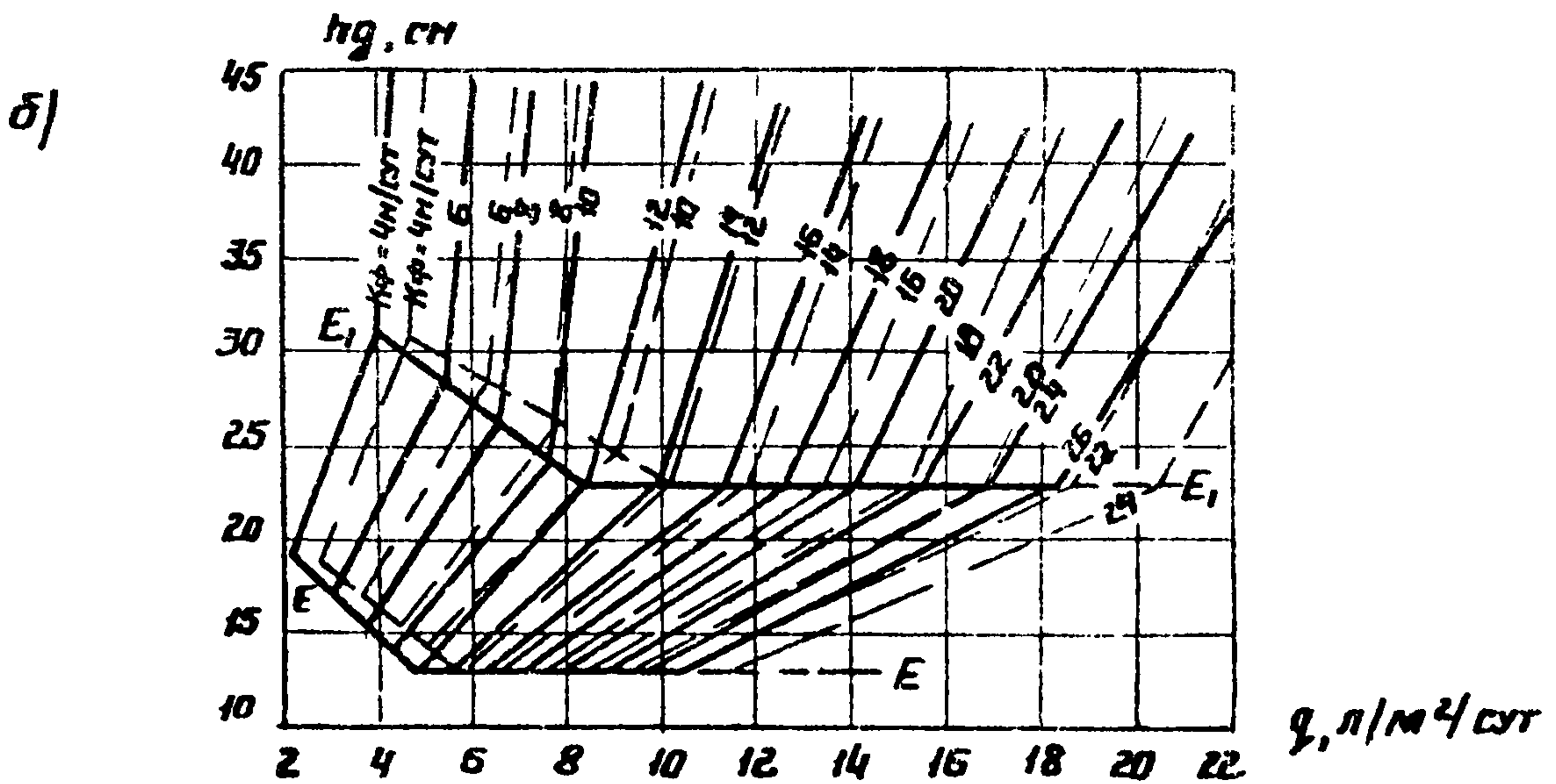
Рис. 25 График для определения толщины дренарующего слоя при поперечном профиле дорожной одежды с индексом Дн пути фильтрации 100
