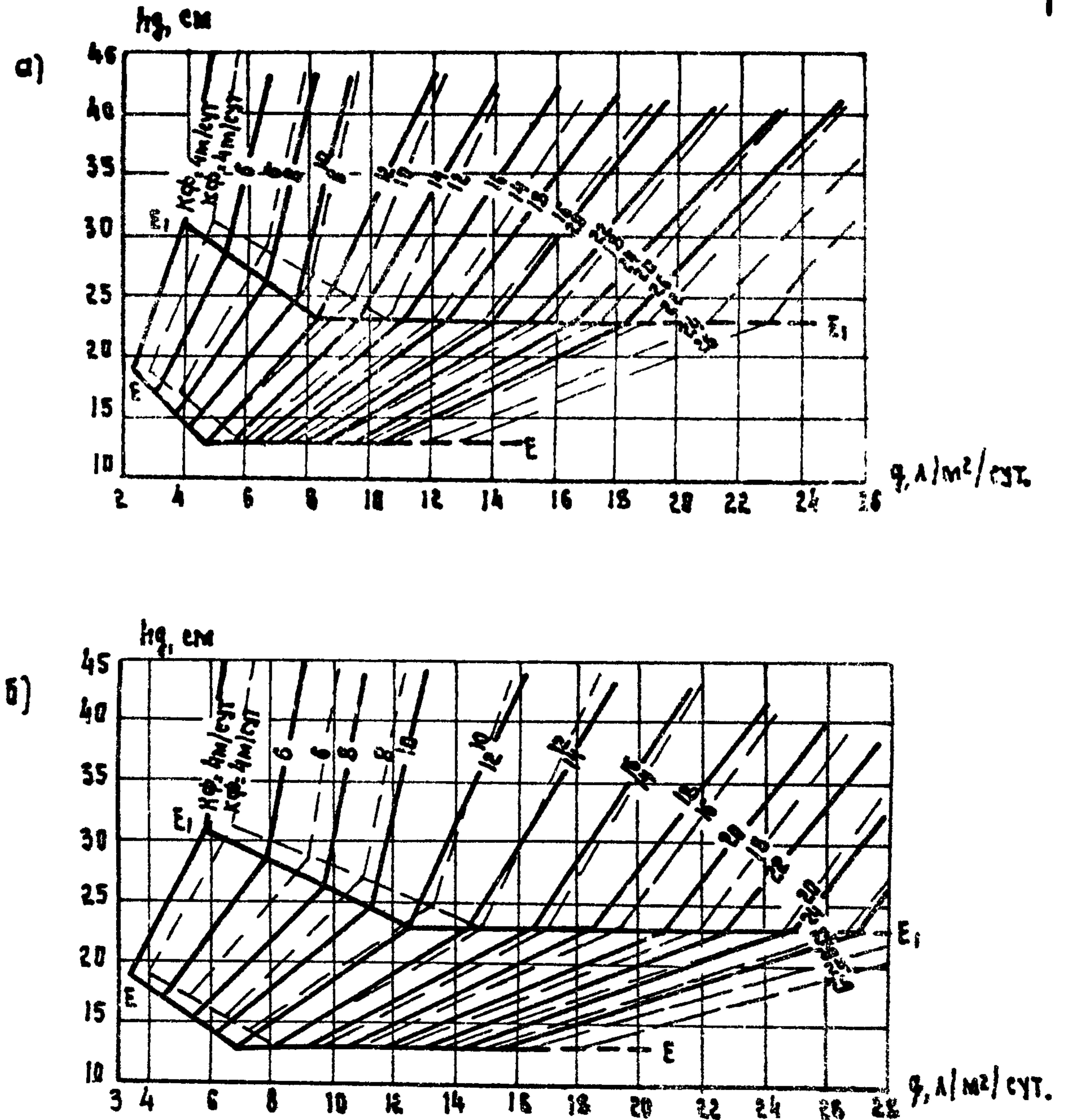
Рис. 22 График для определения толщины дренарующего слоя при поперечном профиле дорожной одежды с индексом \Delta и пути фильтрации h_m .
