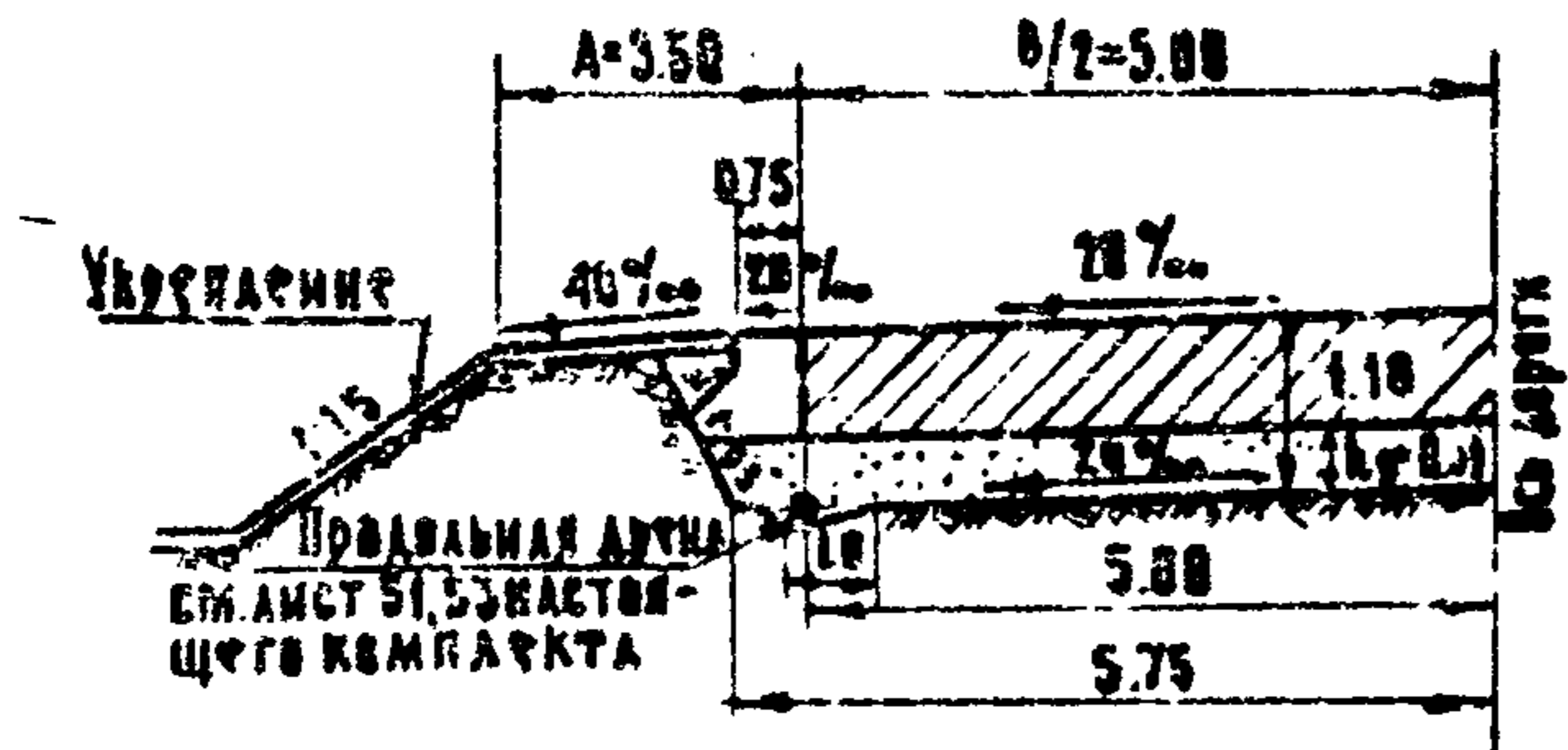
ВЫЕМКА ПРИ ПРОДАЛЬНОМ УКЛОНЕ ДО 40%
