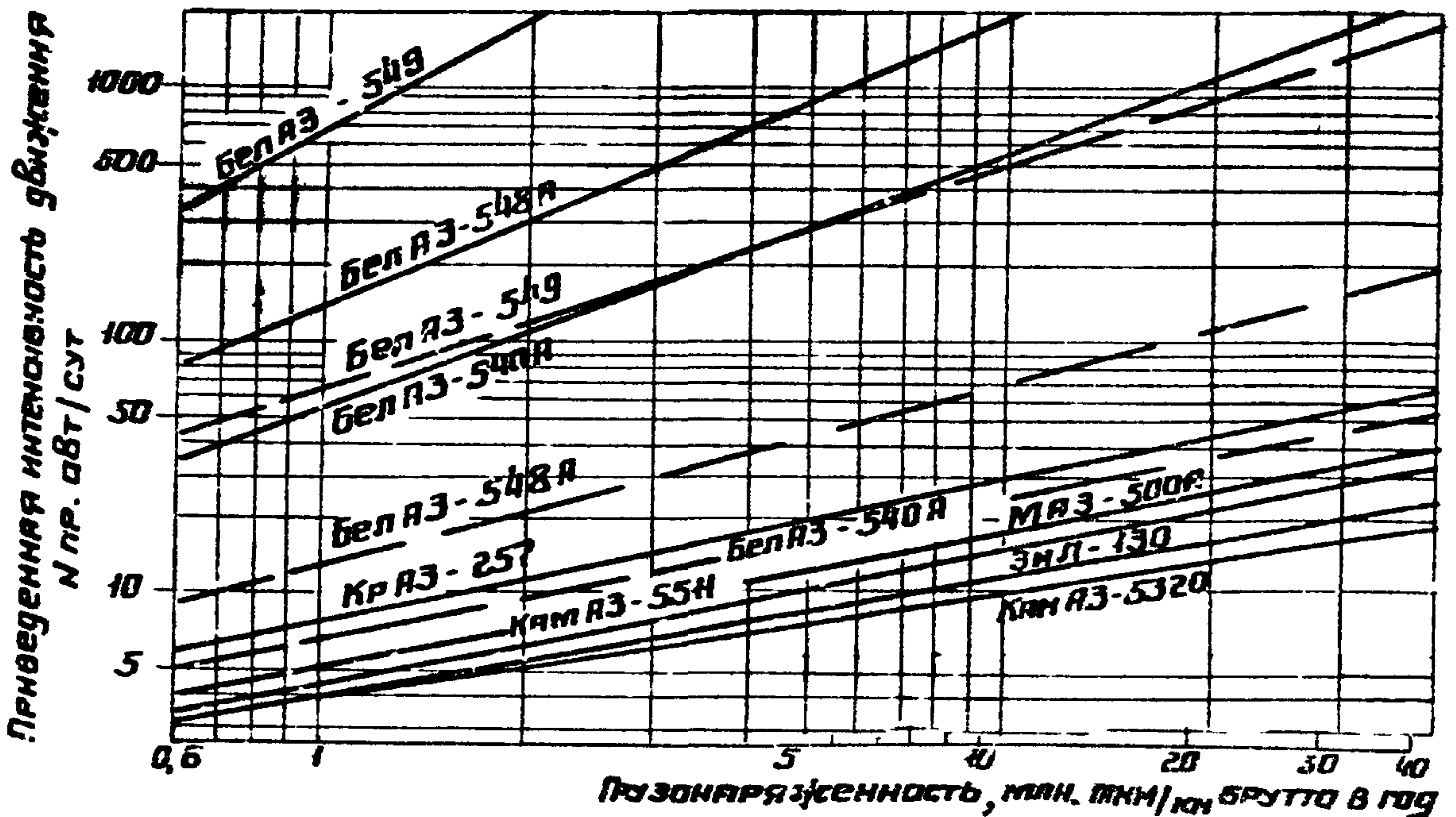
Рис. 29 Номограмма для определения интенсивности движения к расчетному автомобилю БелАЗ - 540
