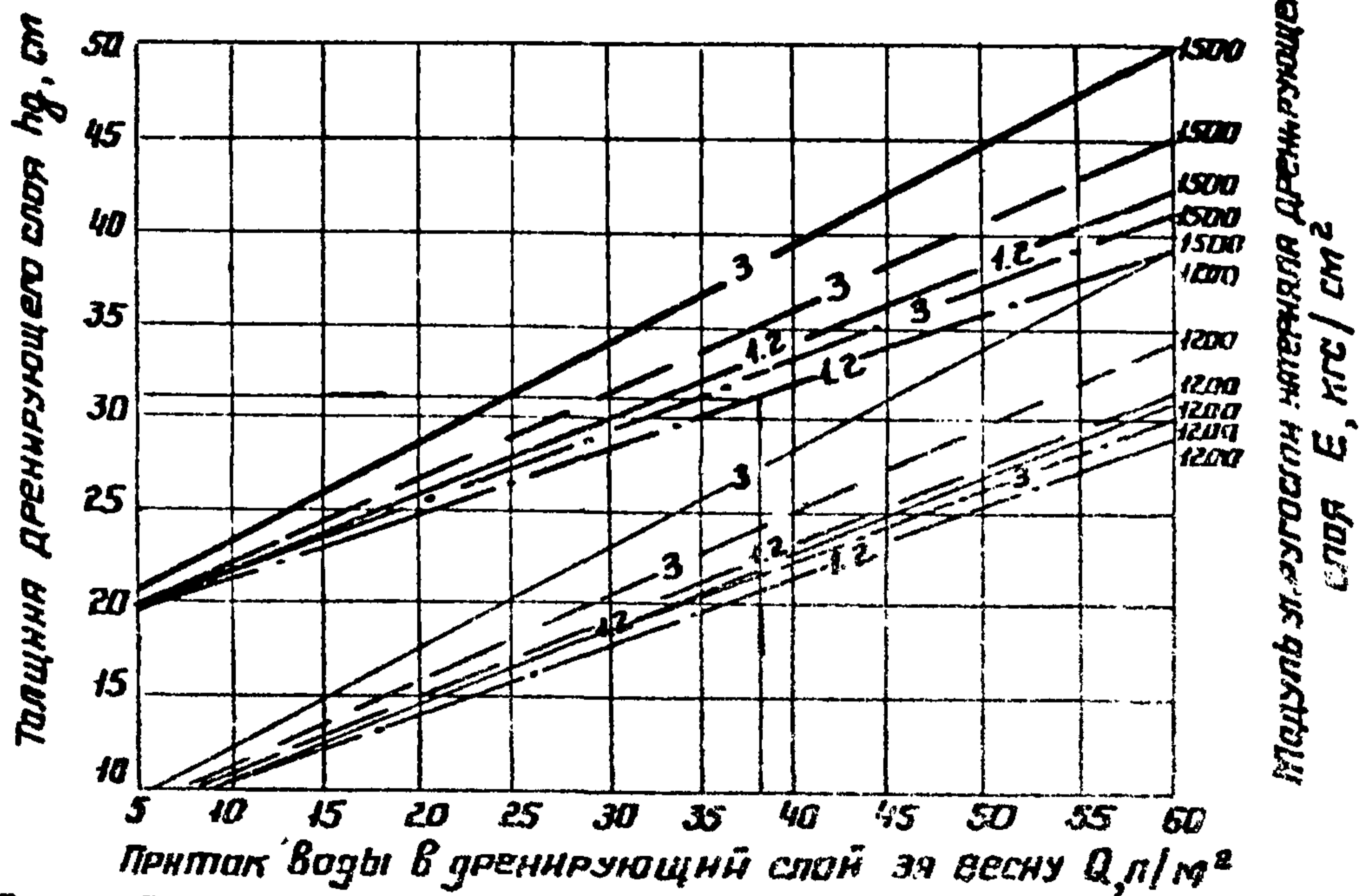
Рис. 5 График для определения толщины дренажного слоя основания h_d из крупного песка при поперечном профиле проезжей части с индексом Б
