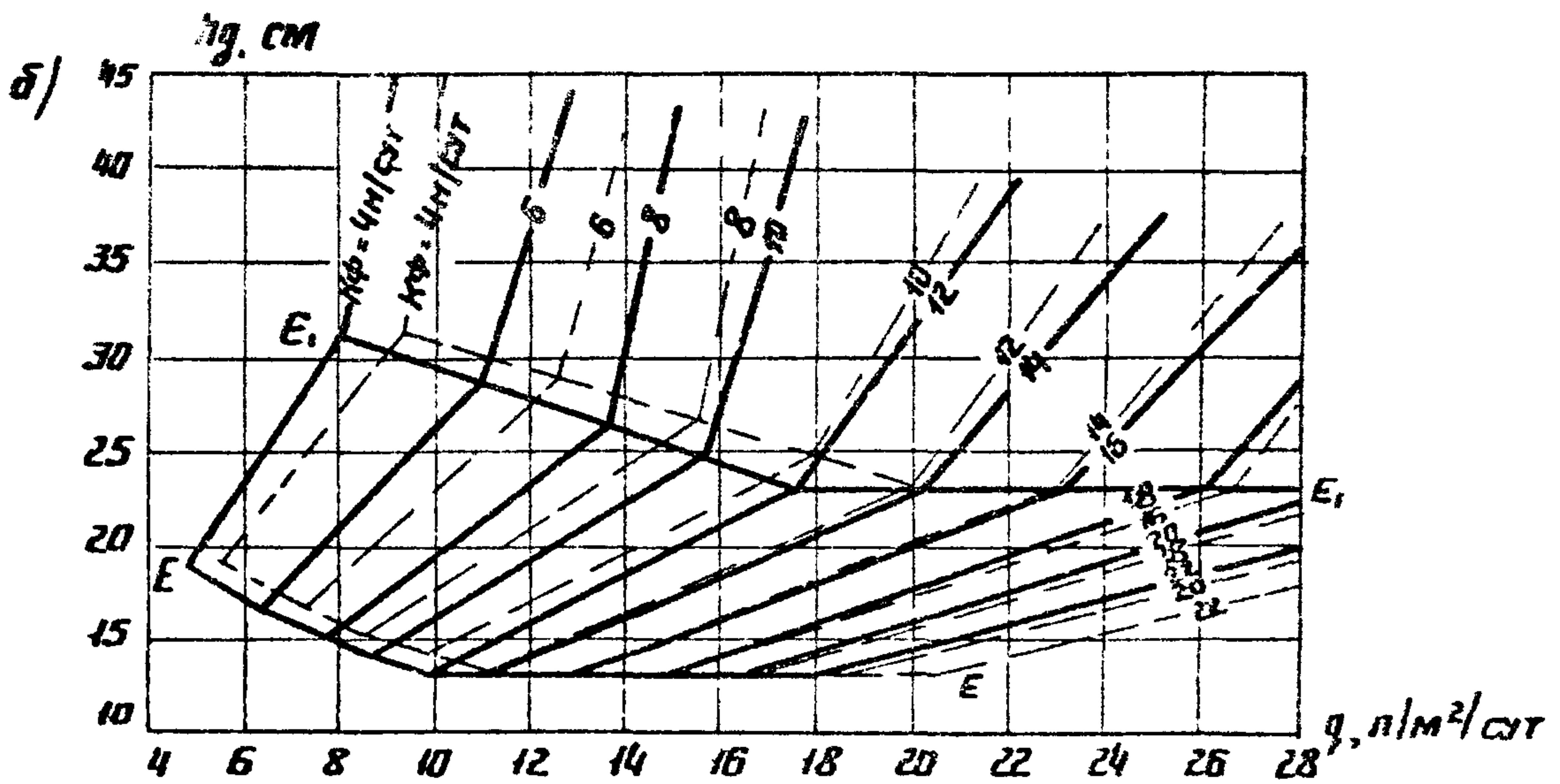
Рис. 20 График для определения толщины дренажного слоя при поперечном профиле дорожной одежды с индексом D_n пути фильтрации 9 м.
