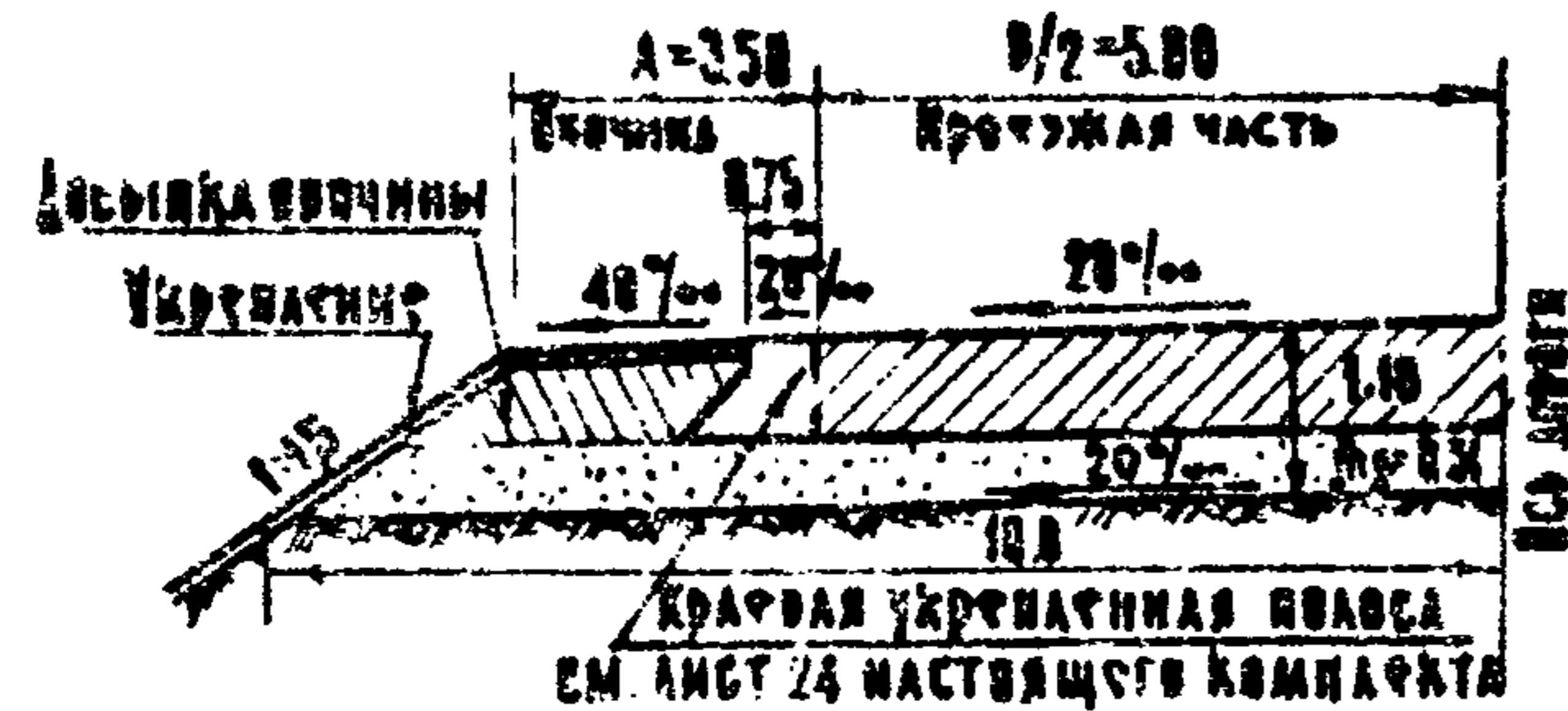
НАСЫПЬ ПРИ ПРОДАЛЬНОМ УКЛОНЕ ДО 40%
