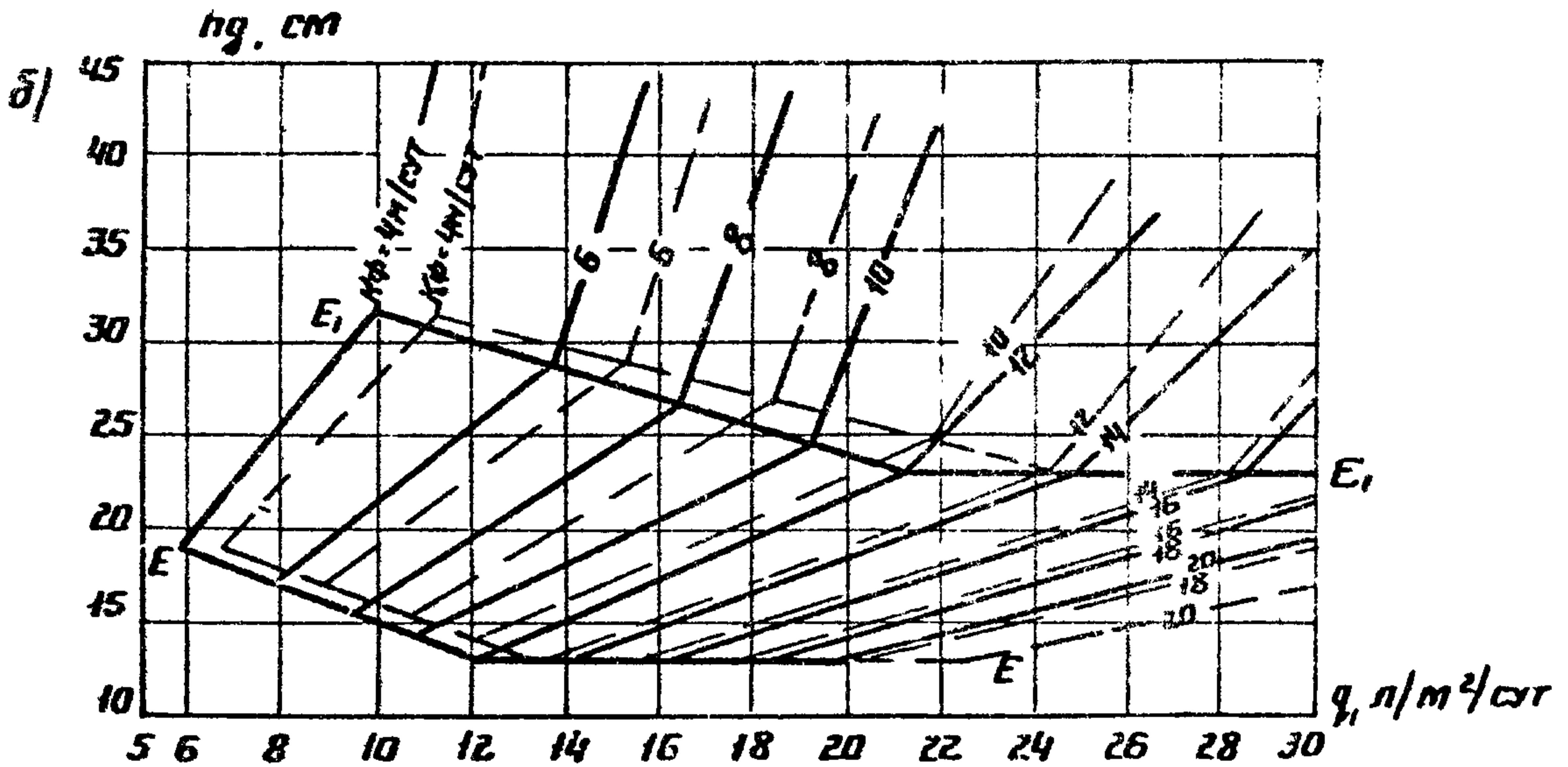
Рис. 19 График для определения толщины дренажного слоя при поперечном профиле дорожной одежды с индексом D и пути фильтрации 8 м.
