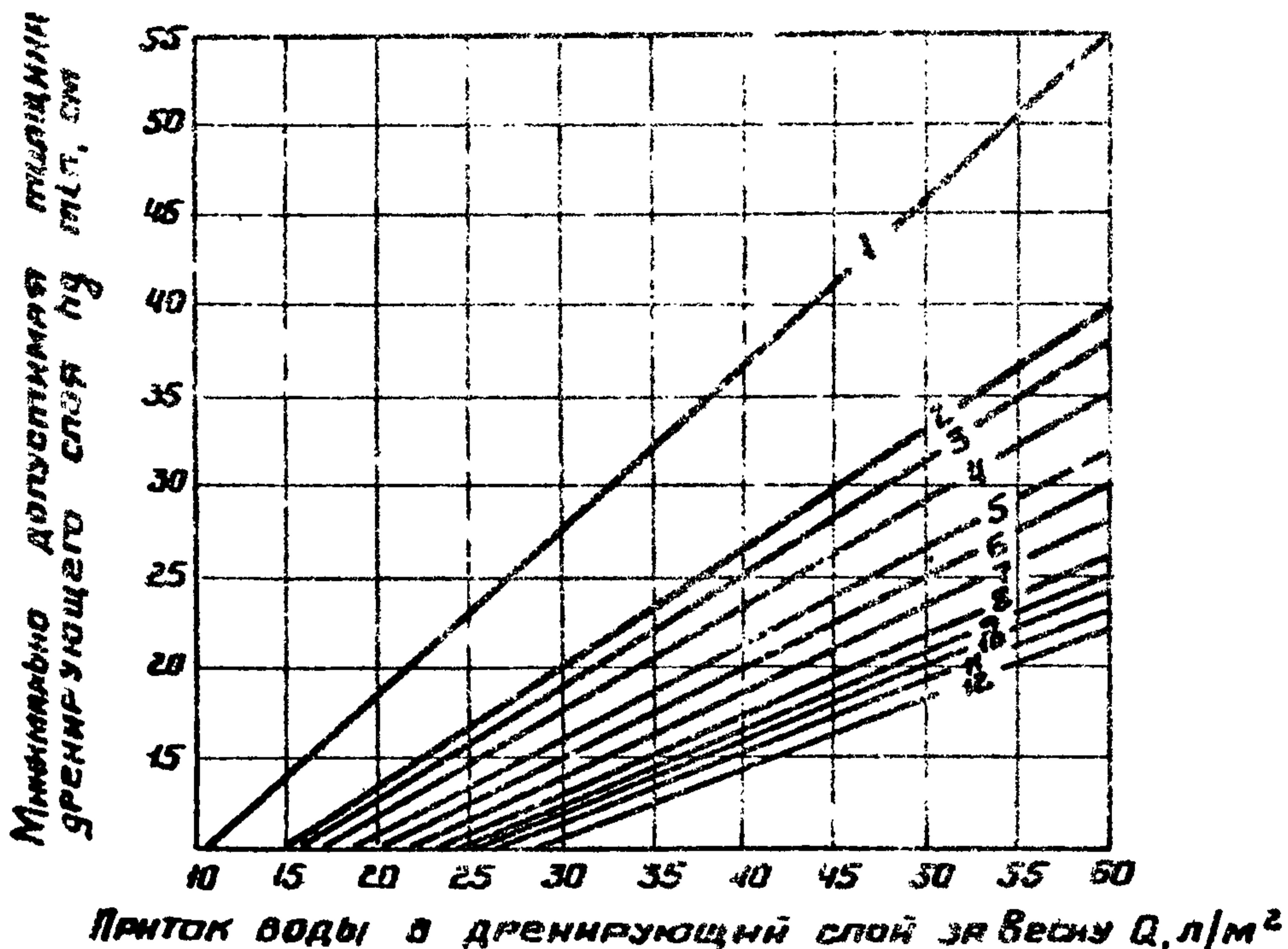
Рис. 6 График для определения толщины дренающего слоя основания h_d при поперечном профиле проезжей части с индексом Б и переходном типе дорожной одежды
