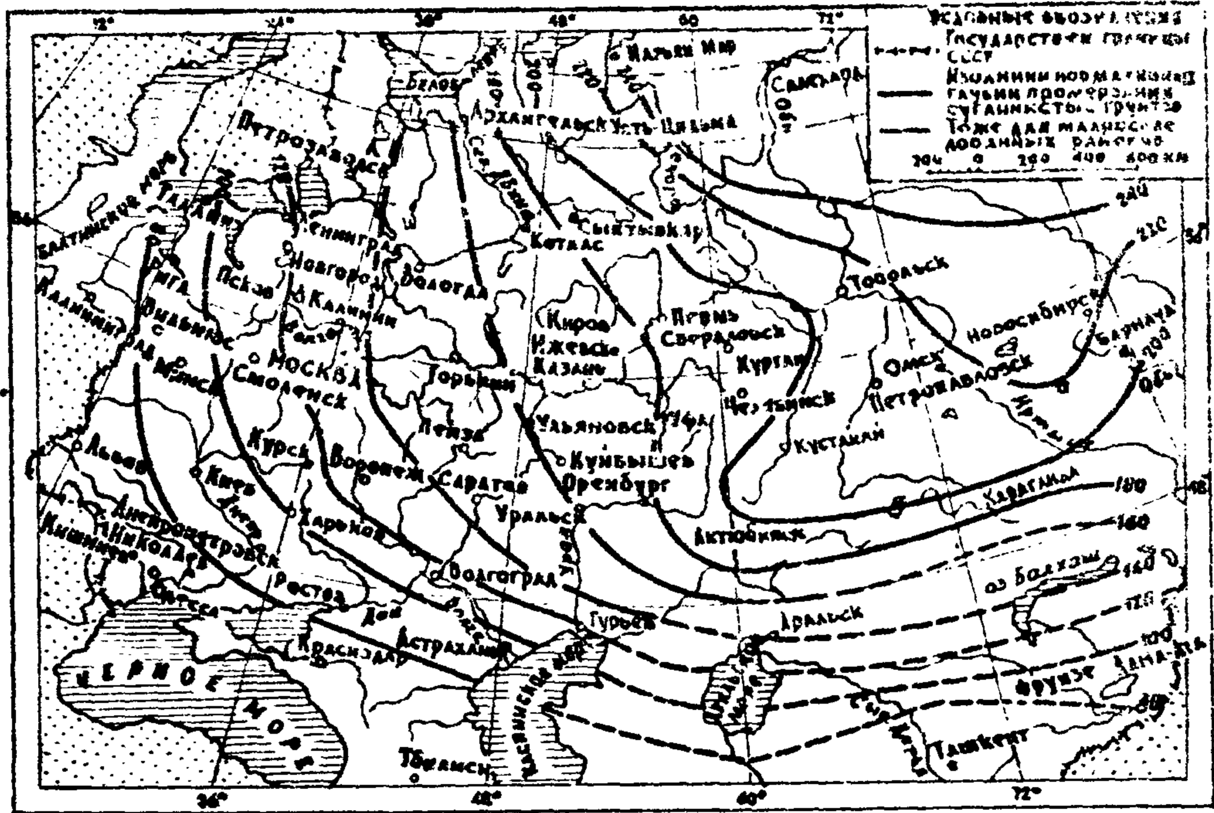
Рис. 37 Карта изотерм глубин наибольшего промерзания грунтов
