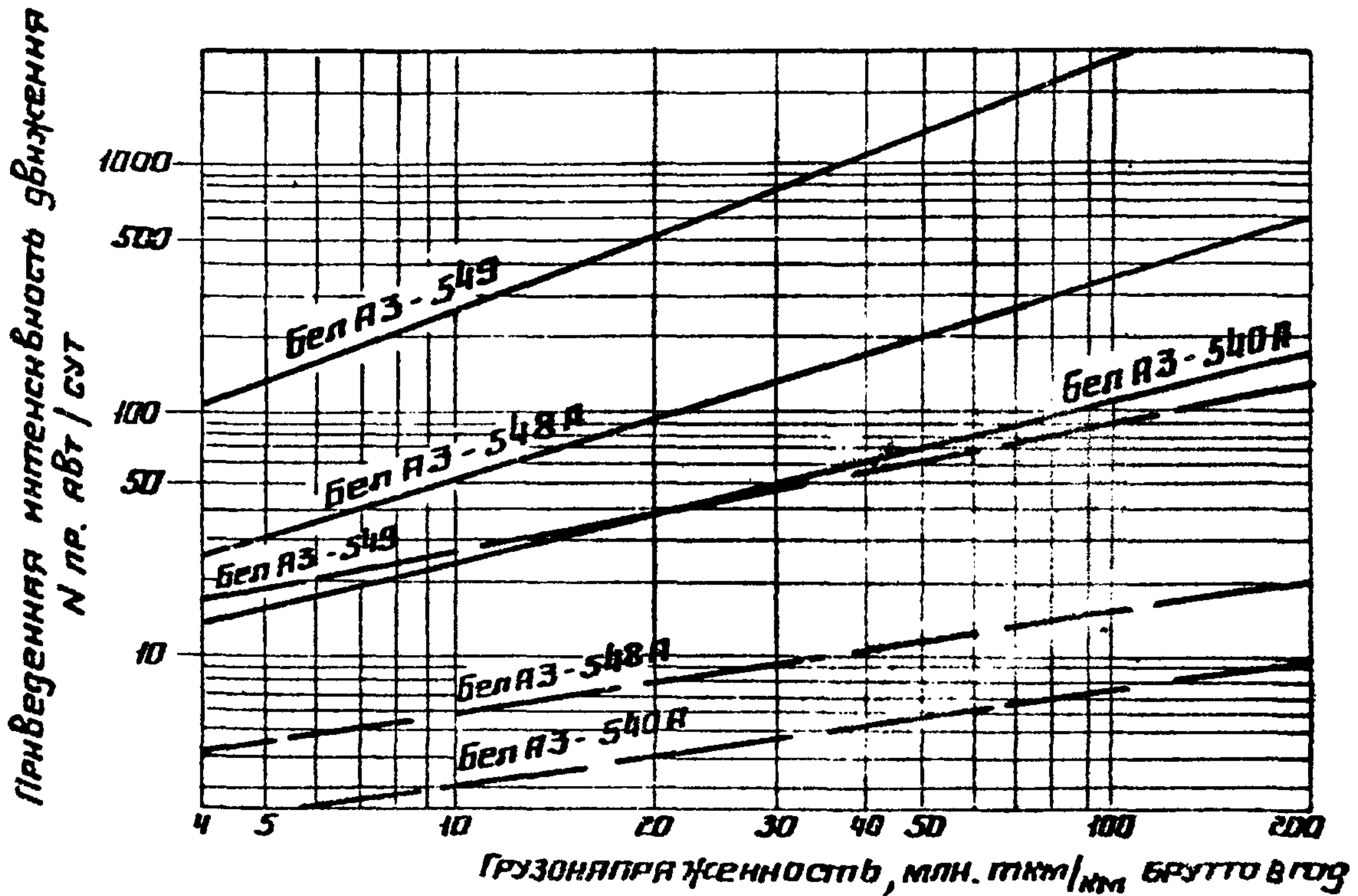
Рис 31 Номограмма для определения приведенной интенсивности движения к расчетному автомобилю БелАЗ-549. Обозначения те же, что и на Рис. 28
