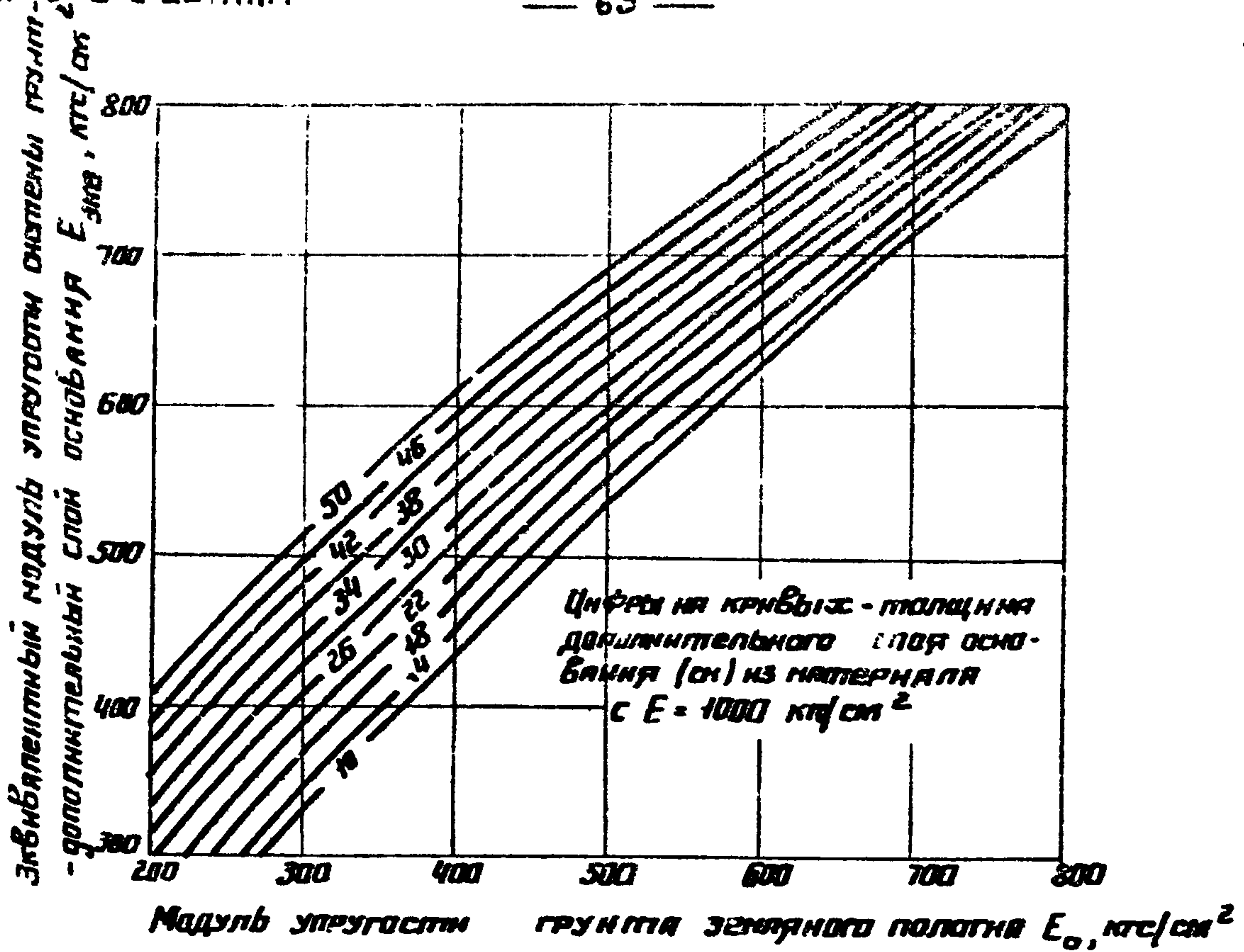
Рис. 35 Нограмма для определения эквивалентного модуля упругости системы грунт-дополнительный слой основания при расчетном автомобиле БелАЗ-548
