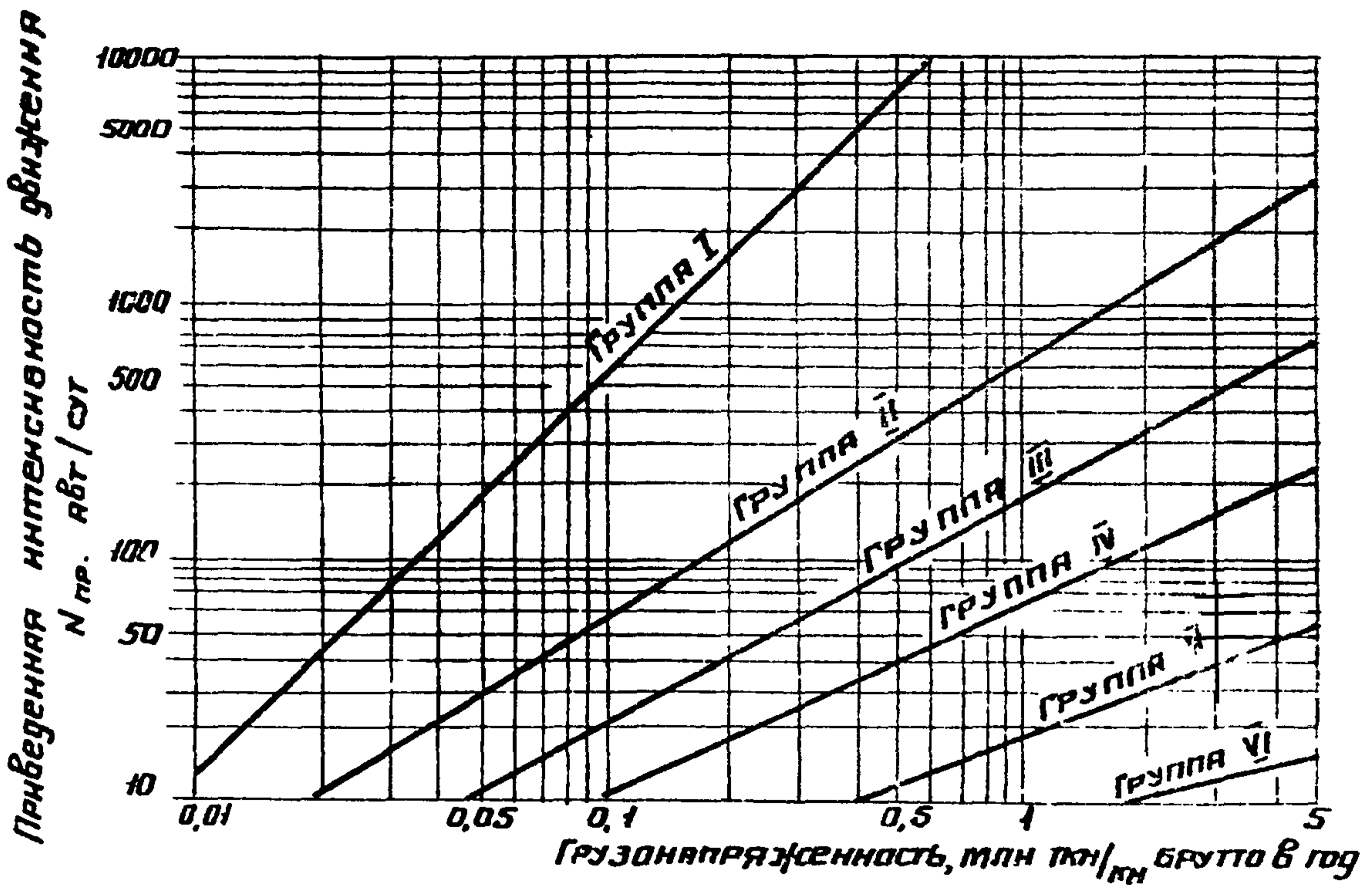
Рис. 32 Номотранна для определения приведенной интенсивности движения погрузчиков и тележек к расчетному автомобилю группы А.
