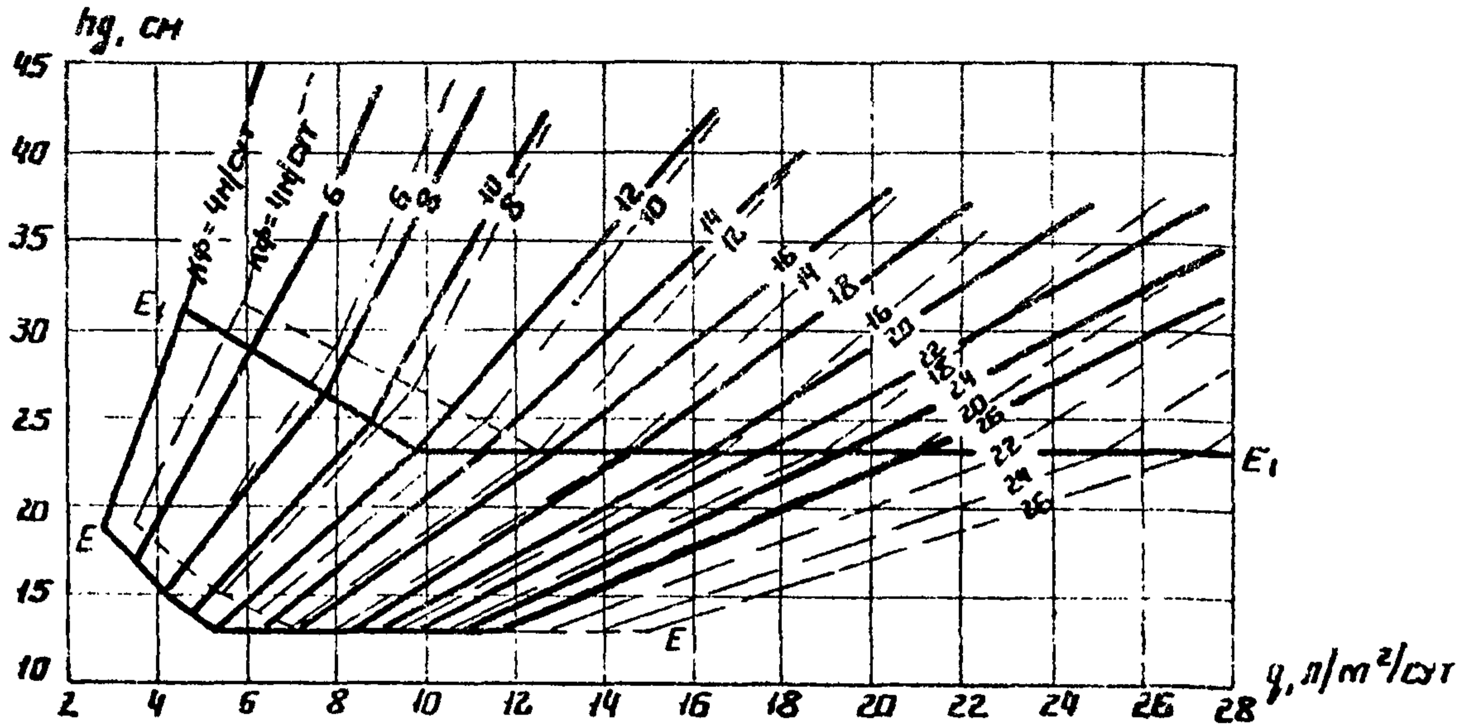
Рис. 11 График для определения толщины дренажного слоя при поперечном профиле дорожной одежды с индексом В и Г и пути фильтрации 8 м. Обозначения те же, что и на рис. 7.
