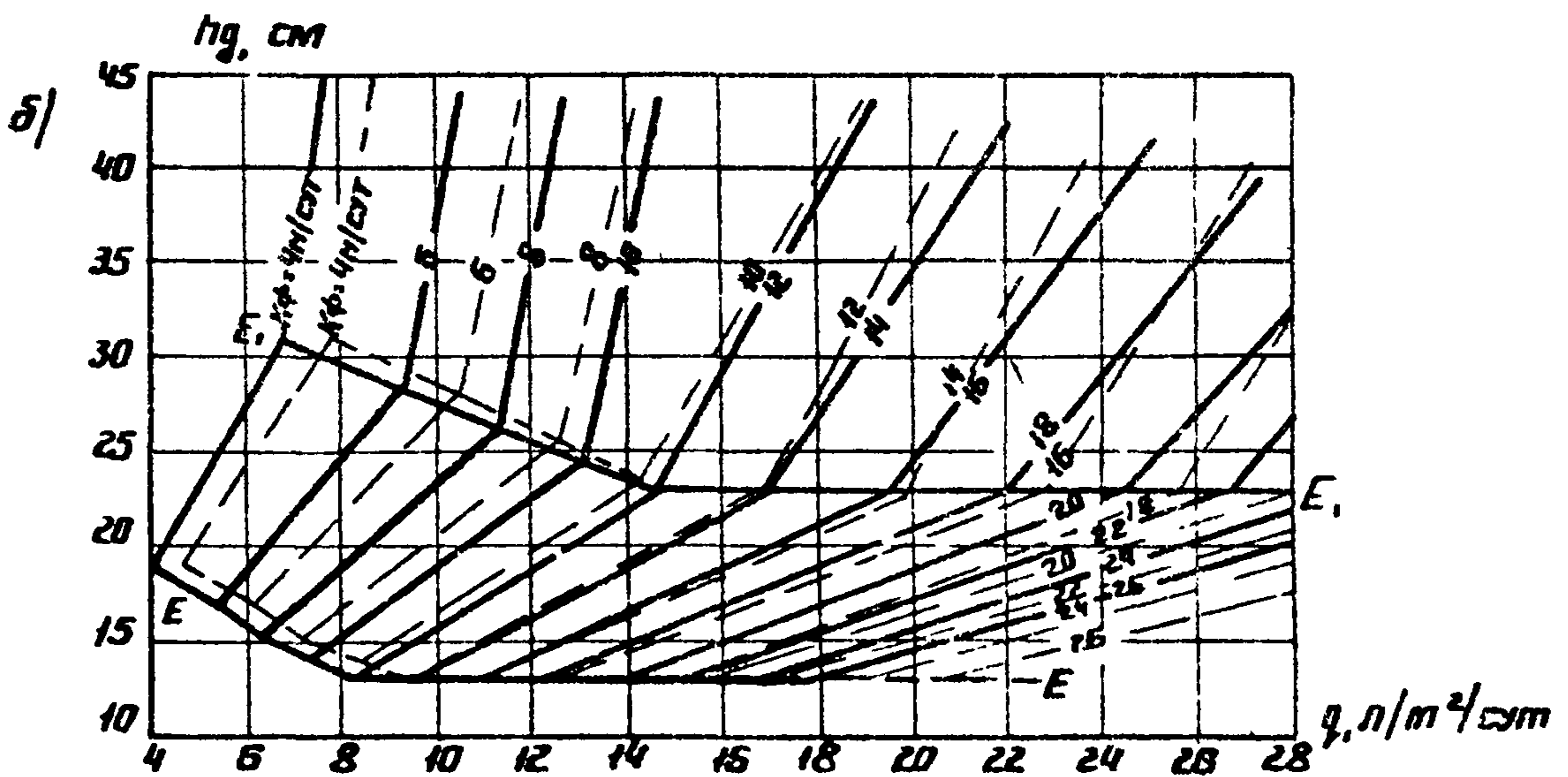
Рис. 21 График для определения толщины дренающего слоя при поперечном профиле дорожной колеи с индексом D и пзтм, фильтрации 10M а - Глубина ровика 25 см; б - Глубина ровика 45 см. Обозначения те же, что и на рис. 7
