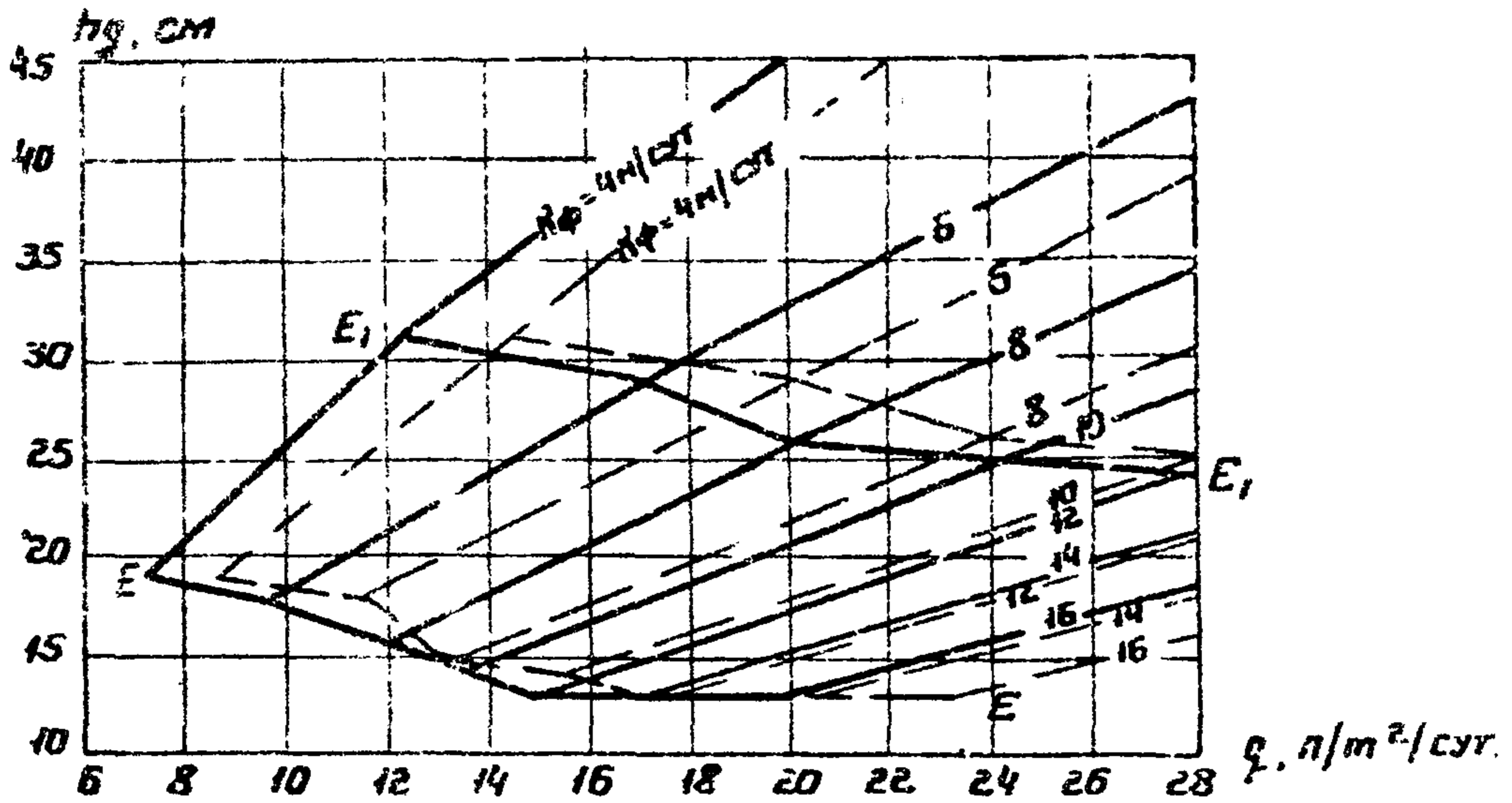
Рис. 7 График для определения толщины дренажного слоя при поперечном профиле дорожной одежды с индексами В и Г и пути фильтрации 4 м
