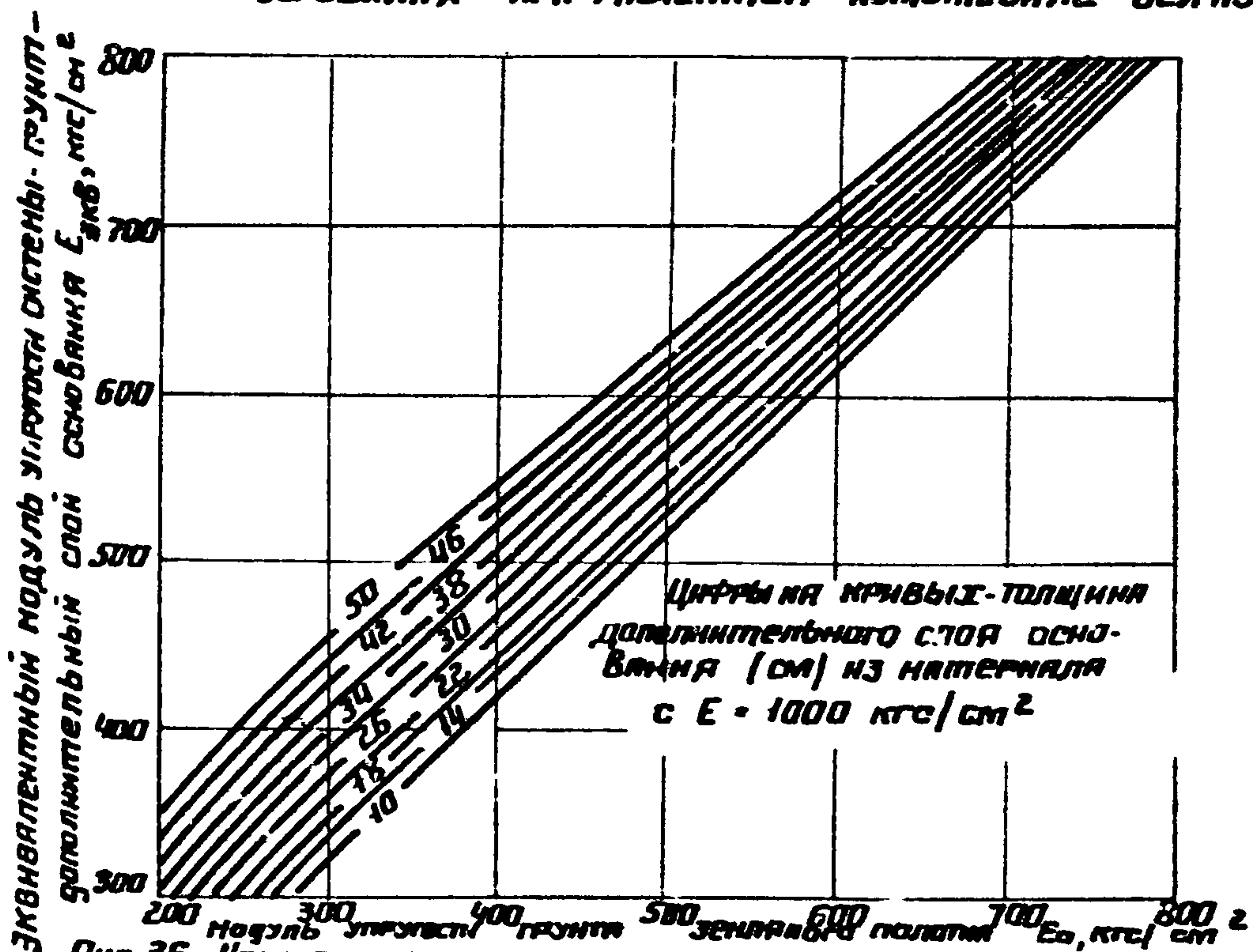
Рис. 36 Нограмма для определения эквивалентного модуля упругости системы грунт-дополнительный слой основания при расчетном автомобиле БелАЗ-549
