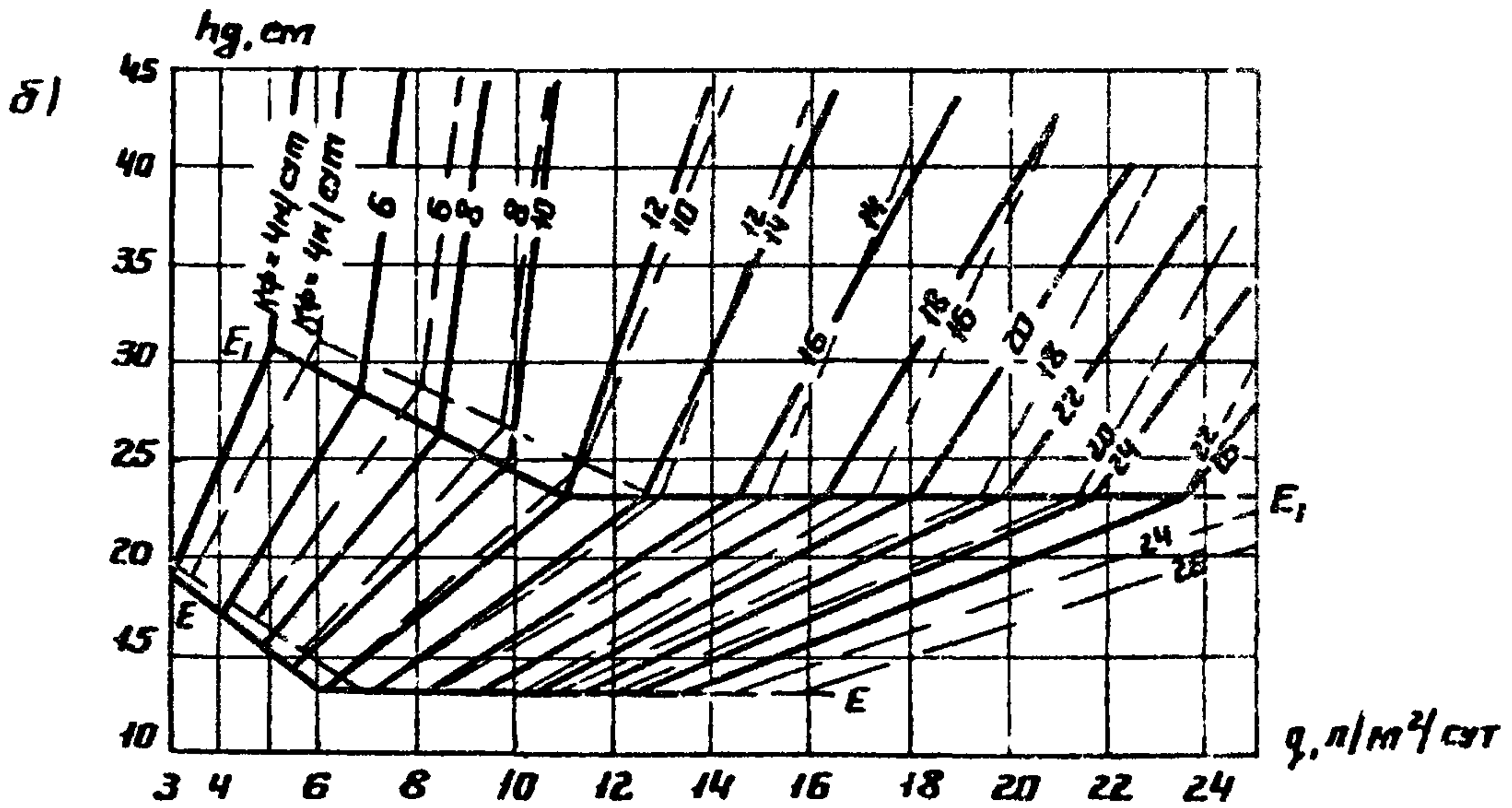
Рис 23 График для определения толщины дренарующего слоя при поперечном профиле дорожной одежды с индексом D_n пути фильтрации 12 м а - глубина ровика 25 см; б - глубина ровика 45 см. Обозначения те же, что и на рис. 7
