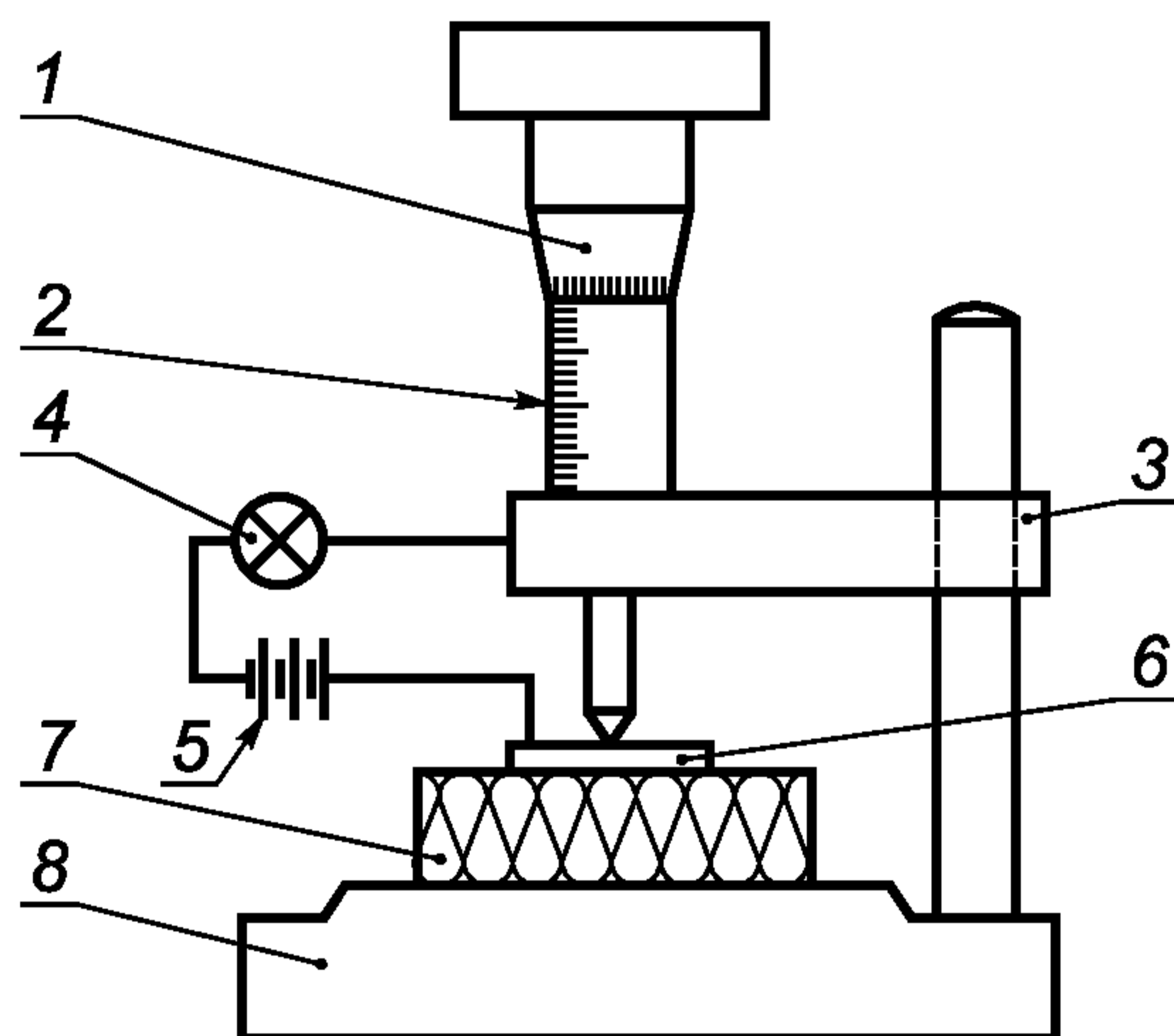
1 — винтовой микрометр; 2 — шкала с делениями в миллиметрах; 3 — регулируемая опора; 4 — лампа; 5 — батарея; 6 — алюминиевая пластина площадью 10 \text{ см}^2 ; 7 — образец для измерения; 8 — основание
