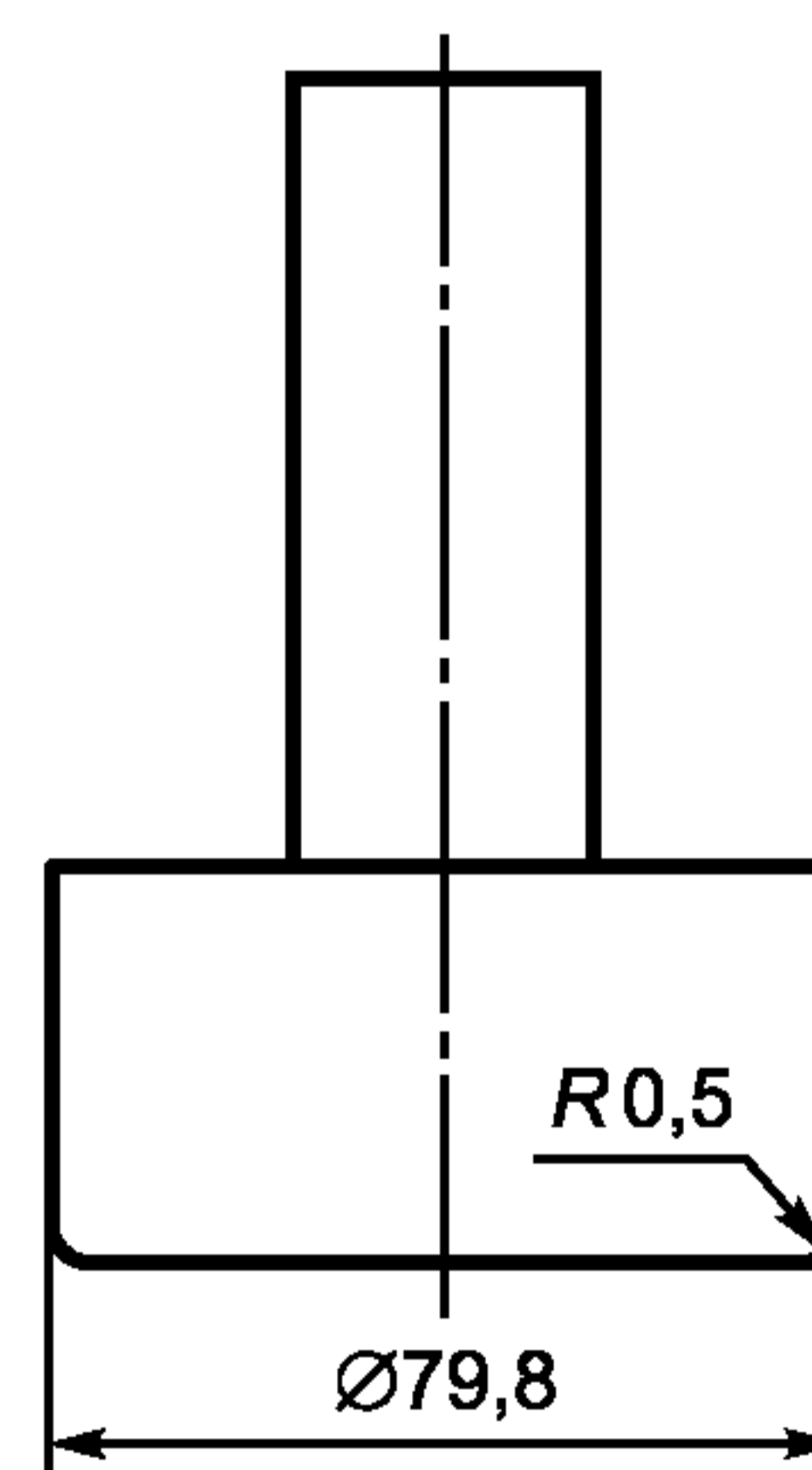
Рисунок 3 — Цилиндрический индентор
