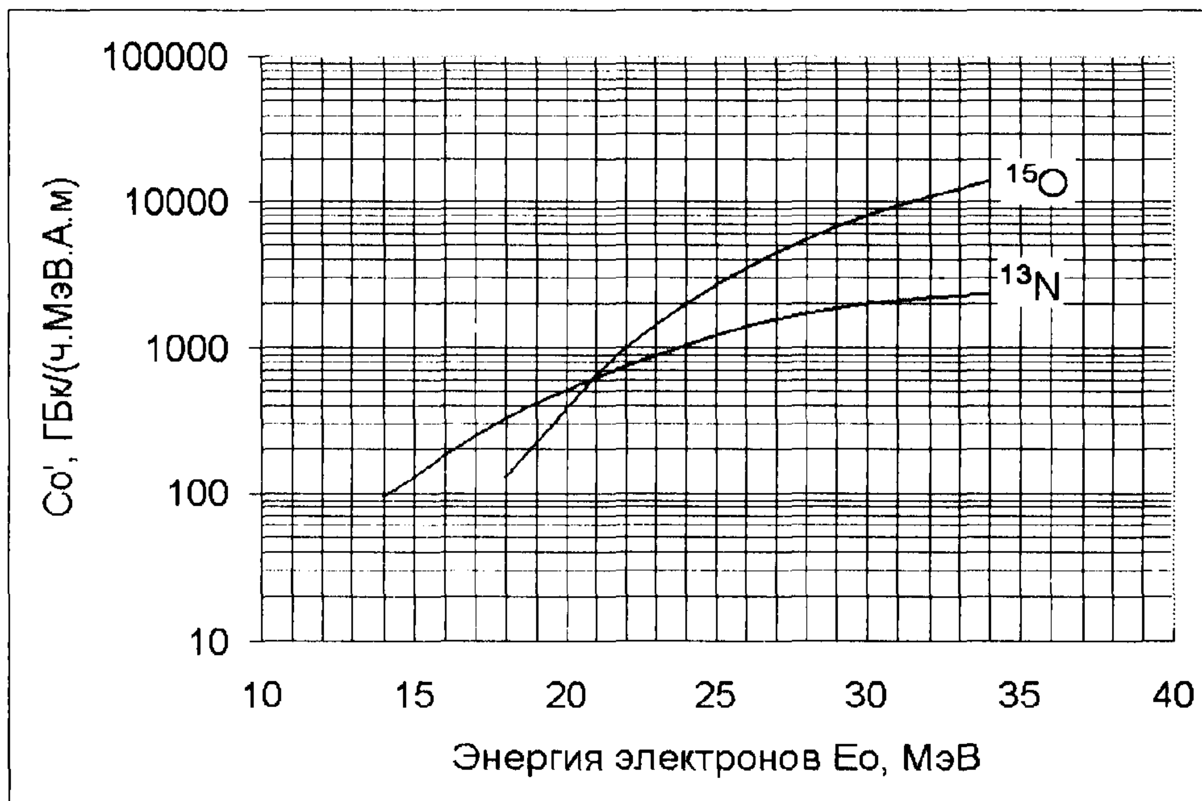
Рис. 1. Зависимость постоянной скорости образования ( C'_0 ) радионуклидов ^{13}\text{N} и ^{15}\text{O} от энергии электронов (вольфрамовая мишень)
