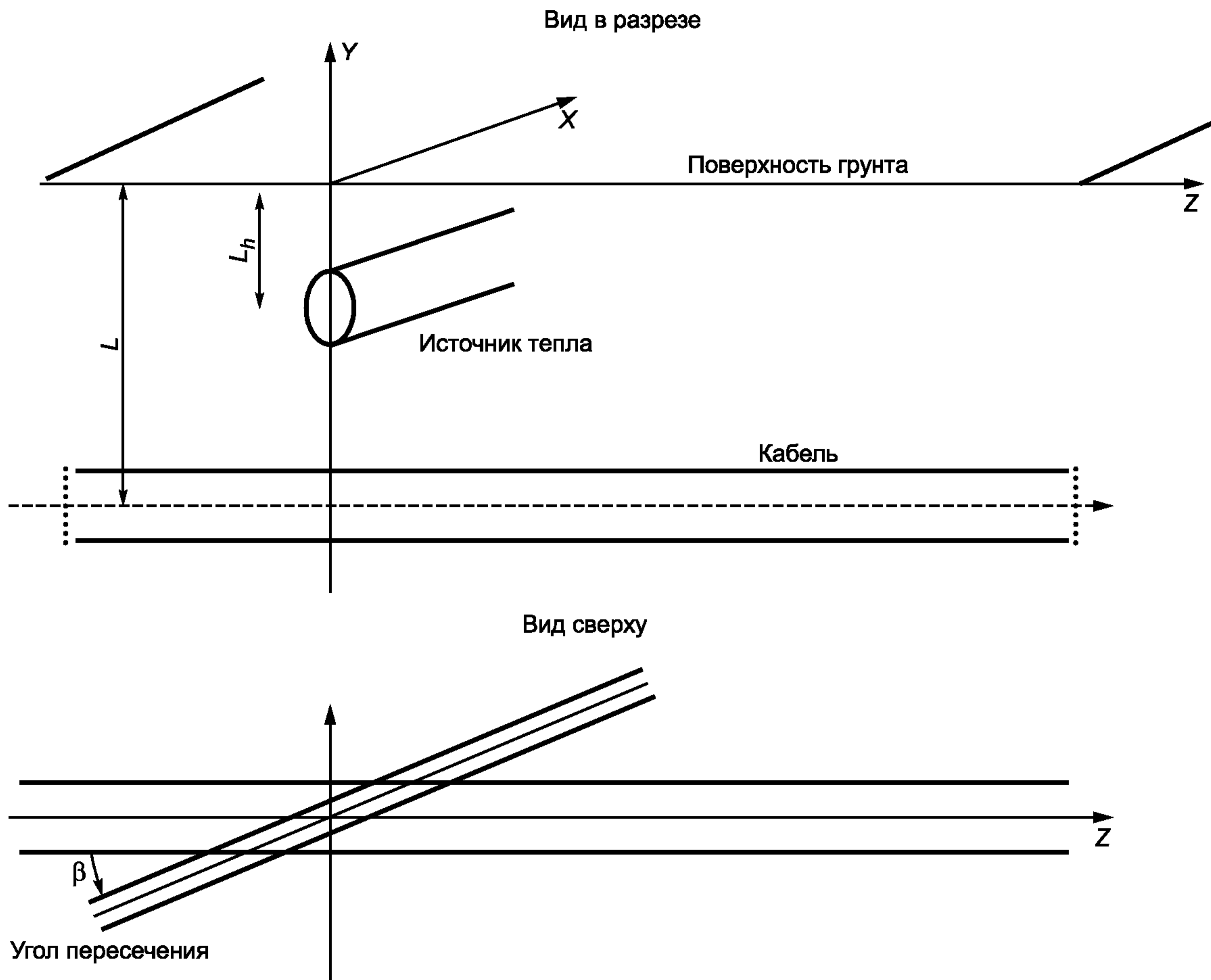
Рисунок 1 — Пример расположения источника тепла, пересекающего рассматриваемый кабель
