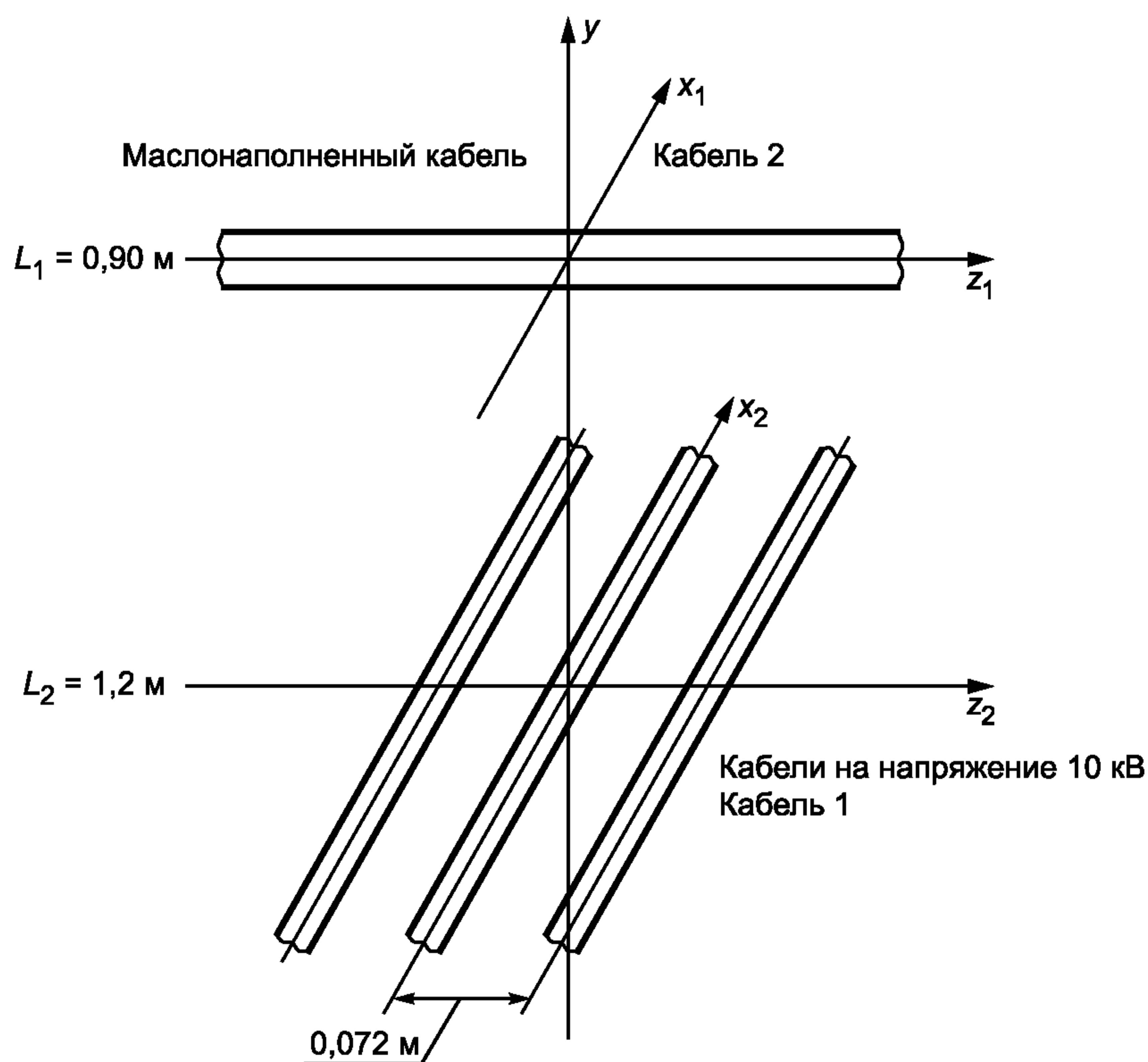
Рисунок А.1 — Расположение кабелей
