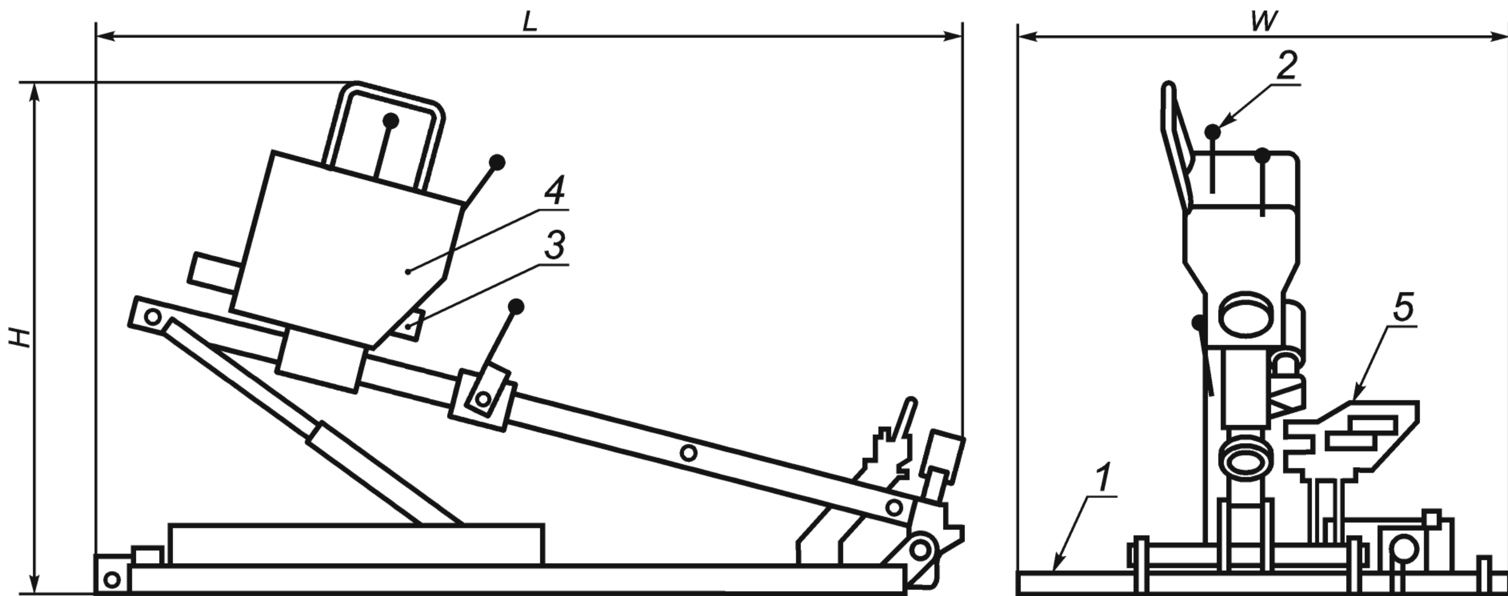
H — общая высота машины; L — общая длина машины; W — общая ширина машины; 1 — место оператора; 2 — управление процессом бурения; 3 — шпindelь; 4 — каретка; 5 — зажим
