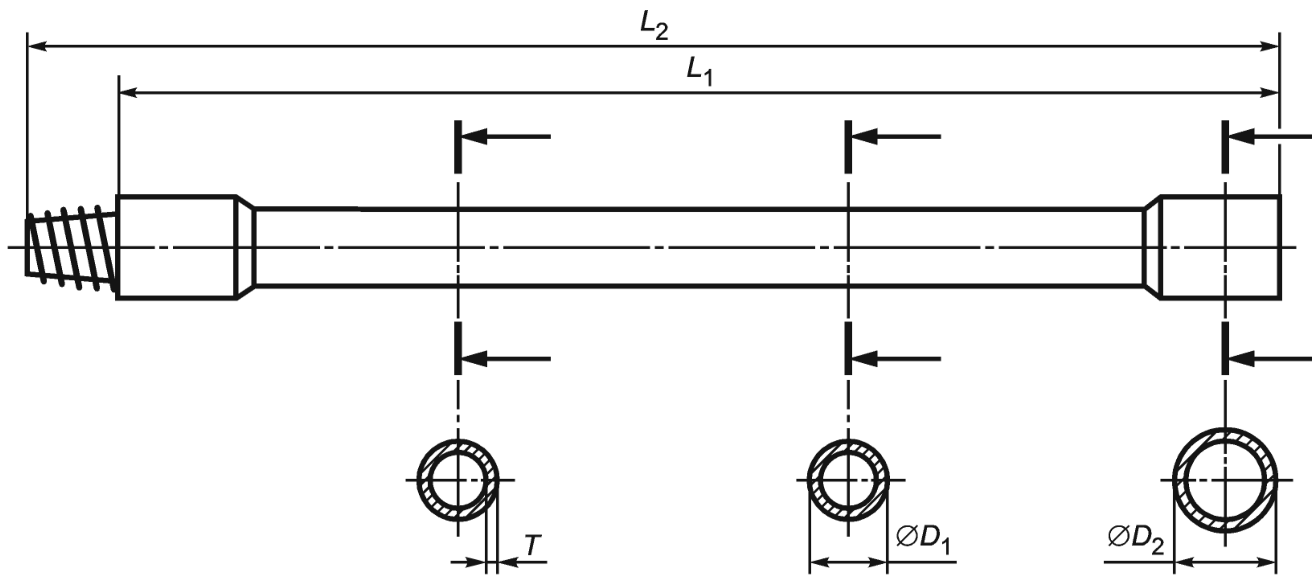
Рисунок 5 — Бурильная труба
