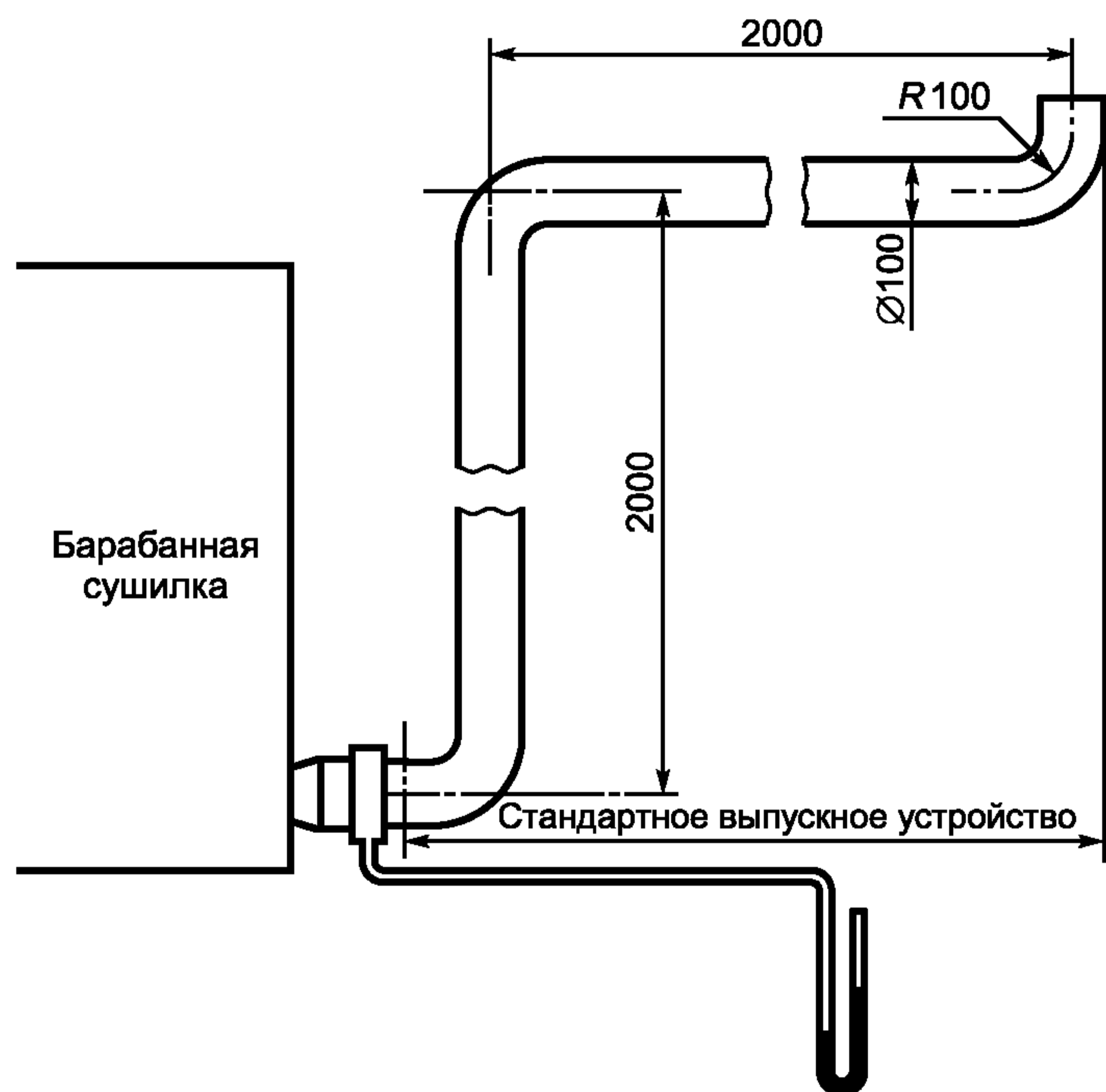
Рисунок А.1 — Стандартное выпускное устройство
