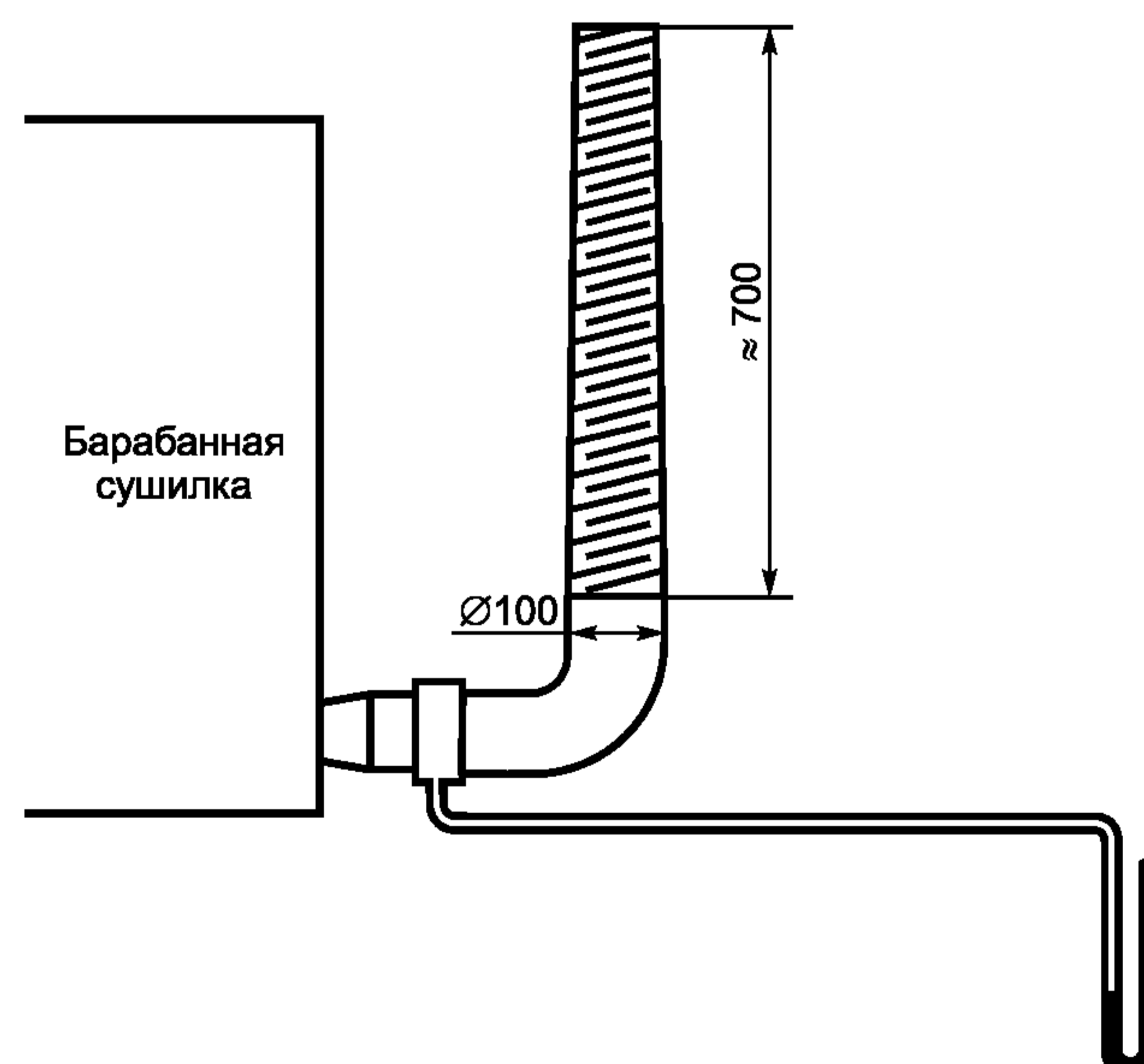
Рисунок А.2 — Стандартное выпускное имитирующее устройство
