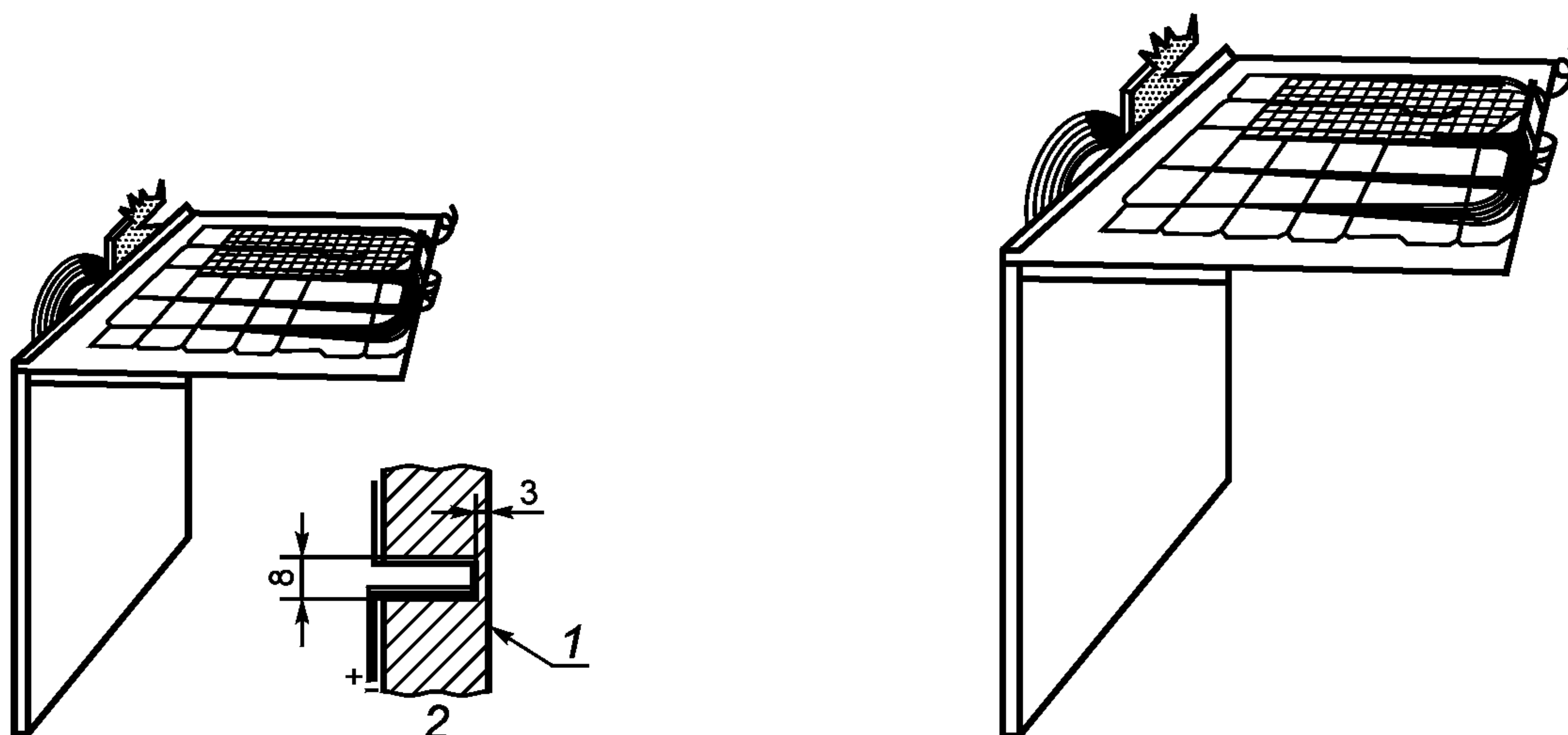
а) Расположение для испытания на агрегате, монтирующемся на стену
