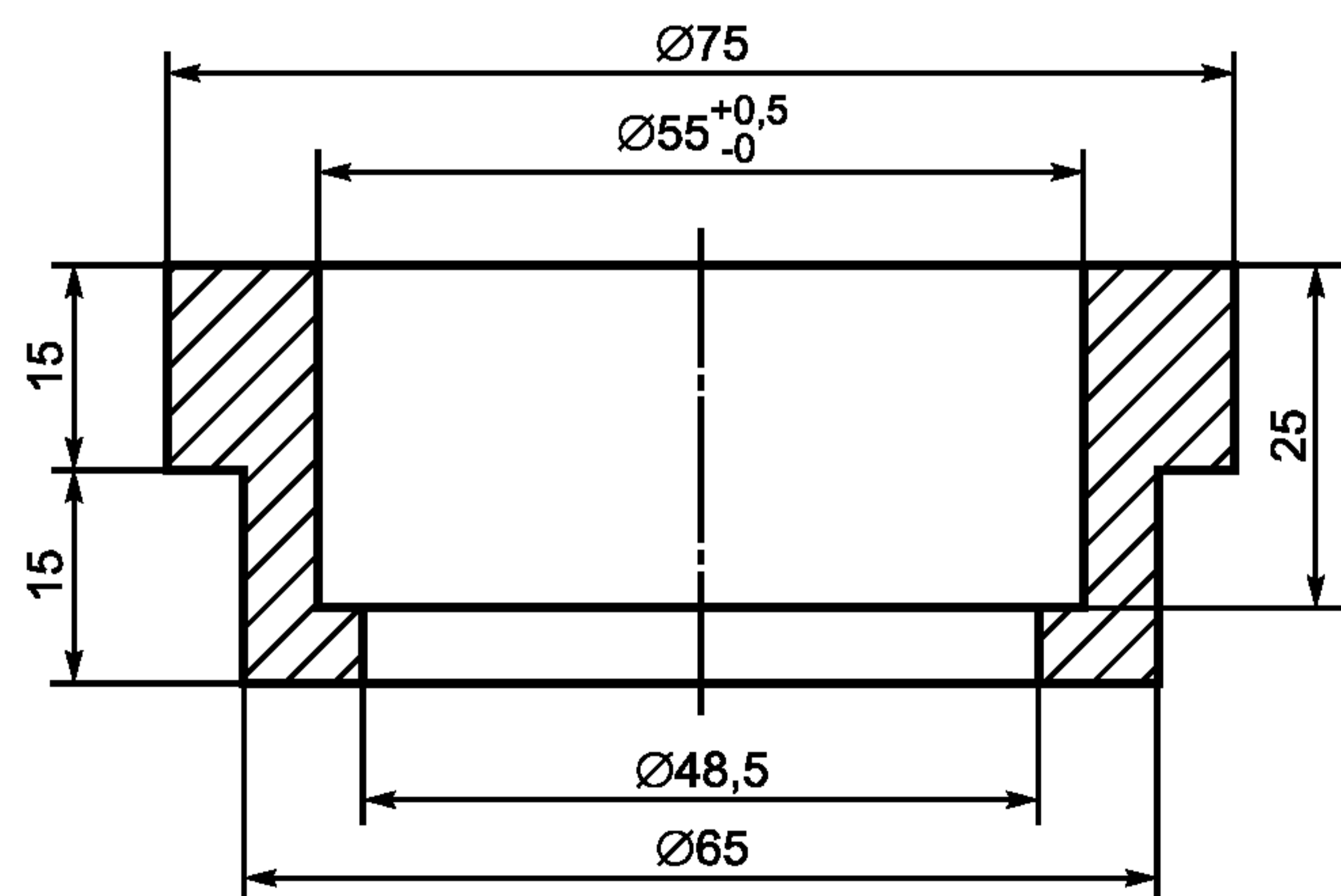
Рисунок 3 — Прокладки
