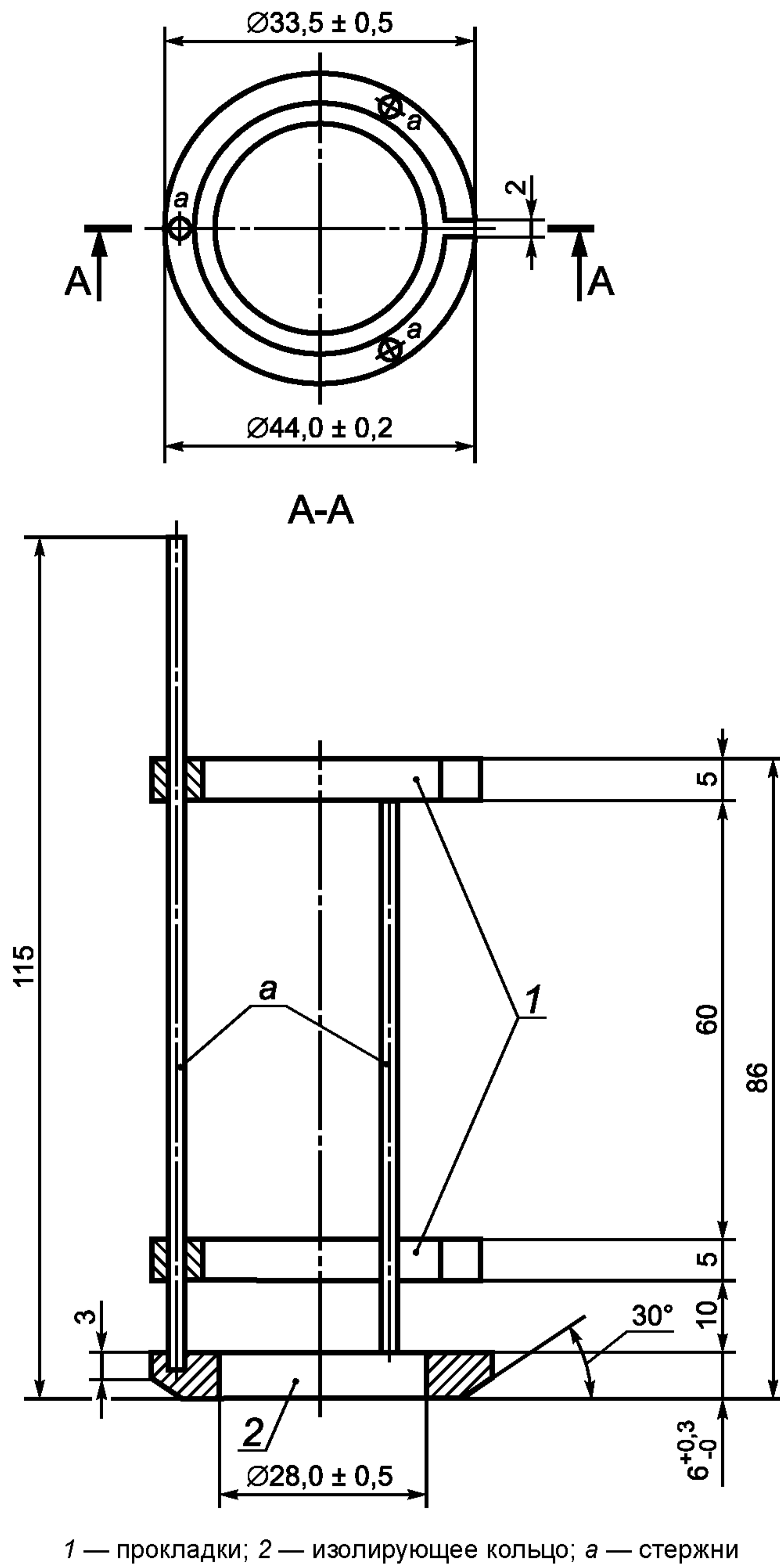
Рисунок 3 — Прокладки
