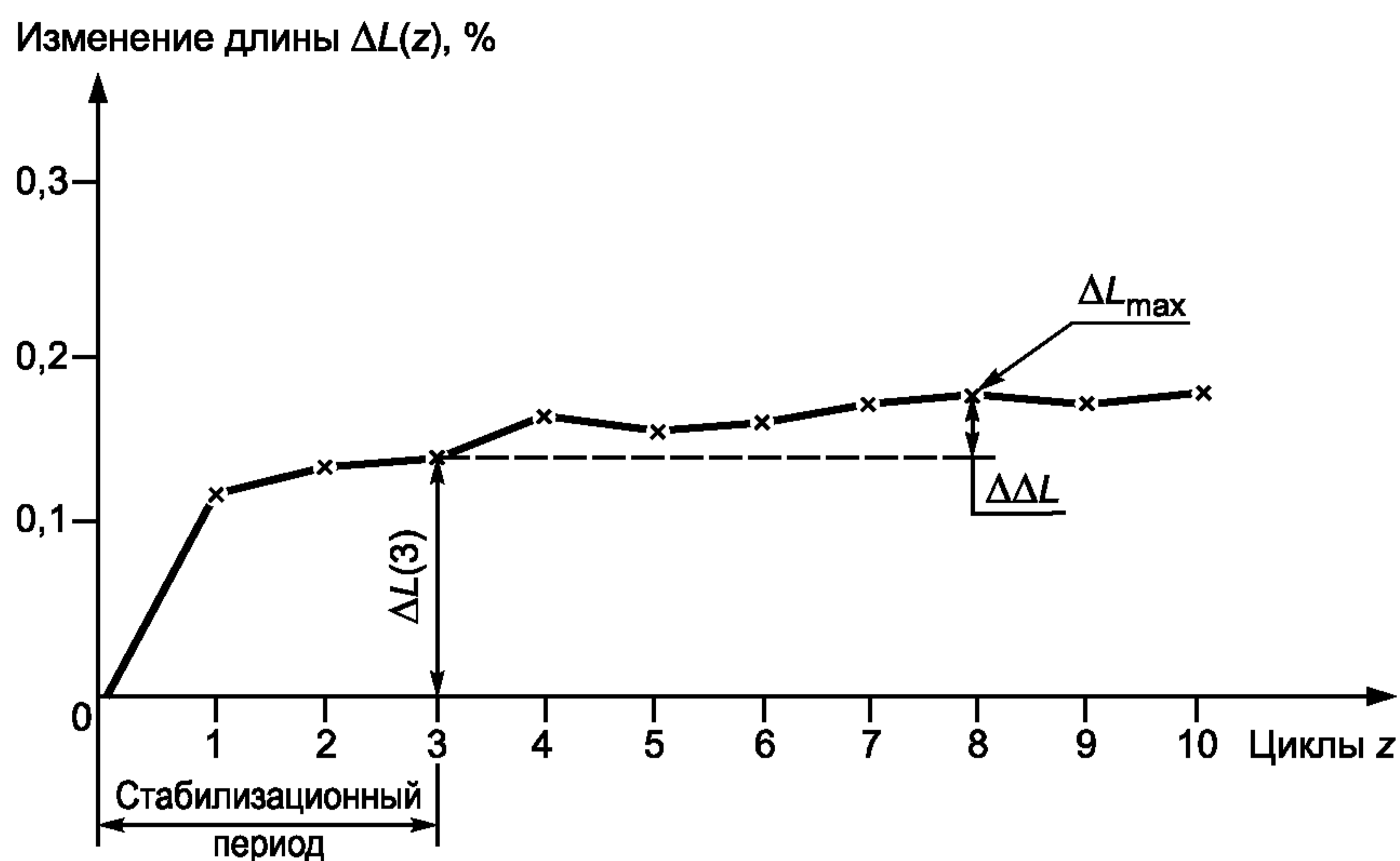
Рисунок 2 — Пример определения формоустойчивости образца
