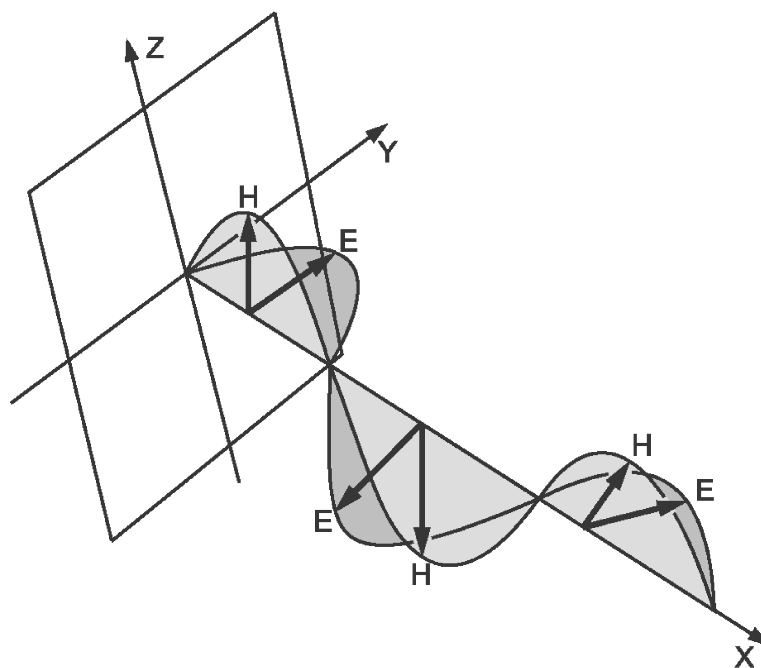
Рисунок 2 — Электромагнитное поле
