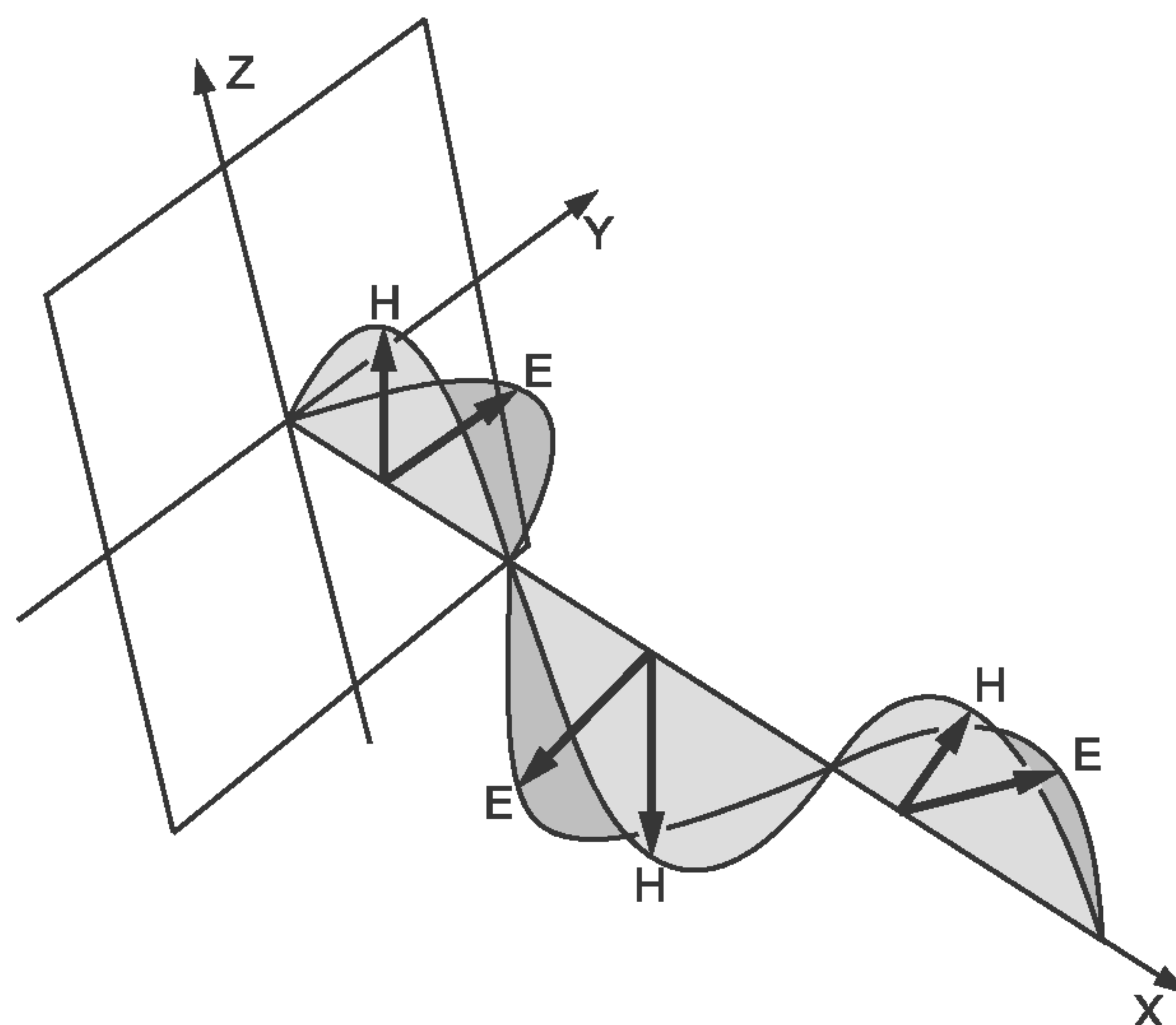
Рисунок 1 — Электромагнитное поле
