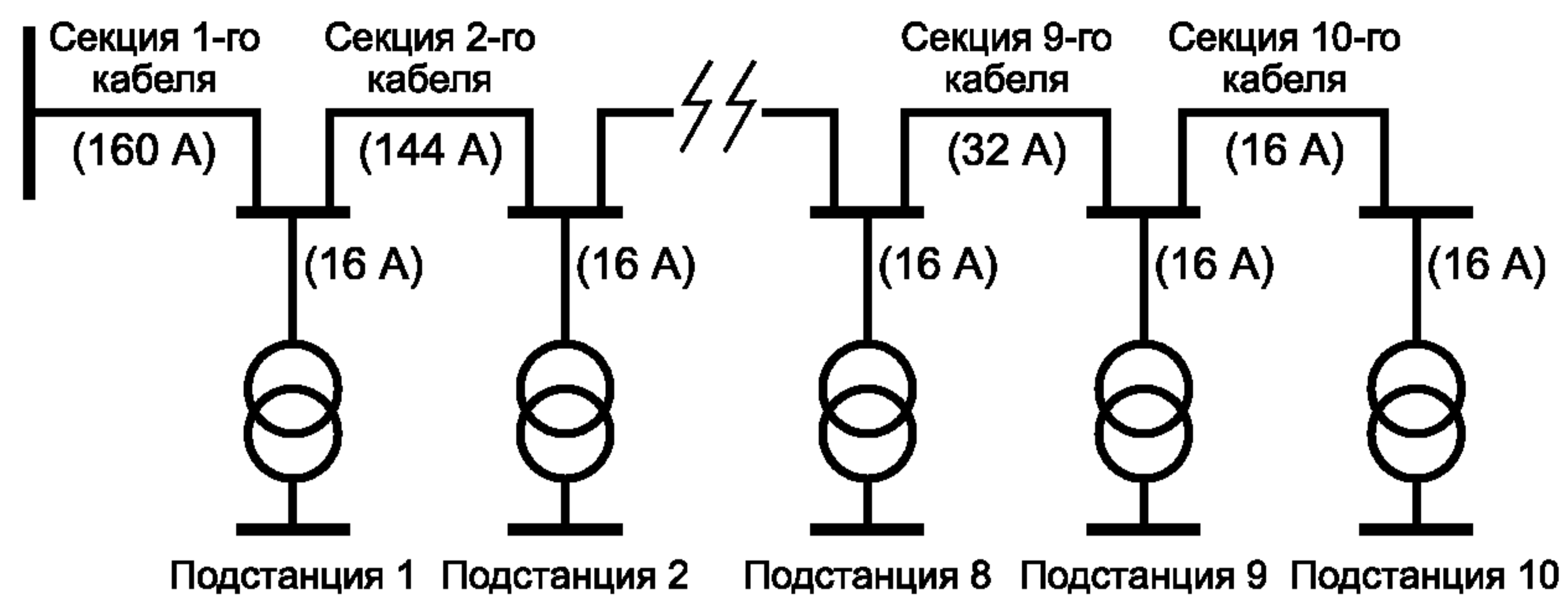
Рисунок А.1 — Схема кабельной системы
