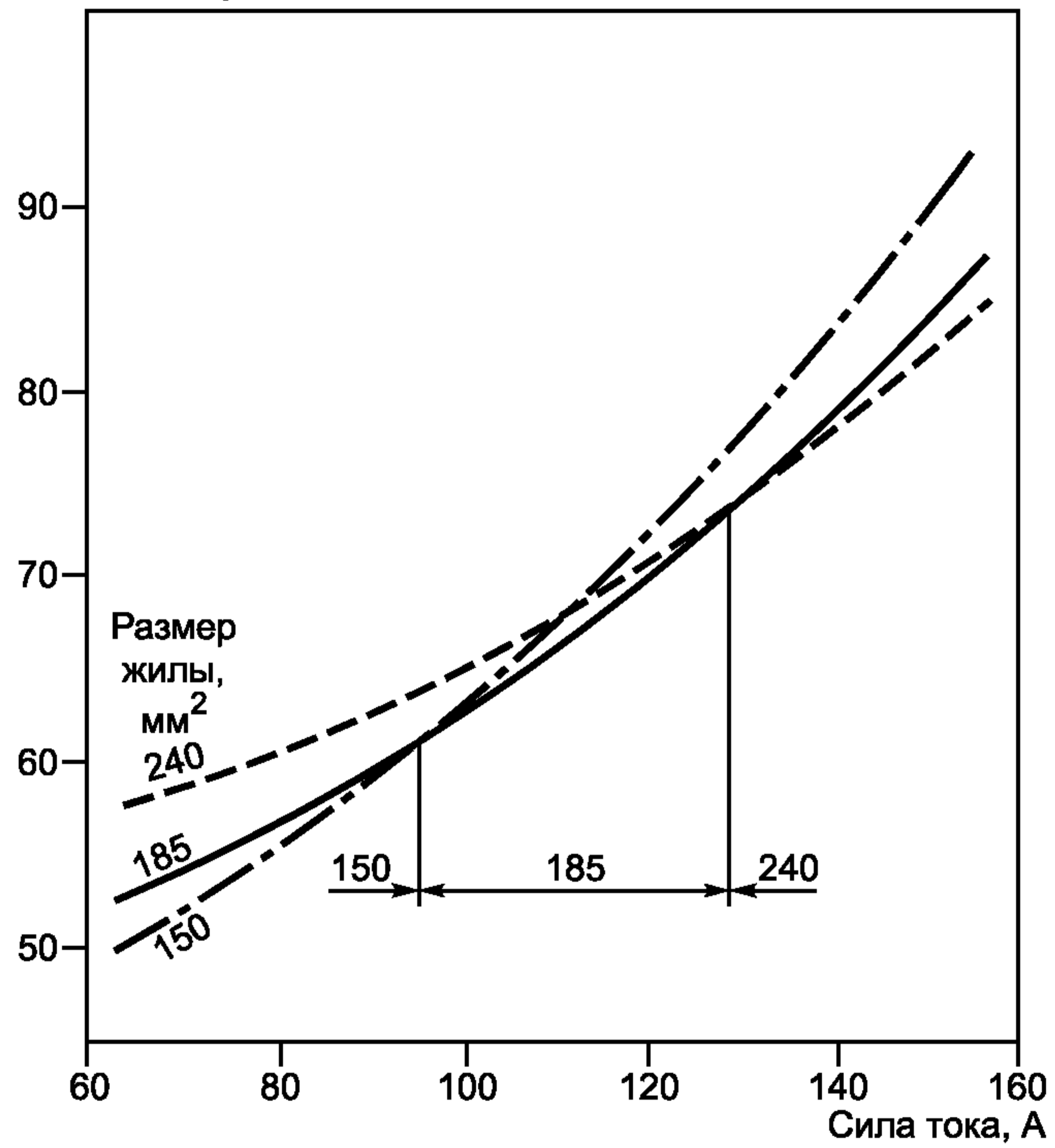
Рисунок А.2 — Диапазоны экономичных токов
