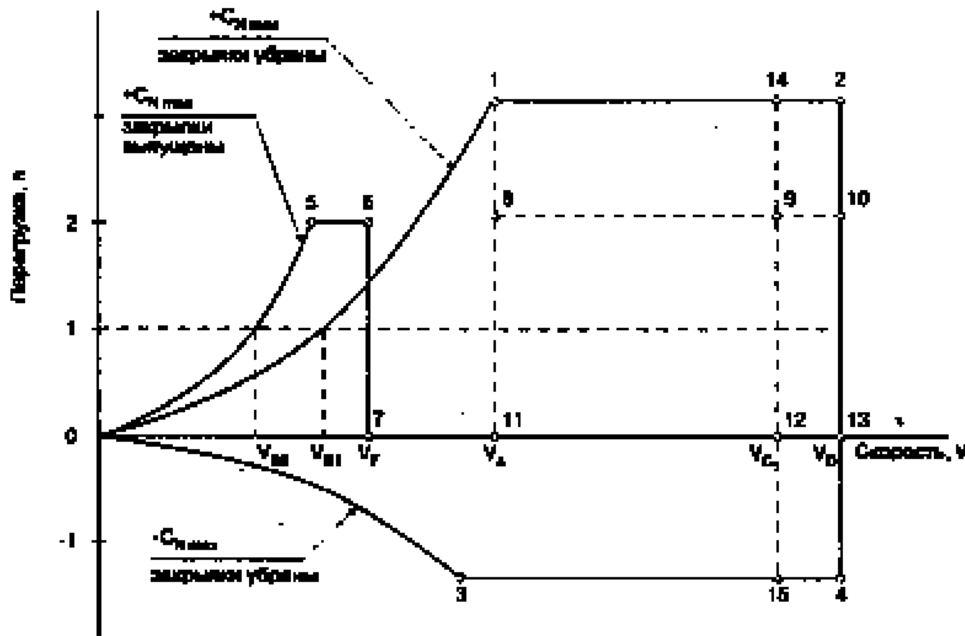
Огибающая перегрузок при полете в неспокойном воздухе
