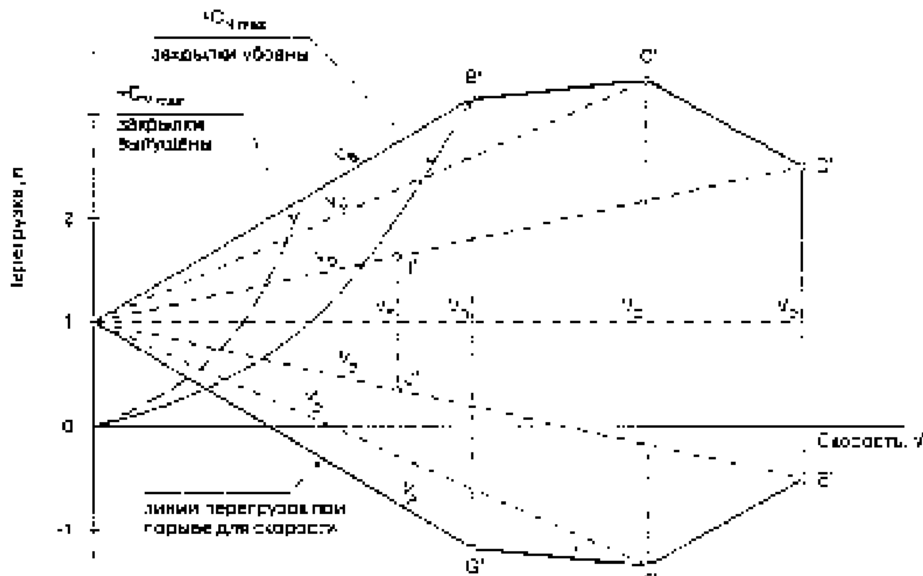
Огибающая перегрузок при полете в неспокойном воздухе
