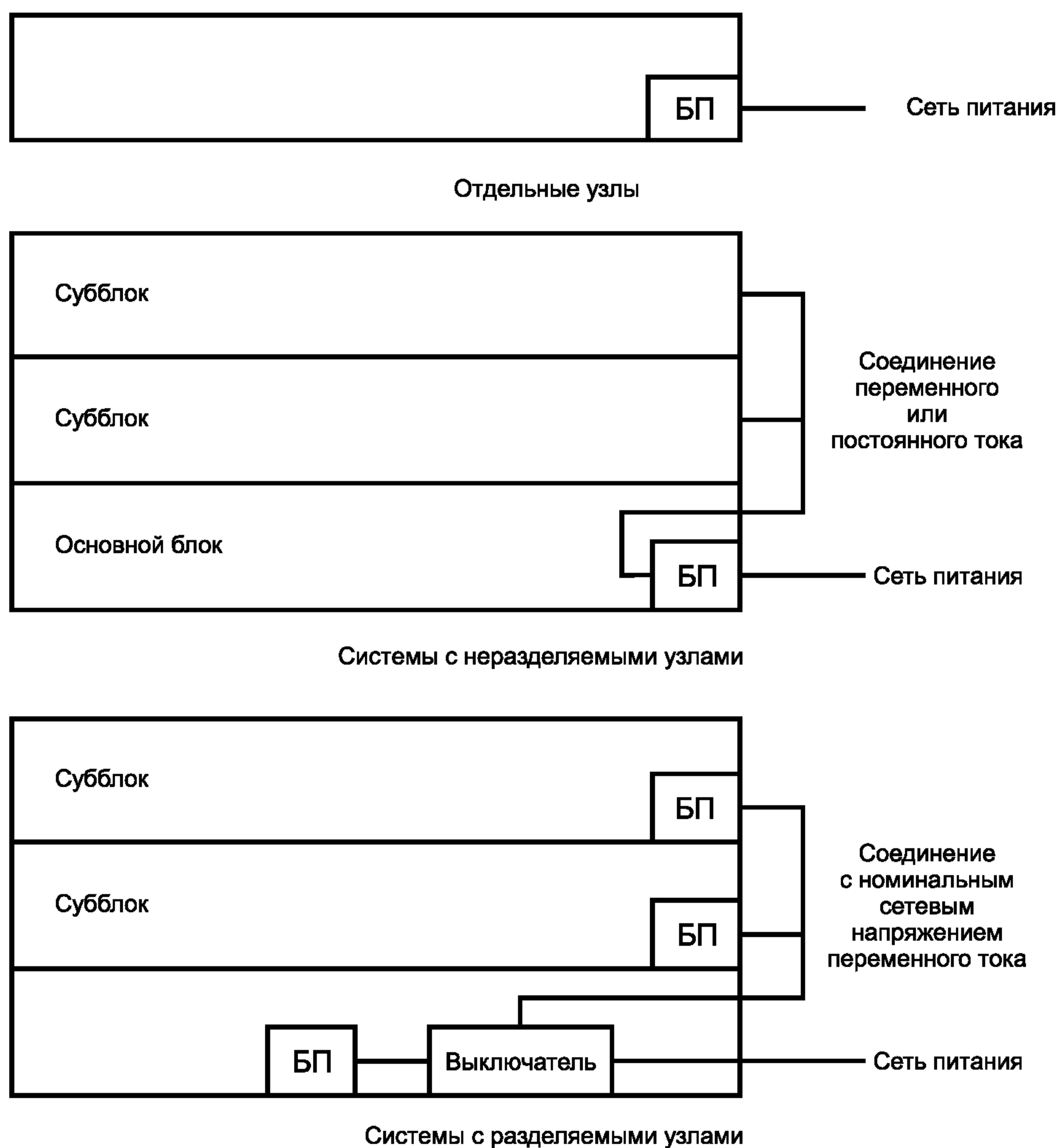
Рисунок 2 — Возможные конфигурации аудиооборудования
