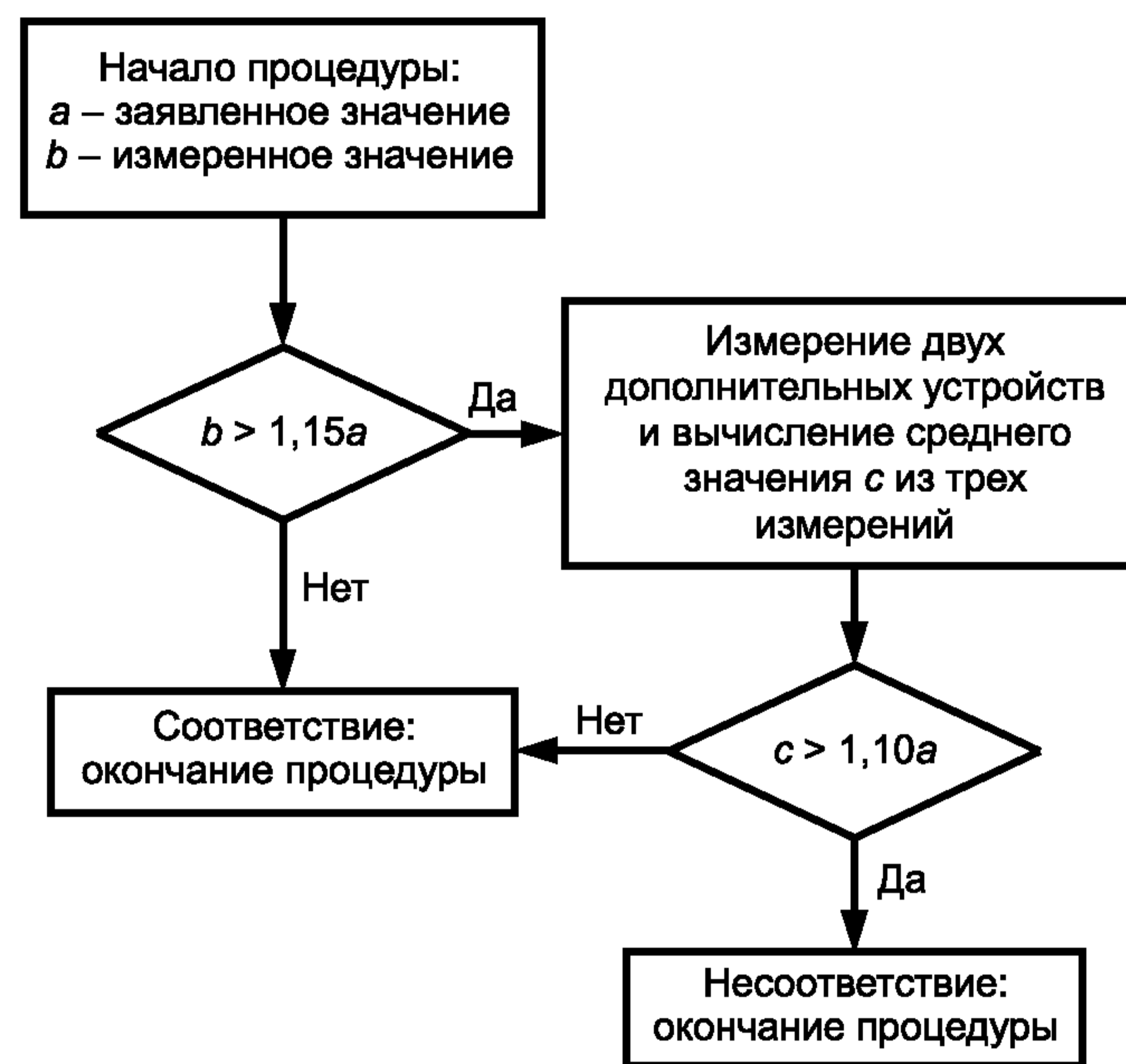
Рисунок А.1 — Схема процедуры проверки
