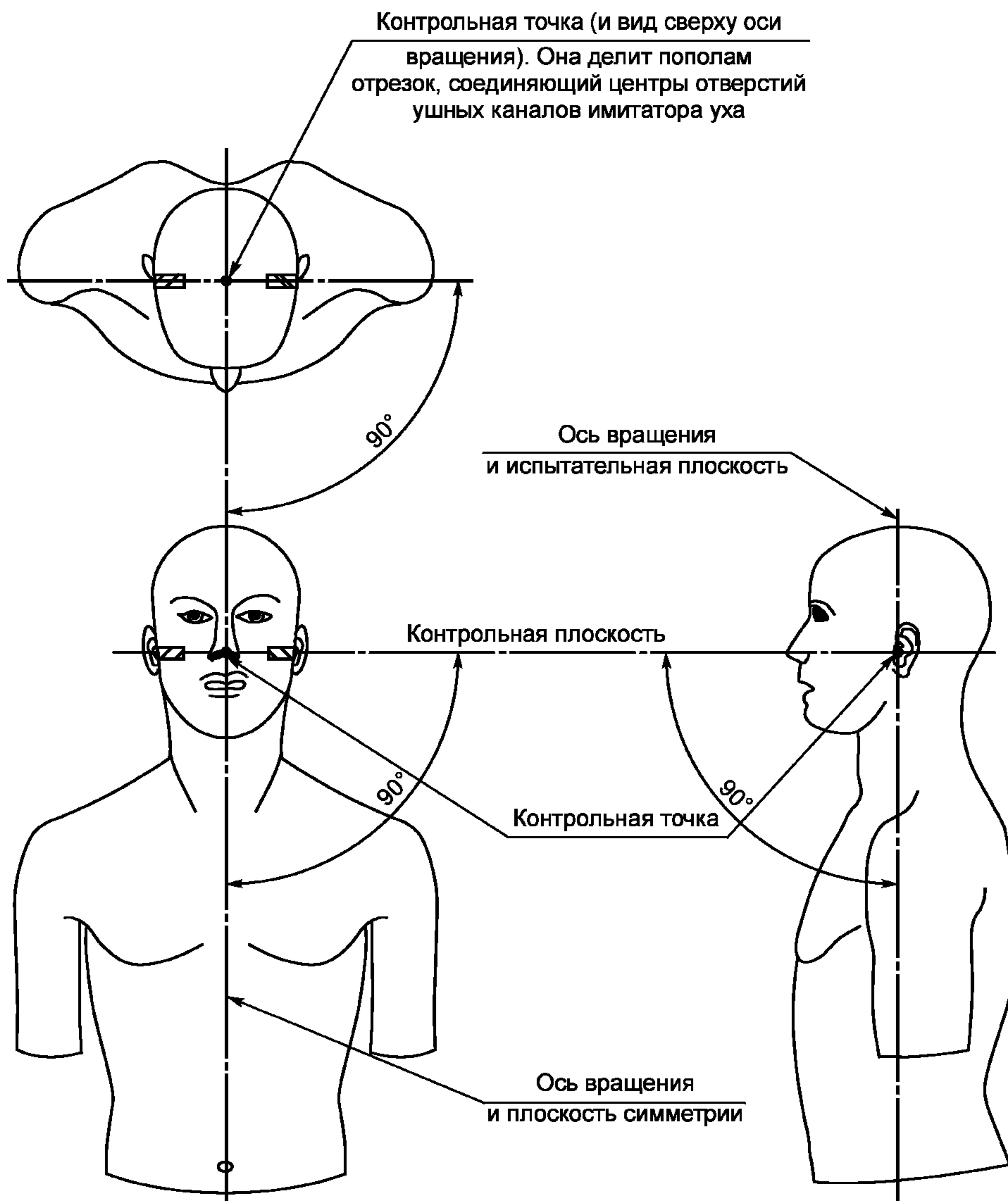
Рисунок С.1 — Геометрические характеристики манекена
