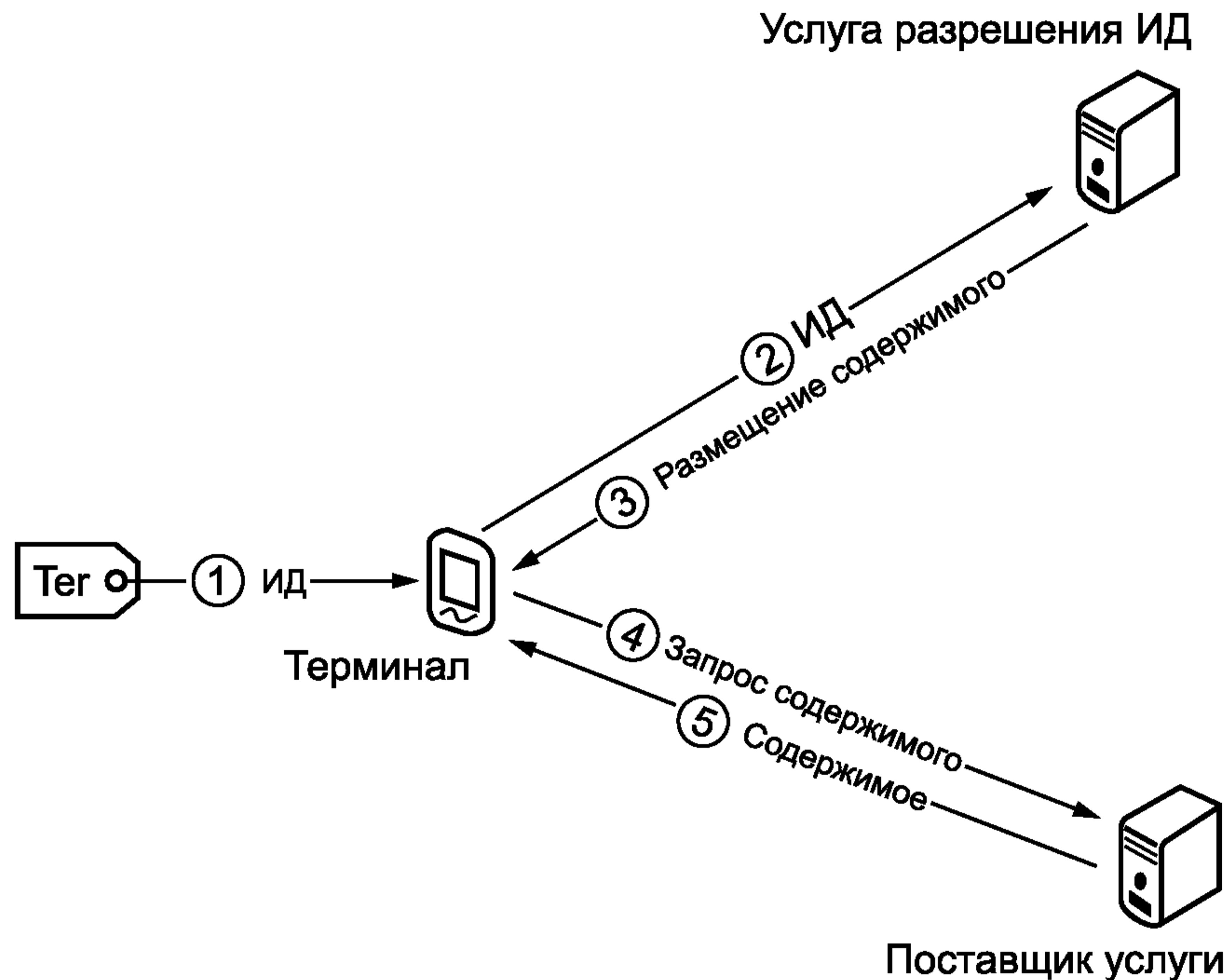
Рисунок 1 — Работа основанных на тегах приложений и услуг
