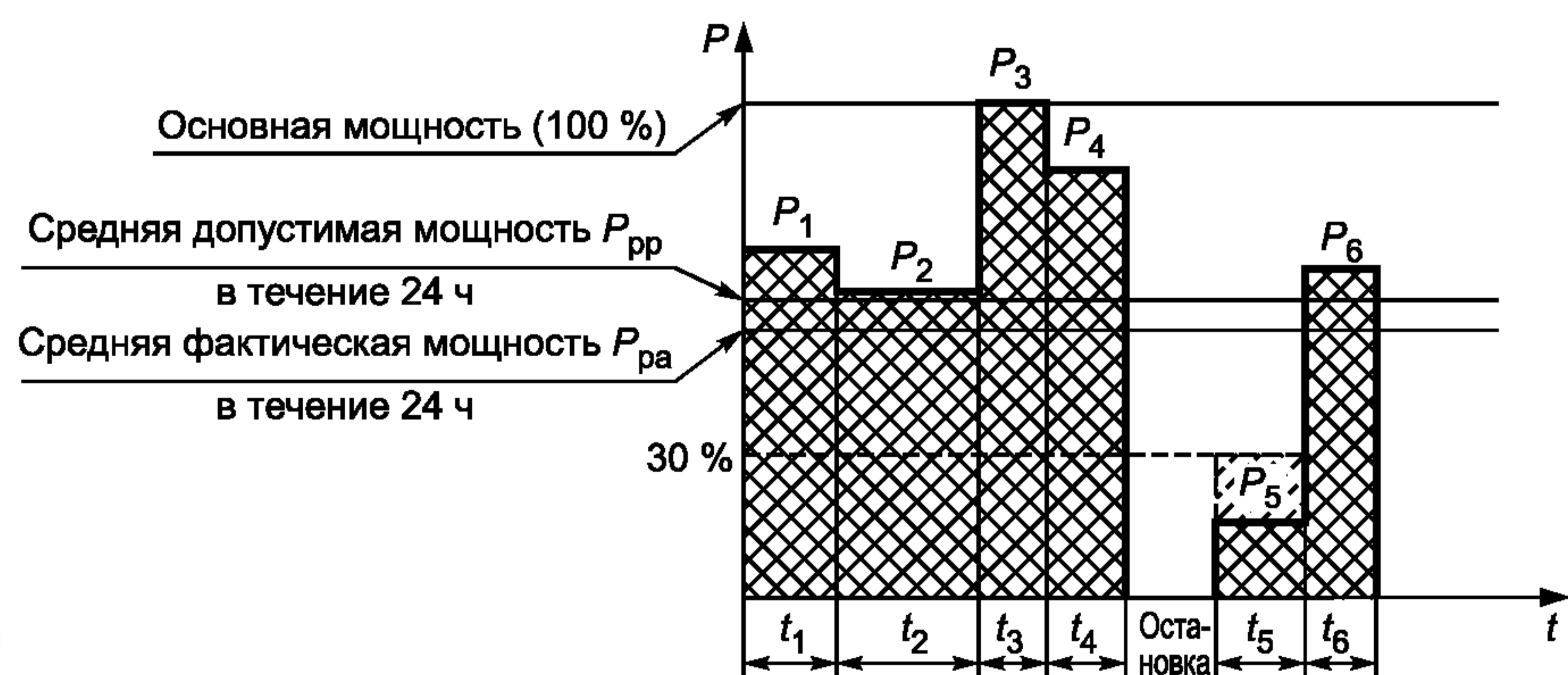
Рисунок 2 — График-иллюстрация основной мощности (PRP)
