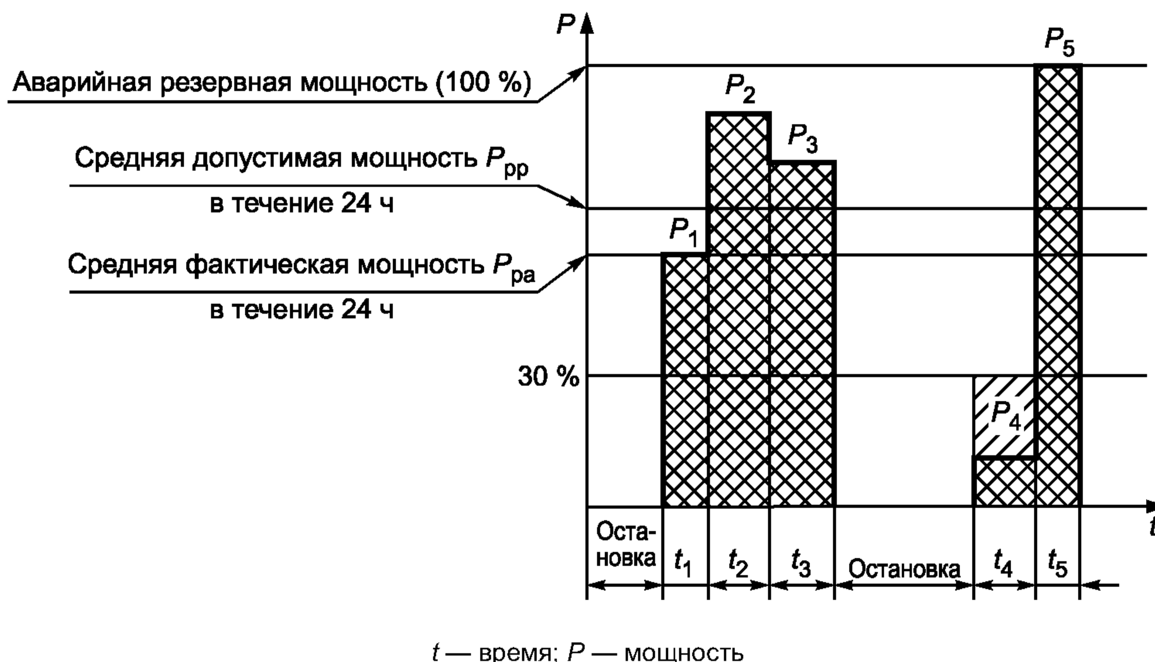
Рисунок 4 — График-иллюстрация аварийной резервной мощности (ESP)
