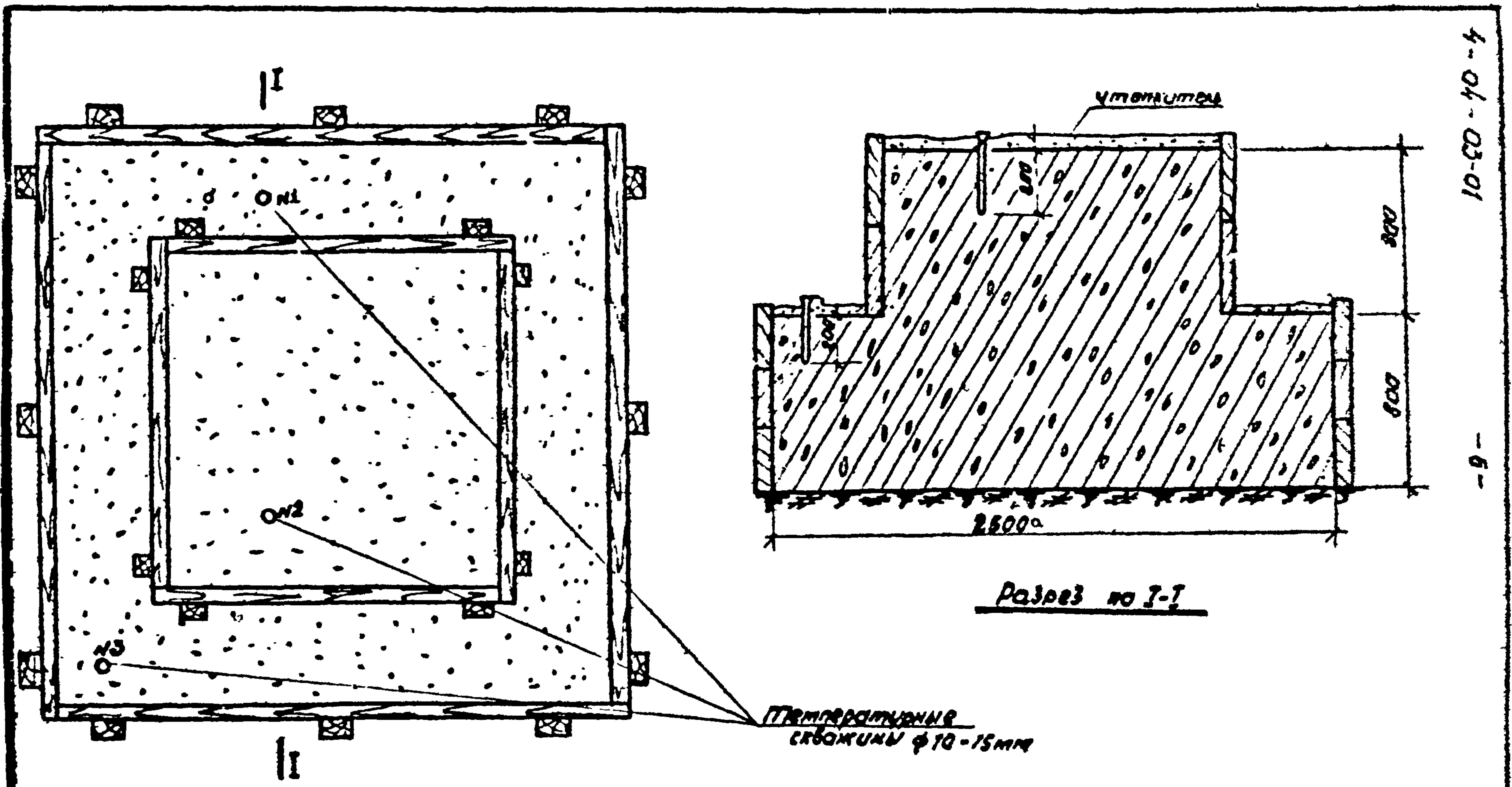
Рис.2 Расположение и нумерация температурных стержней при электропрогреве монолитных фундаментов
