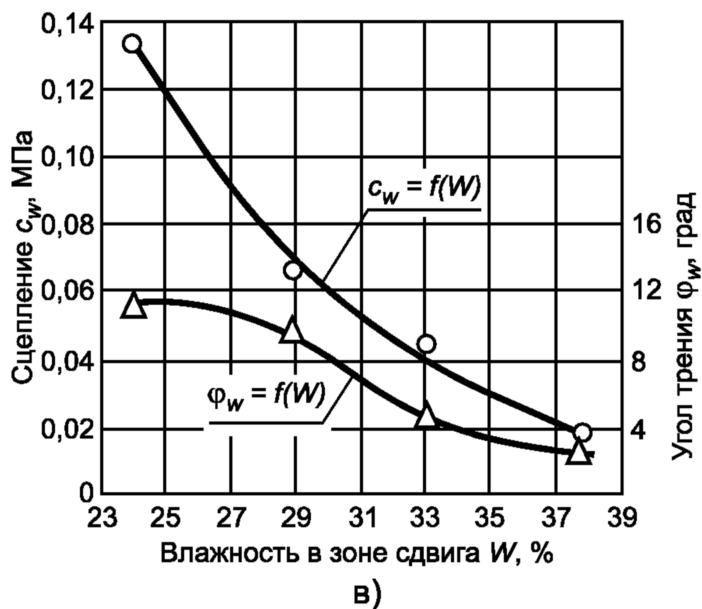
Рисунок 1 — Пример обработки результатов сдвиговых испытаний
