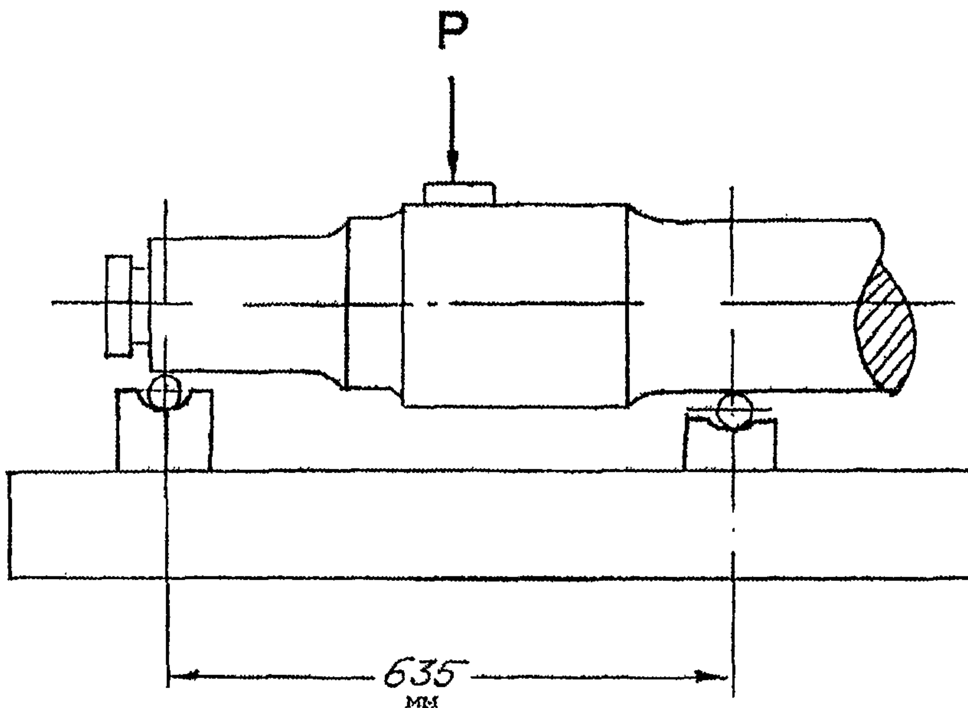
Рисунок 1 – Схема проведения испытаний
