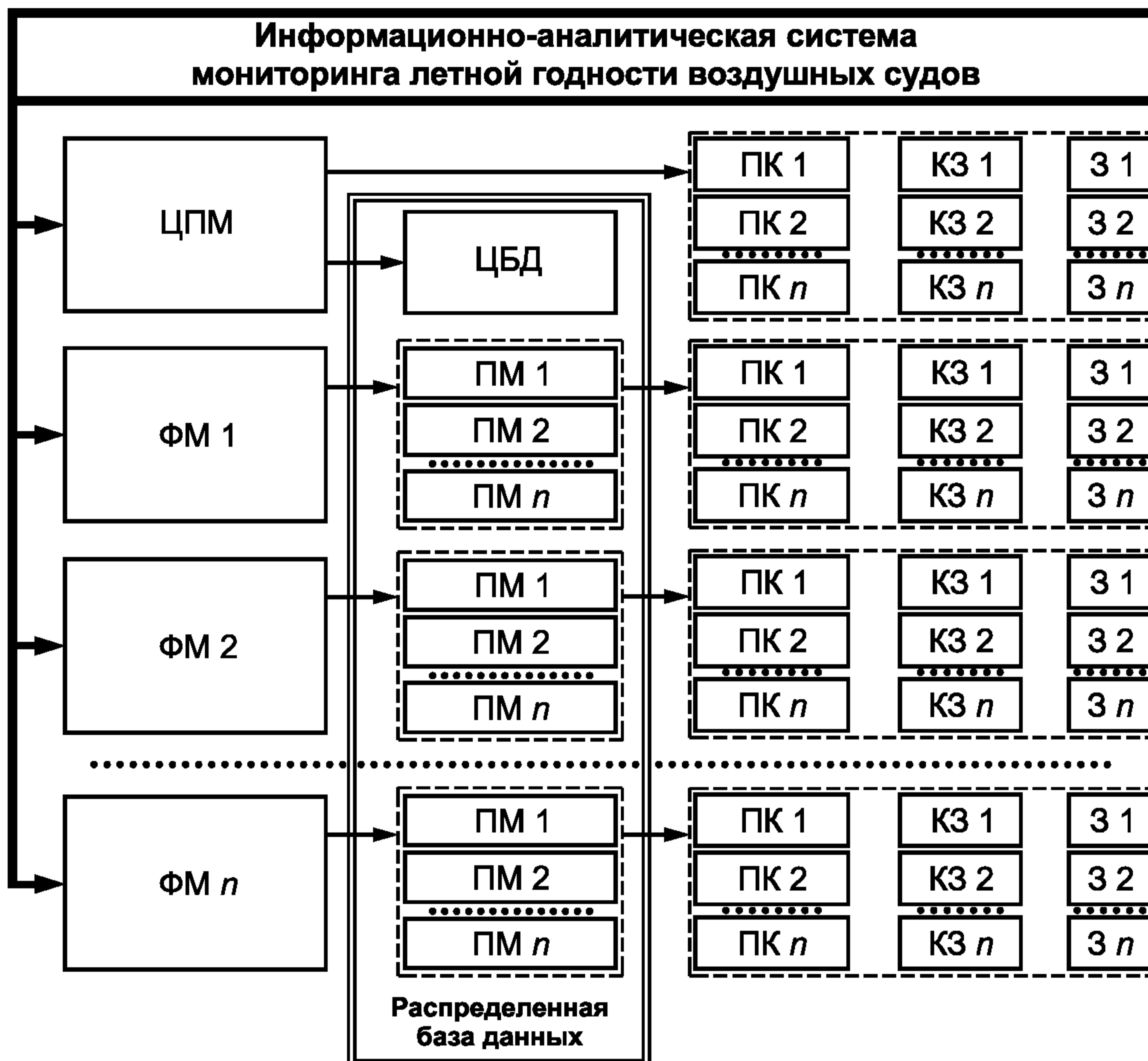
Рисунок 1 — Схема функциональной архитектуры ИАС МЛГ ВС
