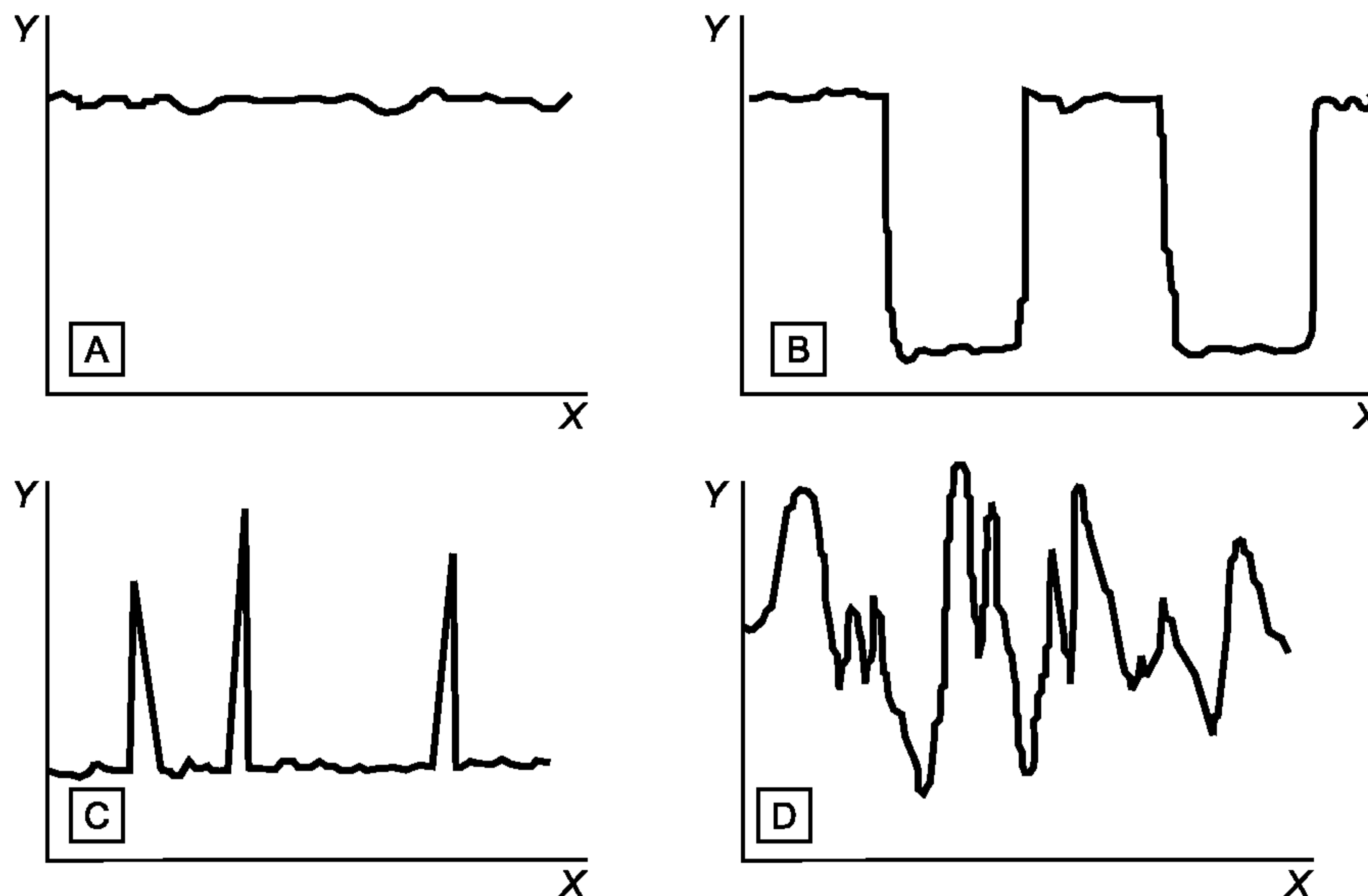
Рисунок 3 — Примеры того, как выбросы могут изменяться со временем
