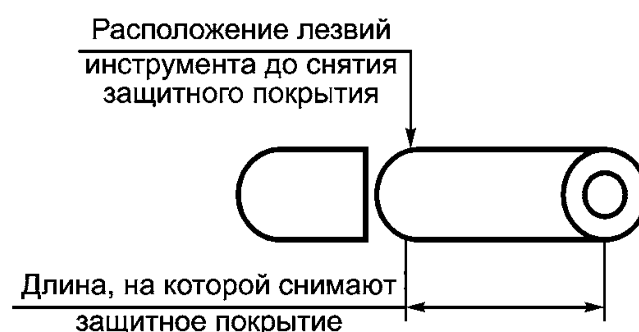
Рисунок 1 — Длина волокна, на которой снимают защитное покрытие
