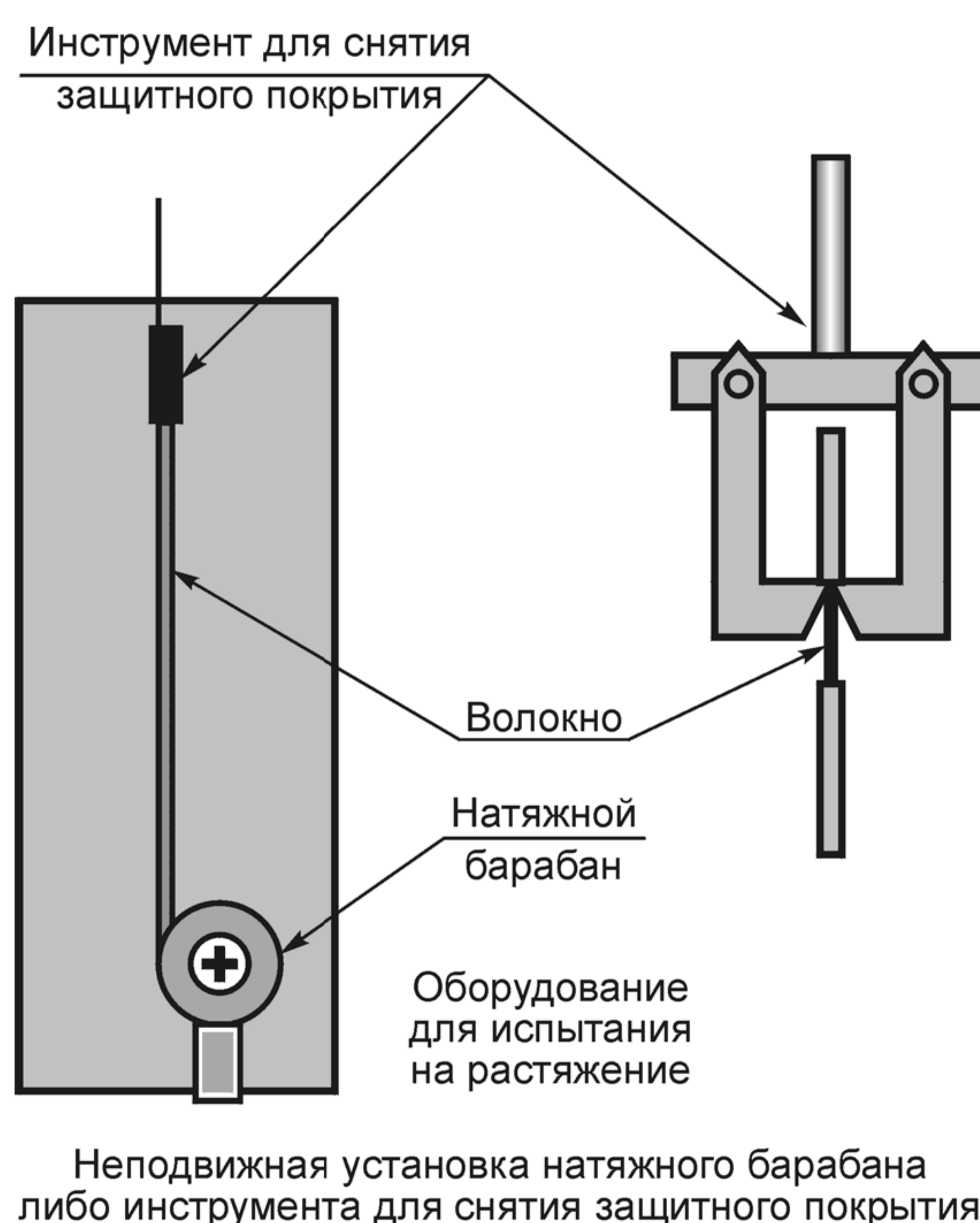
Рисунок 2 — Пример испытательного устройства
