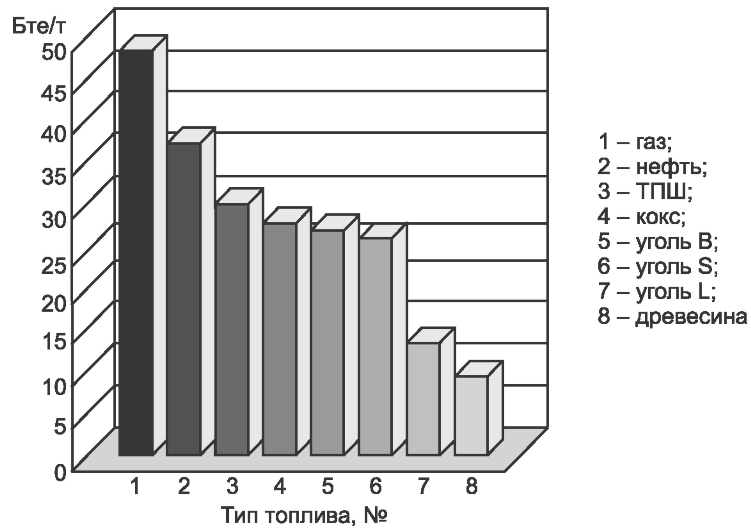
Рисунок 1 — Сравнение относительной энергии различных типов топлива
